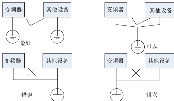
图 4-19 接地示意图
