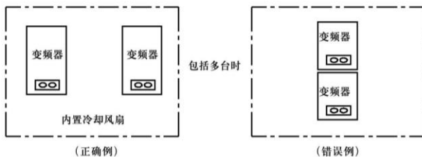
图 1-3 变频器安装在控制柜内示意图
