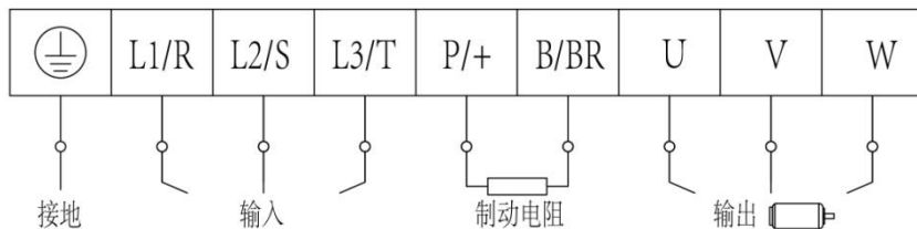
图 4-4 端子示意图
