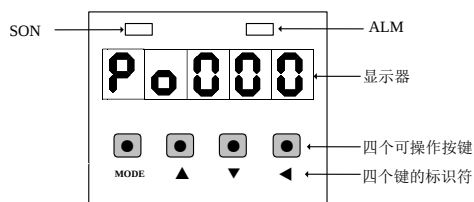
图 5.1.1 操作面板示意图
