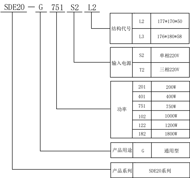
图 2. 1. 1 伺服驱动器命名规则
