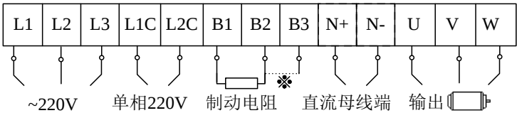
图 4.1.2 220V 伺服功率端子接线示意图
