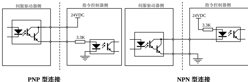
图 4.3.16 光电耦合器输出接口电路
