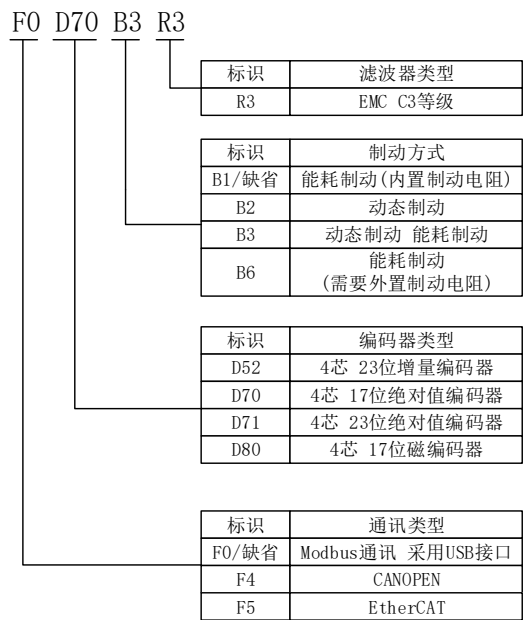
图 2.1.2 伺服驱动器功能部分命名规则
