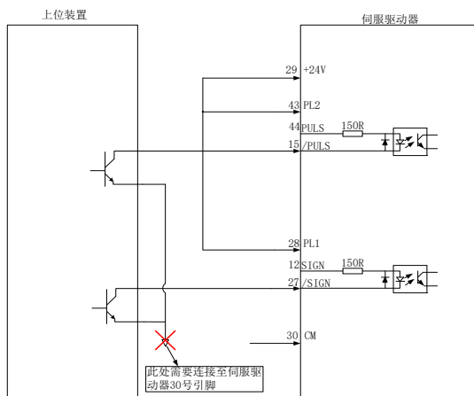
图 4.3.8 24V 集电极开路接线错误示意图 3
