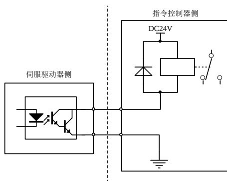
图 4.3.14 继电器输出接口正确电路示意图
