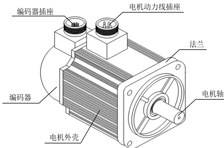
图 2.2.4 伺服电机各部分名称
