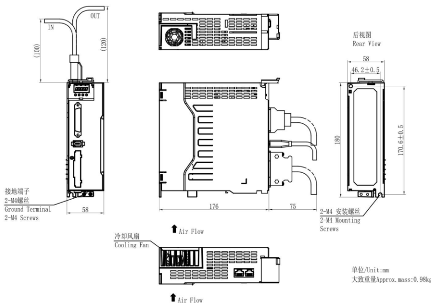
图 3.1.2 伺服驱动器结构尺寸 2
