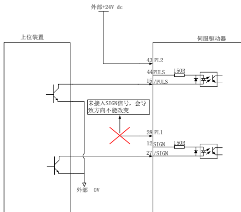
图 4.3.7 24V 集电极开路接线错误示意图 2
