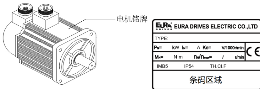
图 2.2.2 伺服电机铭牌示意图（180 及以下法兰伺服电机）
