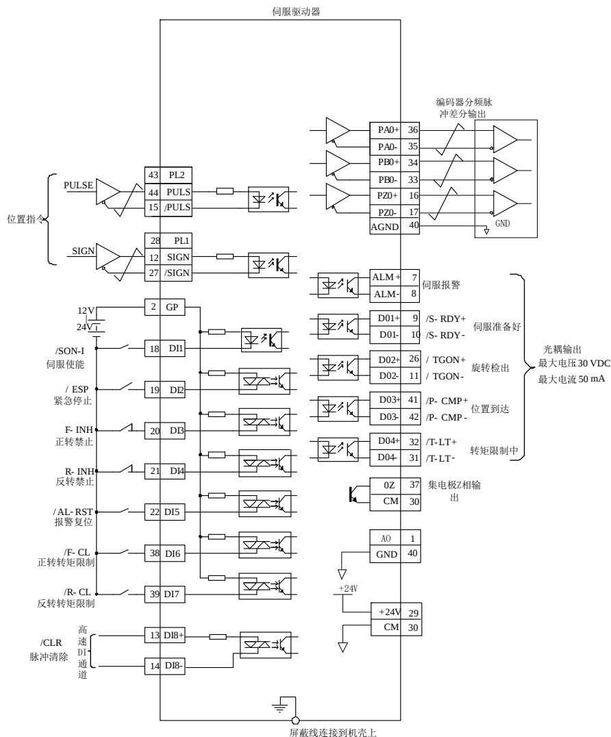
图 6.4.2 外部位置脉冲模式典型接线图
