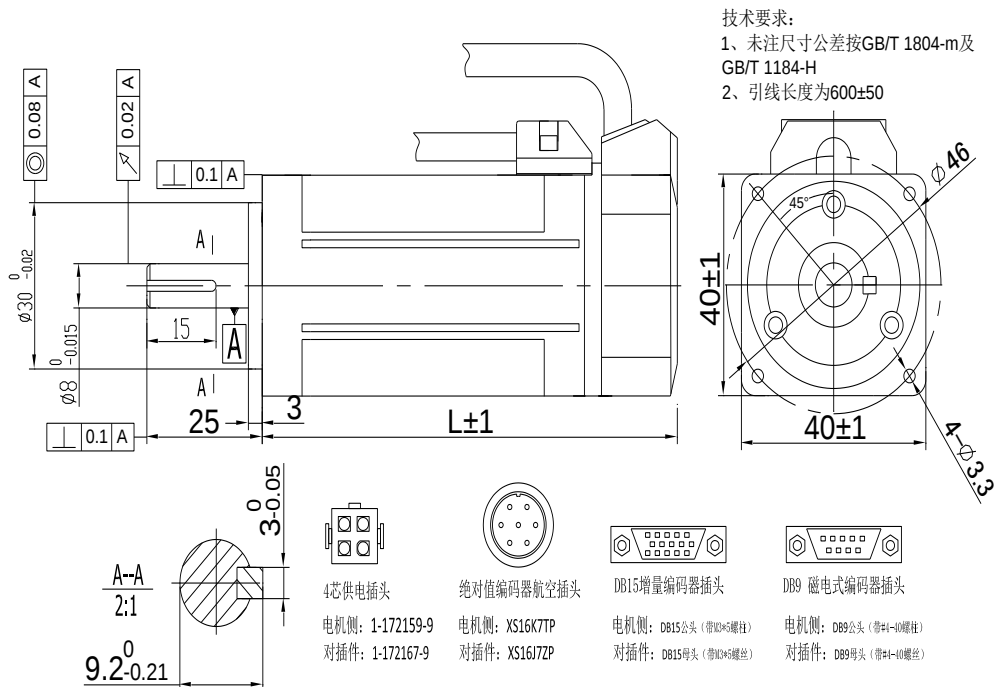
40 法兰电机外形尺寸图
