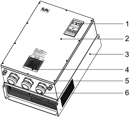
图 1-3 产品外形及结构部件图
