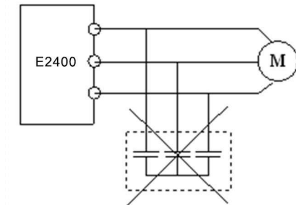
图 1-6 变频器输出端禁止使用电容器
