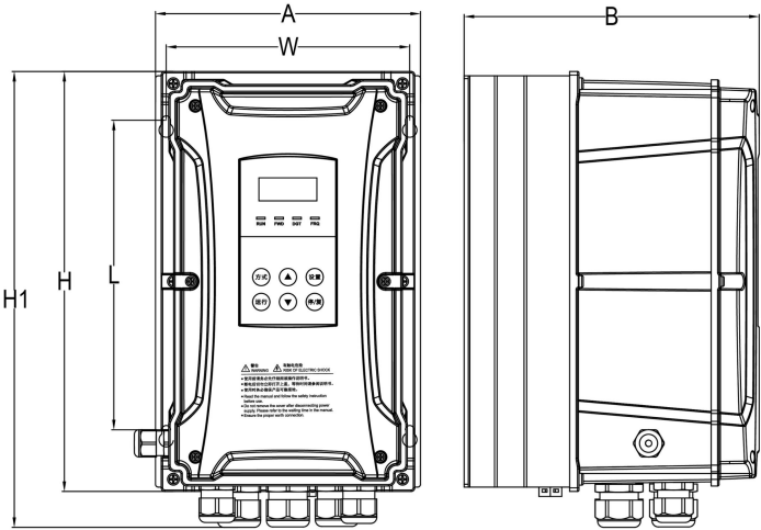
图 7-1 塑壳壁挂外形
