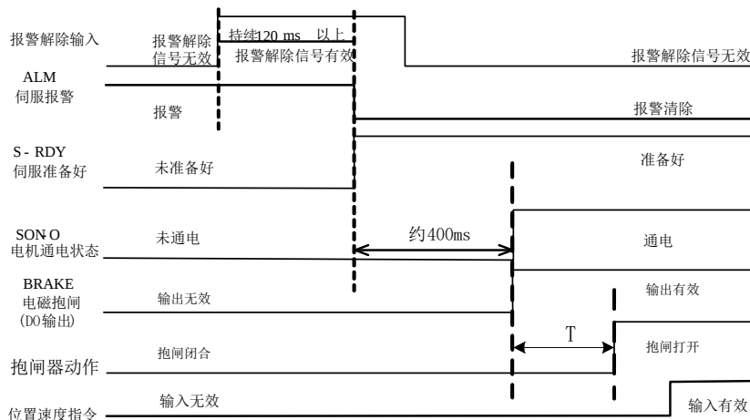
图 7.1.8 报警复位时序
