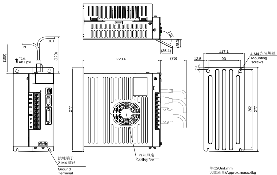
图 3.1.7 伺服驱动器结构尺寸 5
