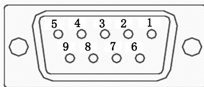
图 4.2.2 旋转变压器编码器端子排列示意图
