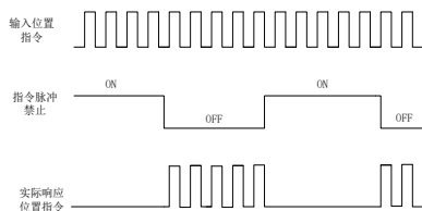
图 7.2.4 位置指令禁止时序图
