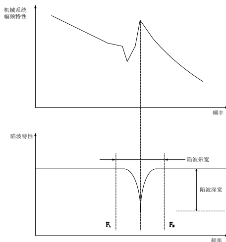
图 9.4.1 陷波器的抑制原理
