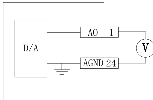
图 4.3.12 模拟量监控输出接口
