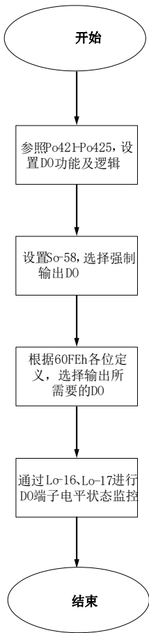
图 7.3.3 DO 信号强制输入设定步骤示意图
