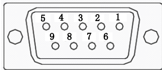
图 4.2.5 Biss-C 型编码器端子排列示意图
