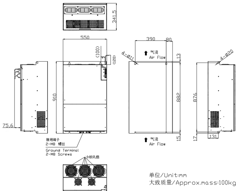
图 3. 1. 13 伺服驱动器结构尺寸 12
