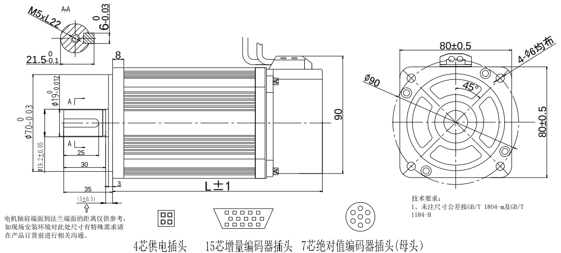
80 法兰伺服电机外形尺寸图
