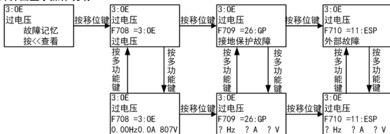
图 5-6 故障界面操作流程图中
