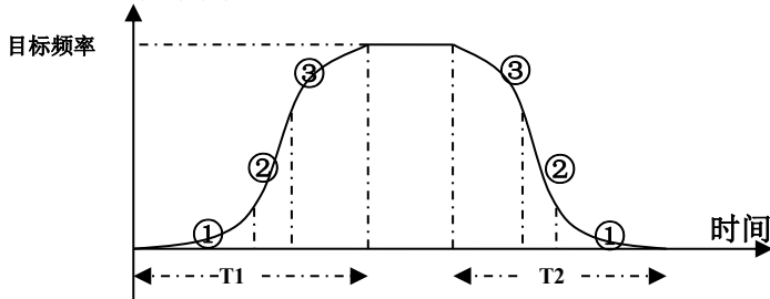
图 6-9 S 曲线加减速示意图
