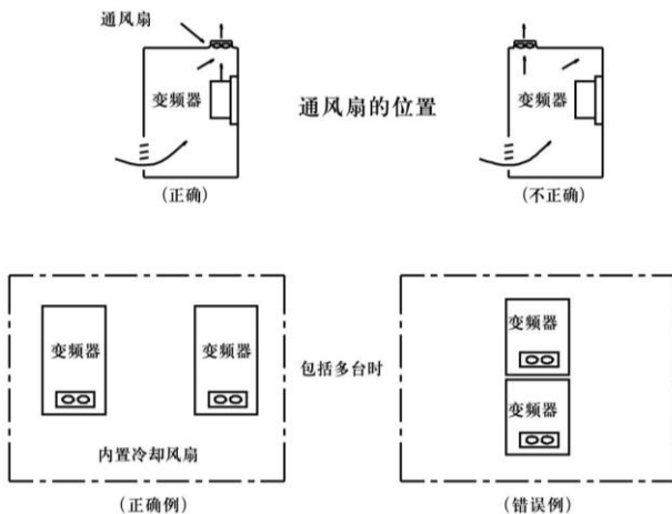
图 1-3 变频器安装在控制柜内示意图
