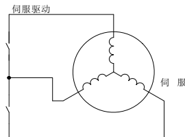
图 7.1.9 动态制动的示意图
