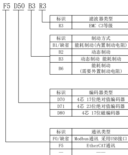
图 2.1.2 伺服驱动器功能部分命名规则
