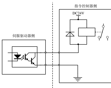
图 4.3.13 继电器输出接口正确电路示意图
