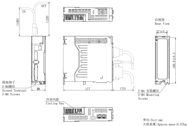
图 3.1.1 伺服驱动器结构尺寸 1
