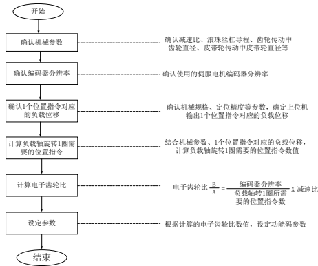
图 7.1.12 电子齿轮比设置步骤流程图
