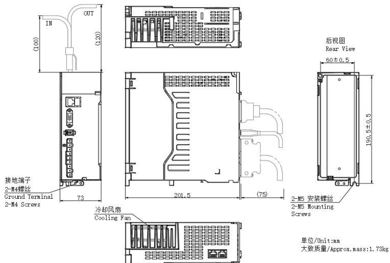
图 3.1.3 伺服驱动器结构尺寸 3
