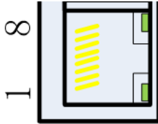
图 4.3.17 L2 结构通讯插头端子排列顺序图
