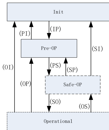
图 6.1.4 EtherCAT 状态机
