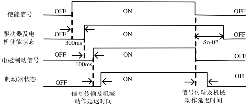
图 7.1.3 电磁抱闸制动时序图
