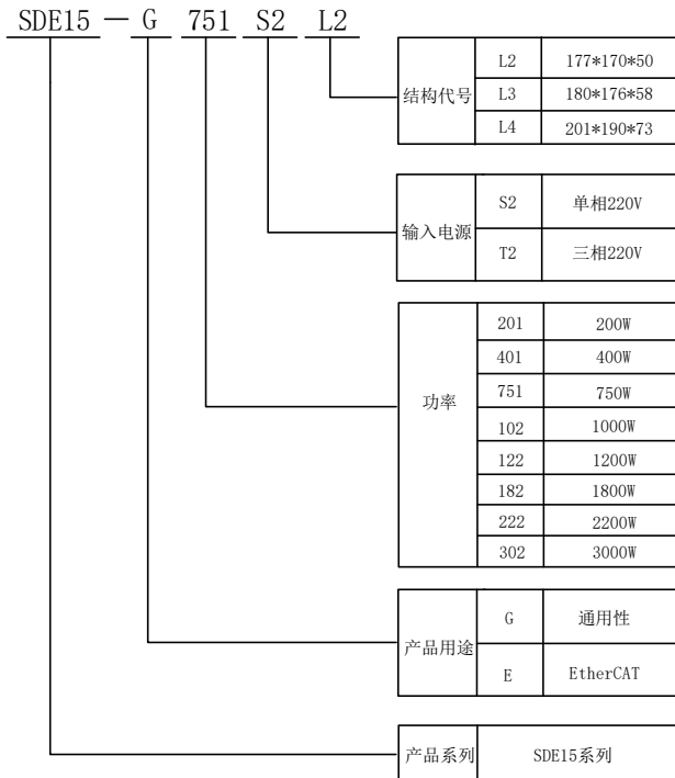
图 2.1.1 伺服驱动器命名规则
