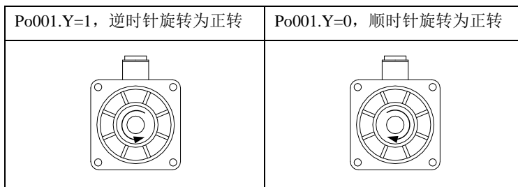
图 7.1.1 电机旋转方向示意图
