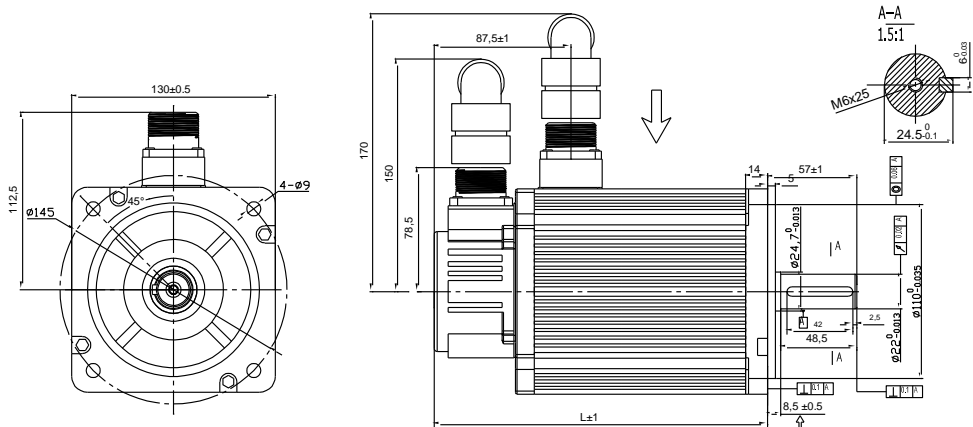
130 法兰伺服电机外形尺寸图
