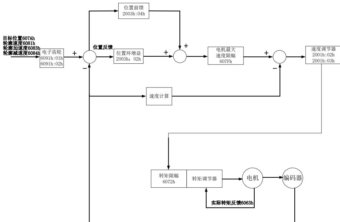
图 7.3.1 轮廓位置模式（PP）控制框图
