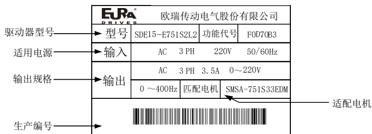
图 2.1.2 伺服驱动器功能部分命名规则
