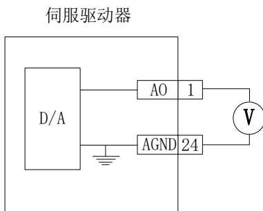
图 4.3.10 模拟量监控输出接口
