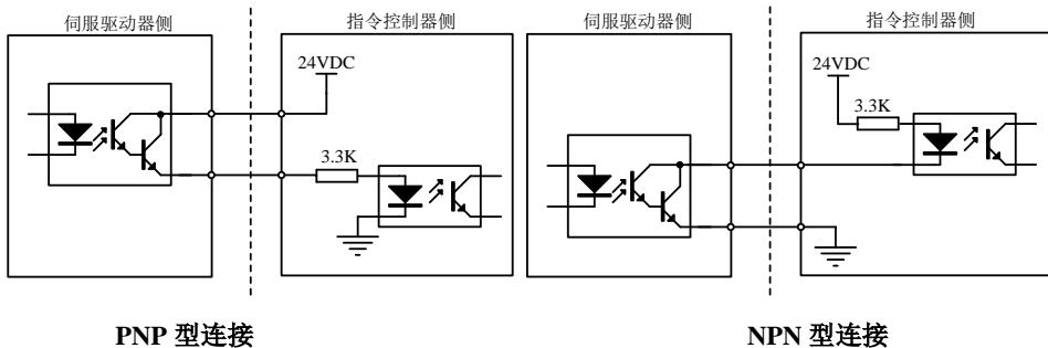
图 4.3.15 光电耦合器输出接口电路
