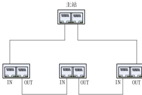
冗余环形连接：
