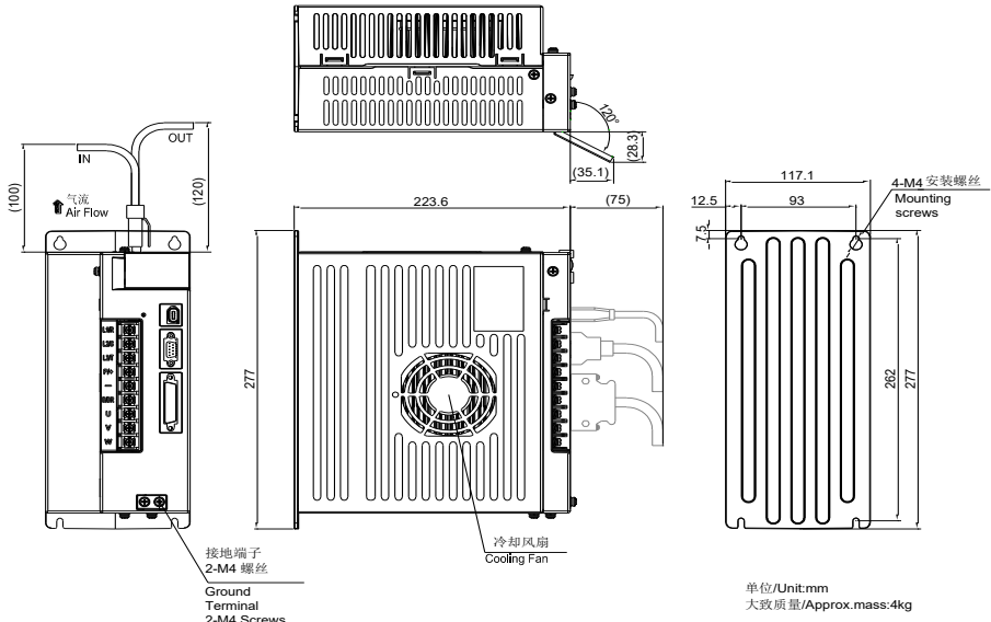
图 3.1.7 伺服驱动器结构尺寸 5
