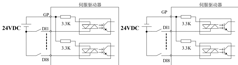
NPN 型接法
