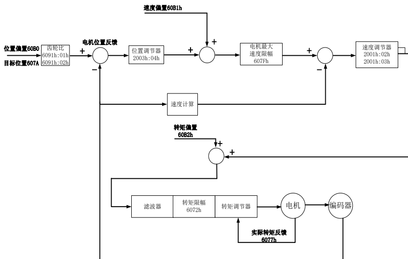
图 7.6.1 周期同步位置（CSP）控制框图
