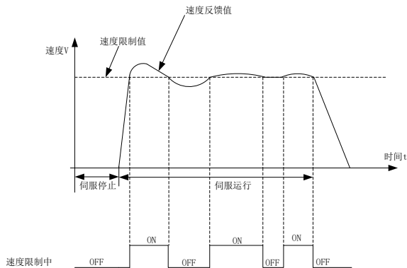
图 7.10.4 转矩模式下速度限制中输出示意图
