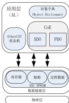
图 6.1.3 基于 CANOpen 应用层的 EtherCAT 通信结构
