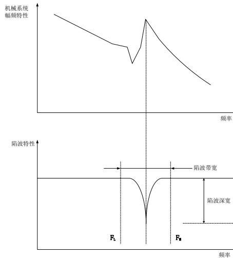
图 9.4.1 陷波器的抑制原理
