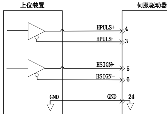
图 4.3.3 高速脉冲输入接口电路
