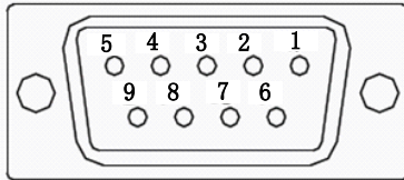
图 4.2.2 旋转变压器编码器端子排列示意图
