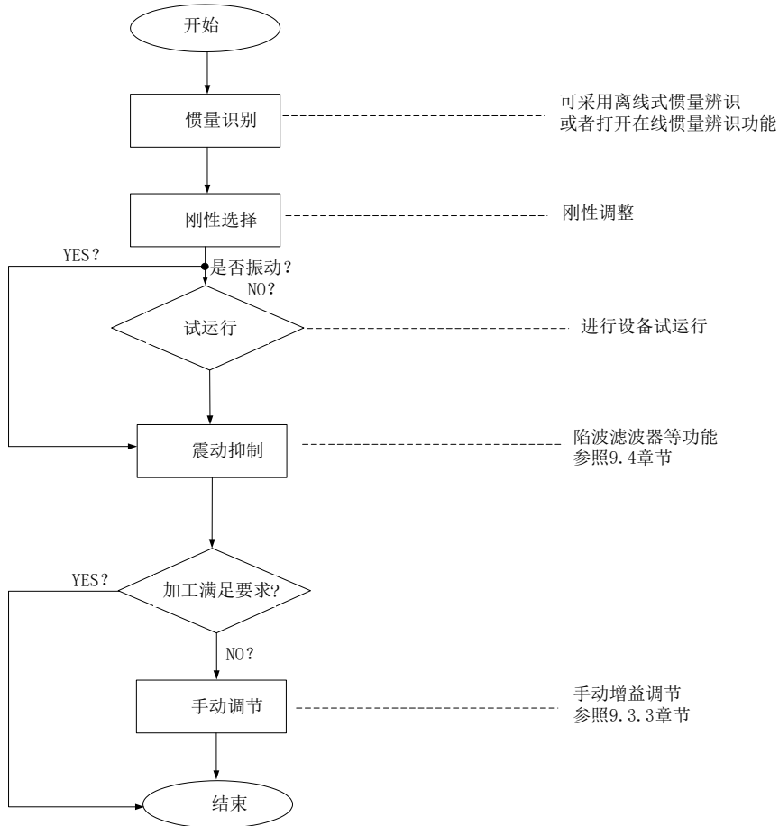
图 9.1.1 增益调节流程图
