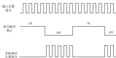
图 7.1.15 位置指令禁止时序图
