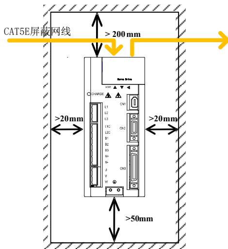
图 3.1.1 典型最小安装尺寸示意图
