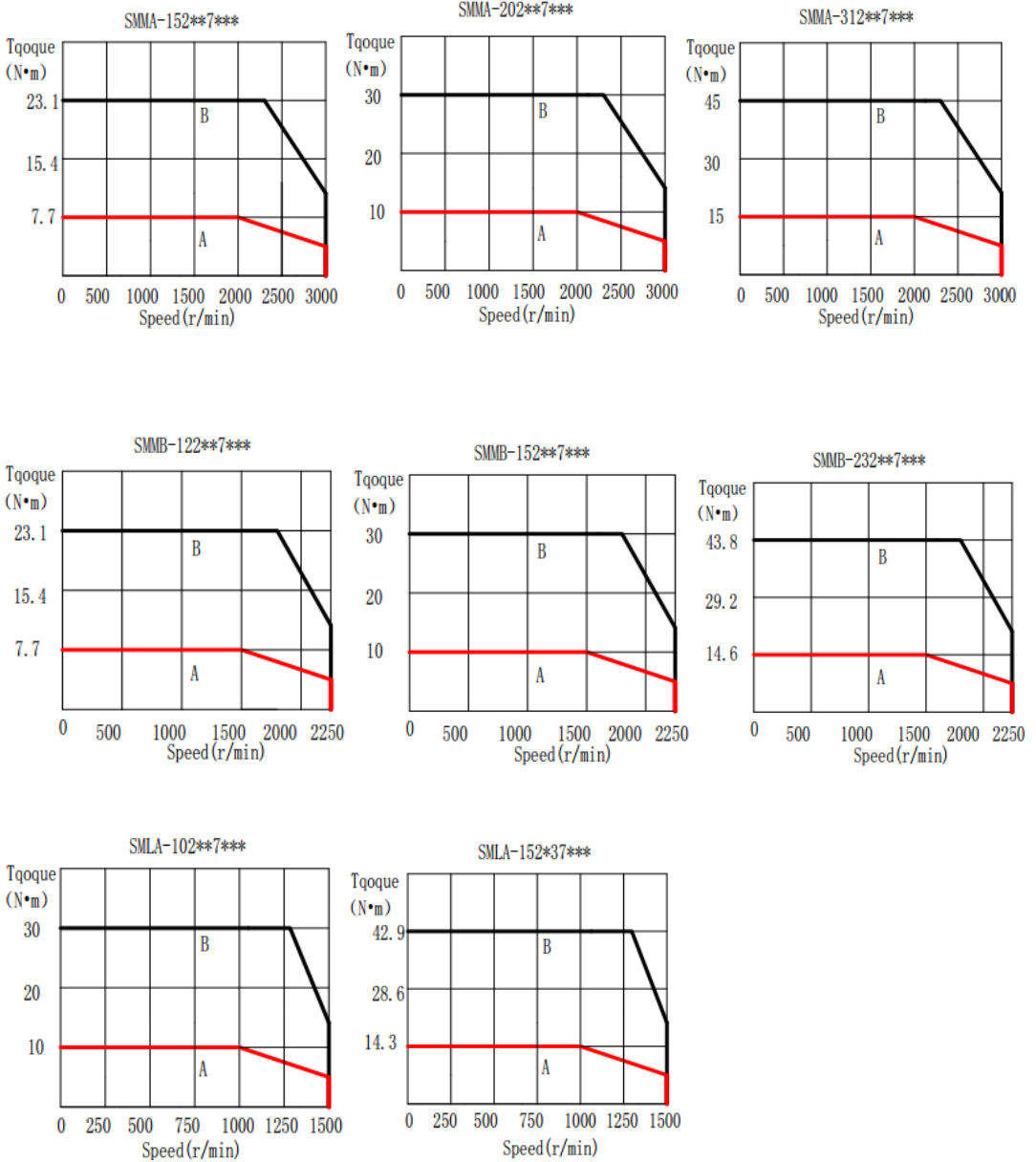
180 法兰伺服电机转矩-转速特性曲线
