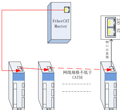
图 6. 1. 1EtherCAT 网络连接示意图
