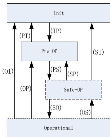
图 6.1.4 EtherCAT 状态机
