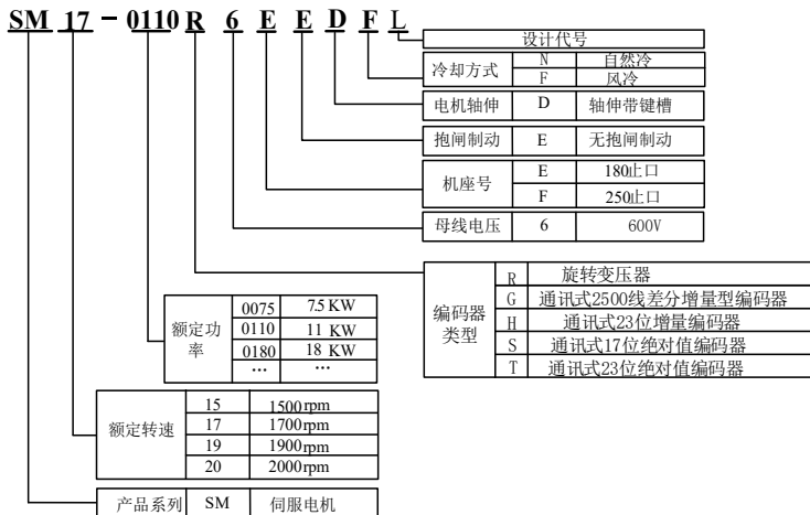
图 2.2.2 伺服电机命名规则（180 及 250 止口电机）
