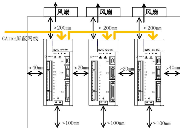
图 3.1.2 多台并列安装最小安装尺寸示意图
