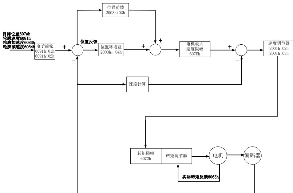
图 7.3.1 轮廓位置模式 (PP) 控制框图
