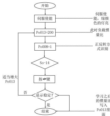
图 9.2.1 离线式转动惯量设置流程图
