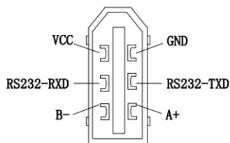
图 4.3.22 通讯口 CN1 插头端子排列顺序图
