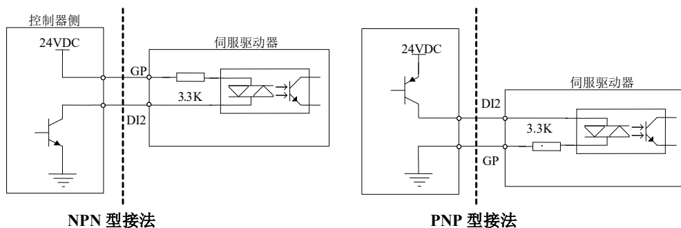
图 4.3.14 有源接点接口电路
