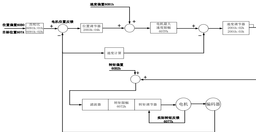
图 7.6.1 周期同步位置（CSP）控制框图
