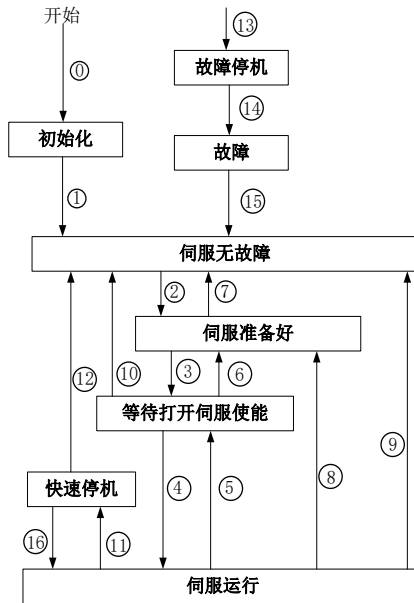
图 7.2.1 CiA402 状态机切换图
