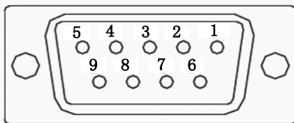
图 4.2.2 旋转变压器编码器端子排列示意图
