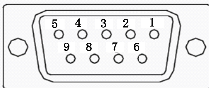
图 4.2.1 绝对值型编码器端子排列示意图
