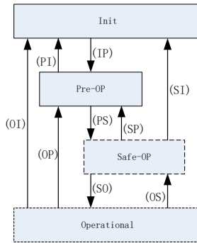
图 6.3.2 EtherCAT 状态机
