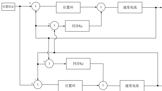
图 6. 4. 41 龙门同步典型应用接线图
