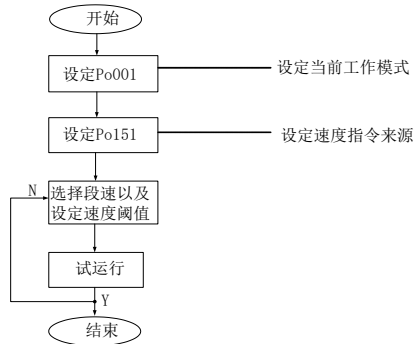
图 6.2.3 内部寄存器速度设置流程图
