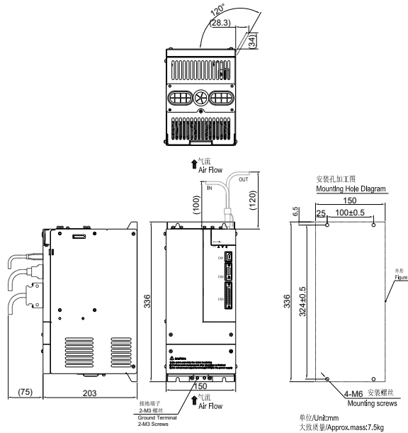
图 3.1.7 伺服驱动器结构尺寸 6
