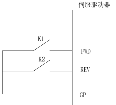
图 6.1.2 两线式运转模式 2 接线示意图
