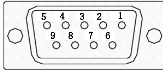
图 4.2.5 Biss-C 型编码器端子排列示意图
