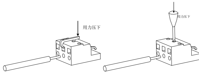
图 4.1.3 主电路端子使用方法
