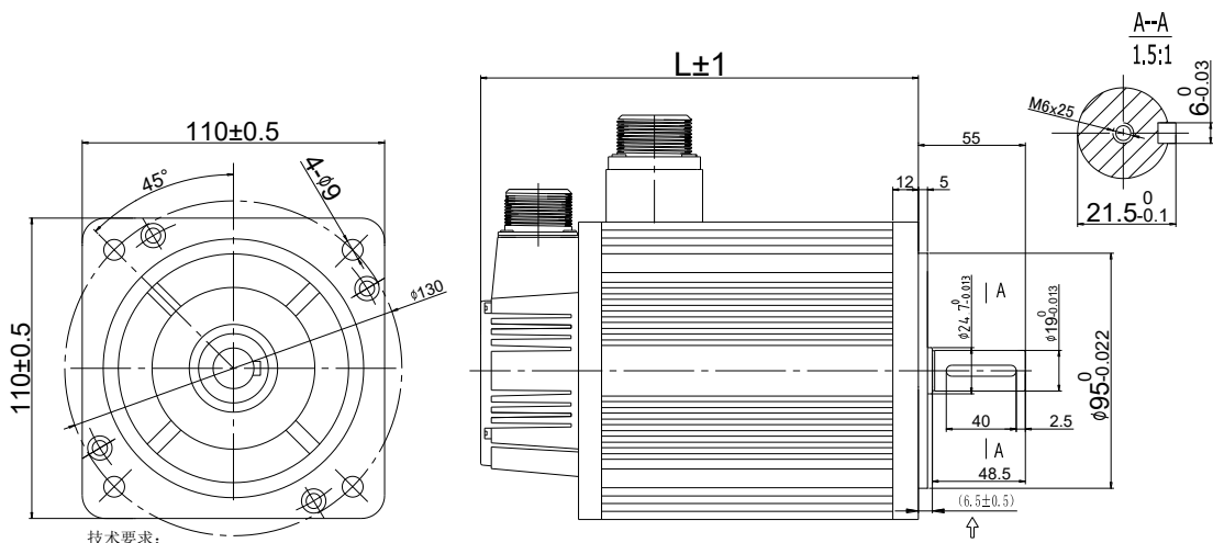
110 法兰伺服电机外形尺寸图
