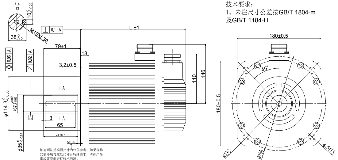
180 法兰伺服电机外形尺寸图
