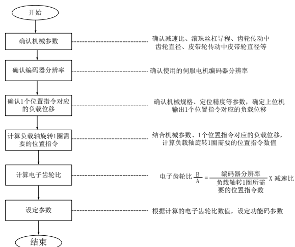
图 7.2.1 电子齿轮比设置步骤流程图
