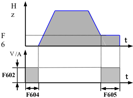
图 6-20 直流制动
