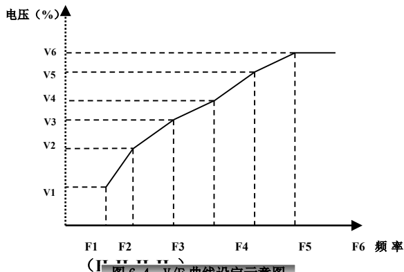
图 6-4 V/F 曲线设定示意图
