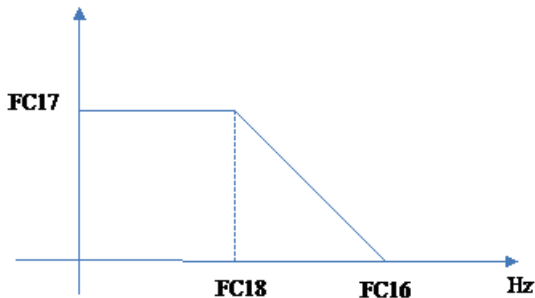
图 6-26 转矩偏置补偿示意图
