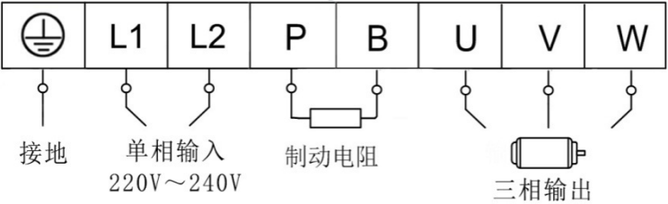
图 4-2 端子示意图
