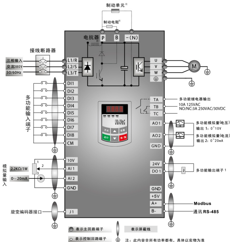
图 4-15 三相变频器标准配线图 (NPN 方)
