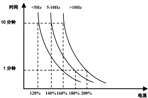
图 6-22 不同频率下的电机过载保护值
