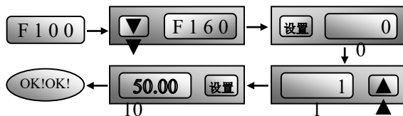
图 6-5 恢复出厂值
