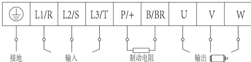
图 4-4 端子示意图
