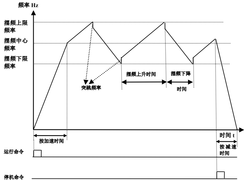
图 6-6 摆频模式 1 工作示意图
