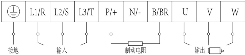
图 4-5 端子示意图
