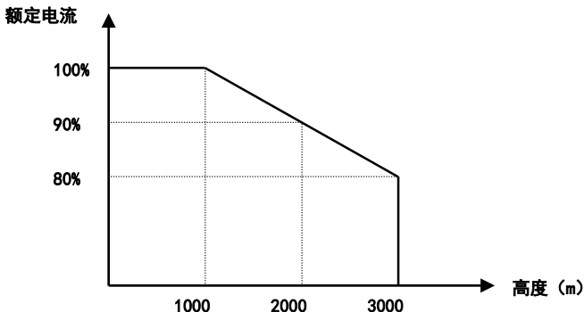
图 1-1 变频器额定电流与海拔高度降额曲线图
