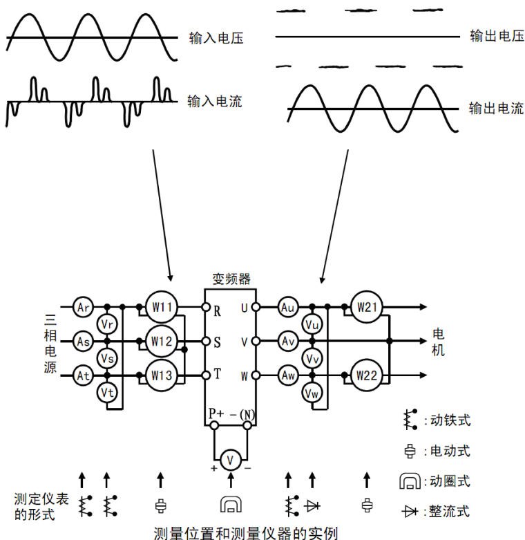
图 4-14 测量示意图
