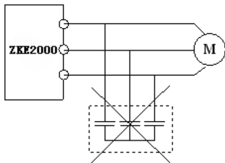
图 1-4 变频器输出端禁止使用电容器
