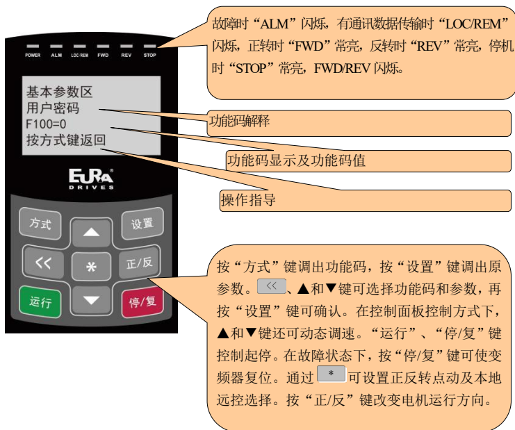
图 3-3 控制面板示意图
