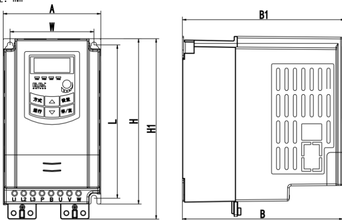
塑壳外形
