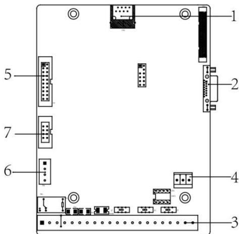
图 2-6 E7 及铁壳接口图
