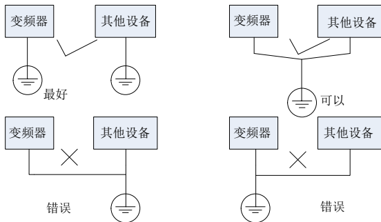
图 4-16 接地示意图
