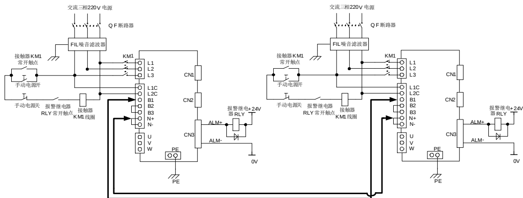
图 4.1. 720V 驱动器共直流母线配线图
