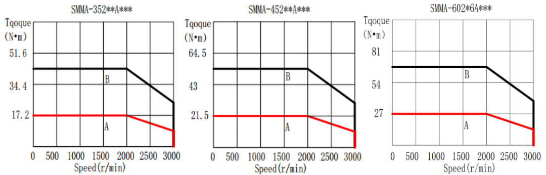
180 法兰伺服电机转矩-转速特性曲线
