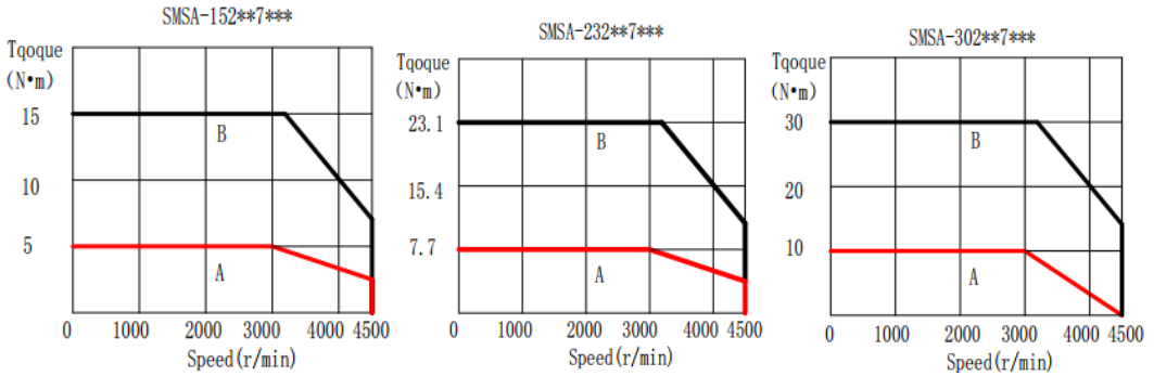
130 法兰伺服电机转矩-转速特性曲线
