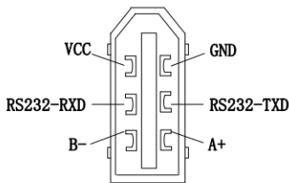
(焊片侧)
