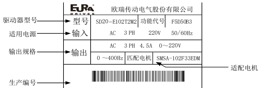
图 2.1.3 伺服驱动器铭牌
