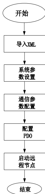
图 6.1.2 EtherCAT 使用设置流程图
