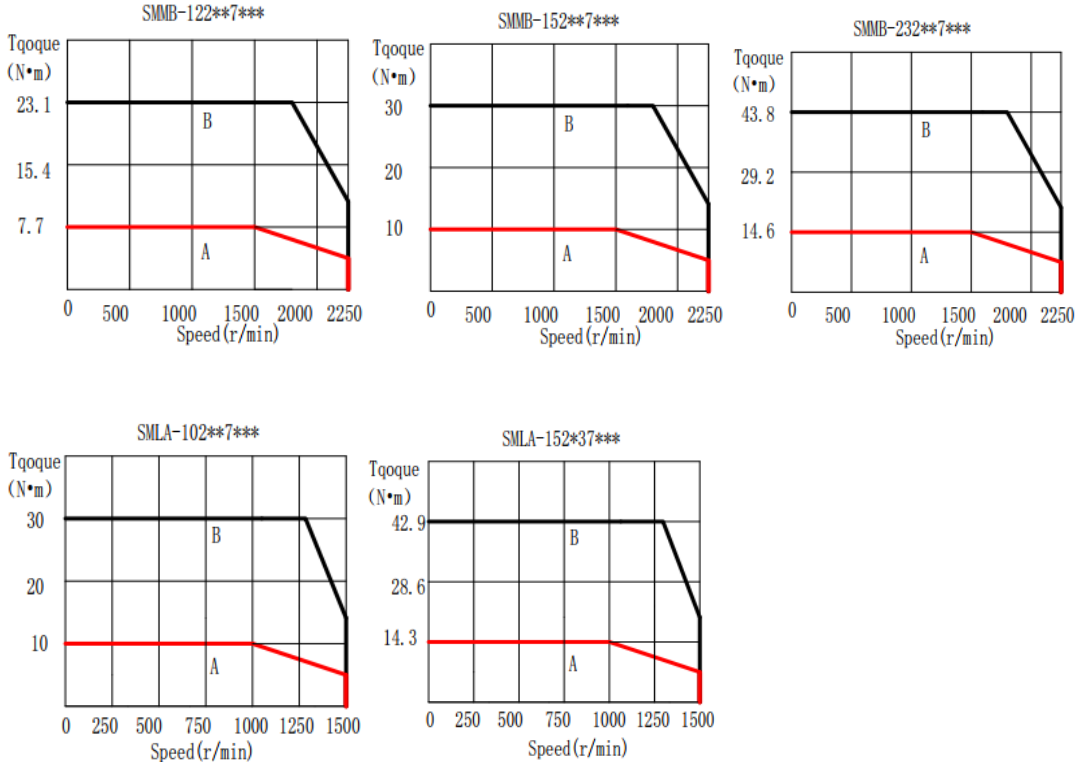
180 法兰伺服电机转矩-转速特性曲线
