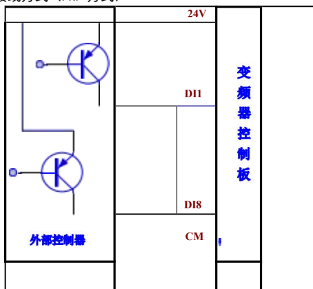
图 4-11 有源共漏极接线方式示意图
