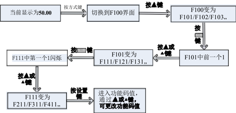
图 5-1 功能码区内和区间切换
