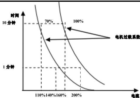
图 6-21 电机过载系数设定
