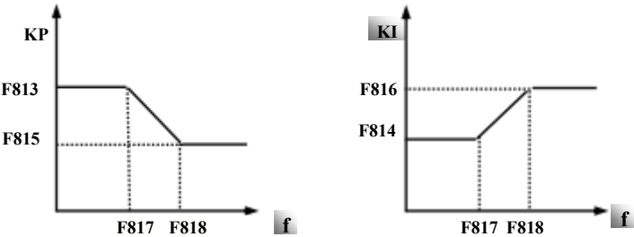
图 6-2 PI 参数示意图
