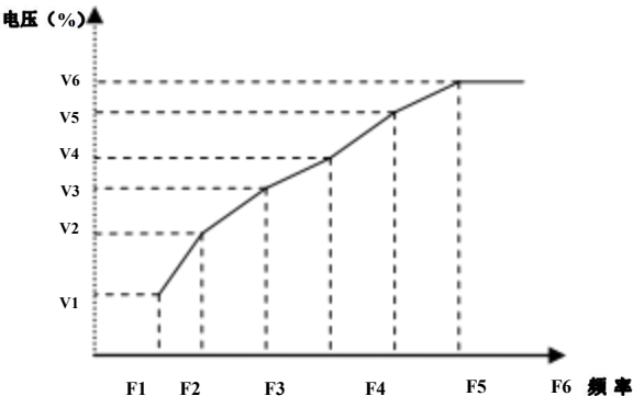
图 6-4 V/F 曲线设定示意图
