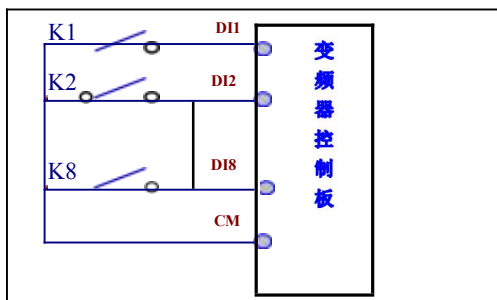
图 4-8 无源共源极接线方式示意图
