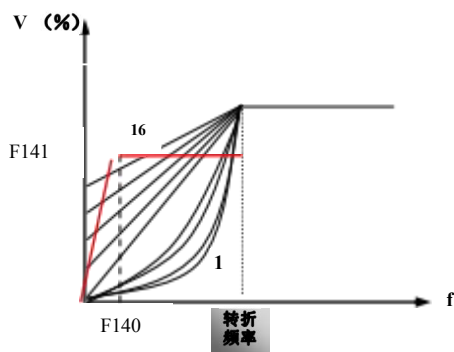
图 6-3 转矩提升示意图
