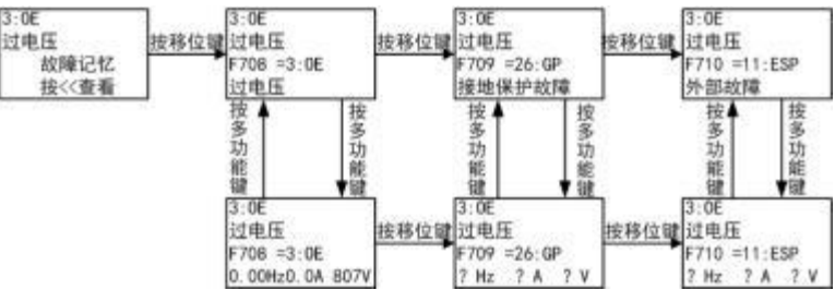
图 5-6 故障界面操作流程
