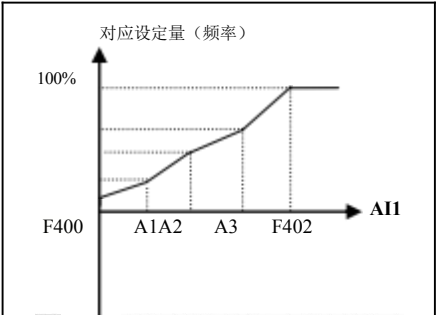
图 6-18 折线式模拟量输入与设定量关系
