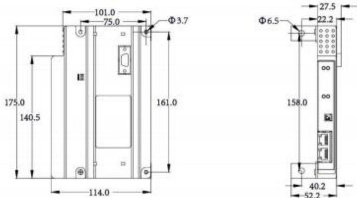
图 11-2 变频器 EtherCAT 总线卡尺寸图
