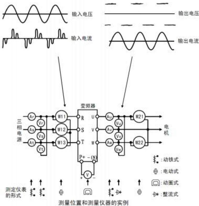
图 4-13 测量示意图
