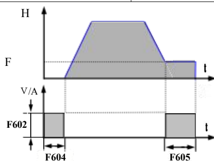
图 6-20 直流制动
