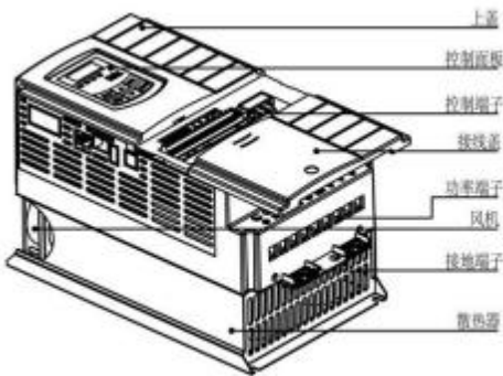
图 2-4 产品外形及结构部件图
