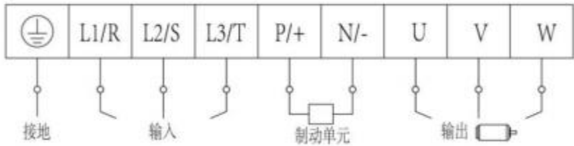
图 4-7 端子示意图
