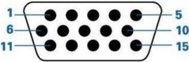
图 11-7 接口引脚图
