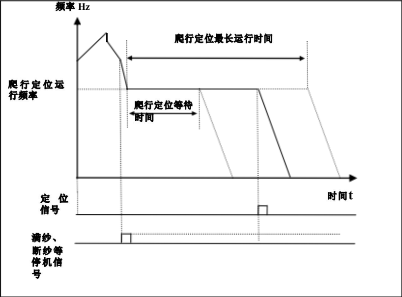
图 6-8 爬行定位工作模式示意图
