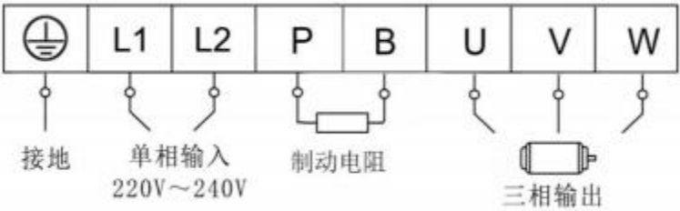
图 4-2 端子示意图
