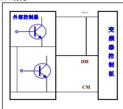
图 4-9 有源共源极接线方式示意图
