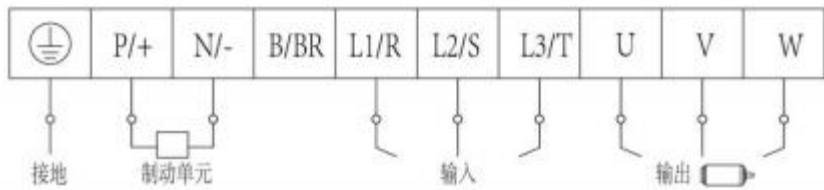
图 4-6 端子示意图
