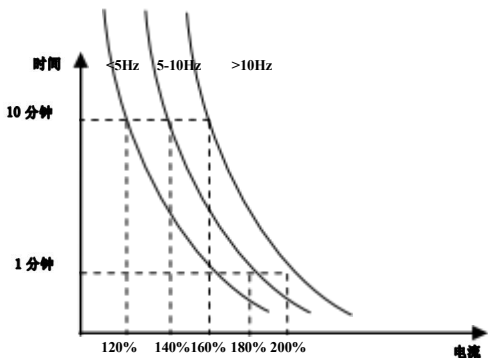
图 6-22 不同频率下的电机过载保护值
