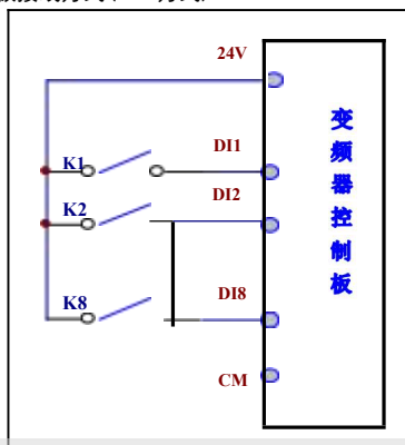
图 4-10 无源共漏极接线方式示意图
