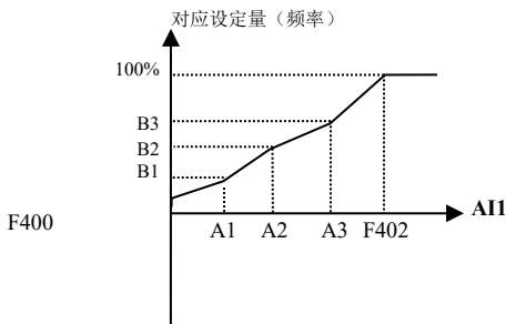
图 6-14 折线式模拟量输入与设定量关系
