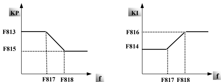
图 6-20 PI 参数示意图
