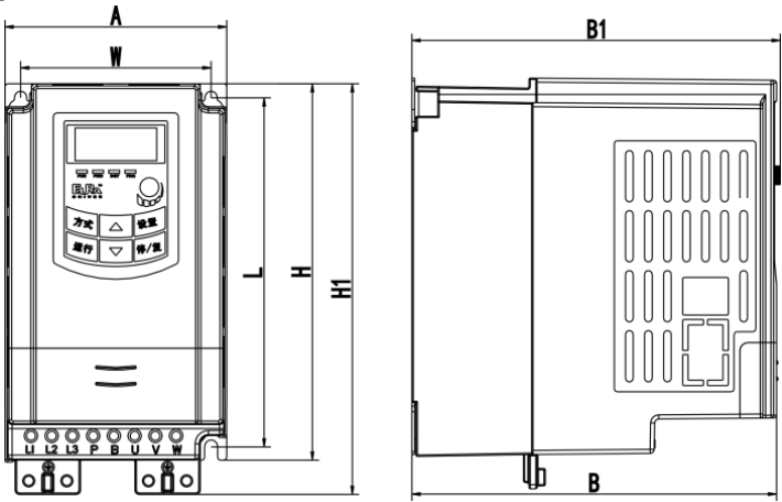
塑壳外形
