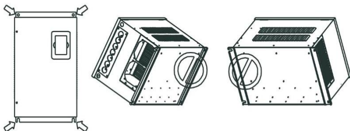
图 1-2 变频器垂直安装示意图
