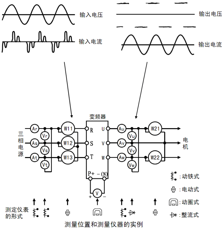
图 4-11 测量示意图
