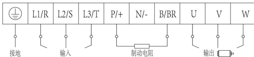
图 4-3 端子示意图
