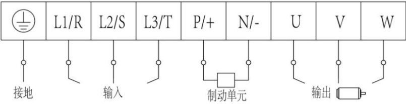
图 4-5 端子示意图
