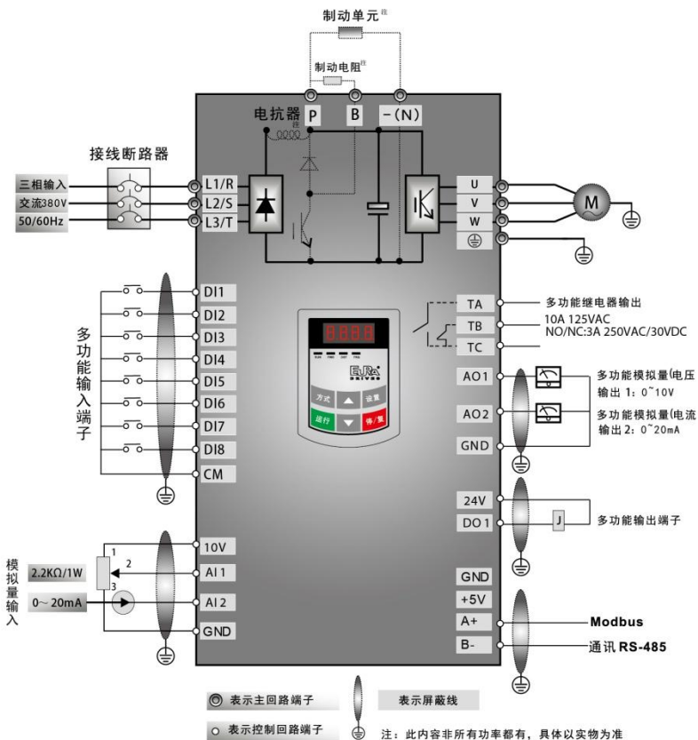
图 4-12 三相变频器标准配线图 (NPN 方
