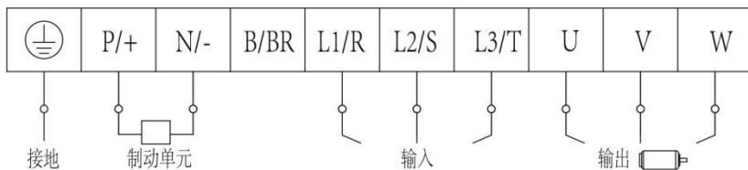
图 4-4 端子示意图
