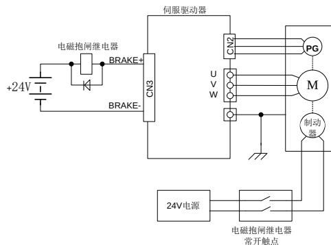
图 7.1.2 抱闸器接线示意图
