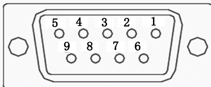
图 4.2.2 旋转变压器编码器端子排列示意图
