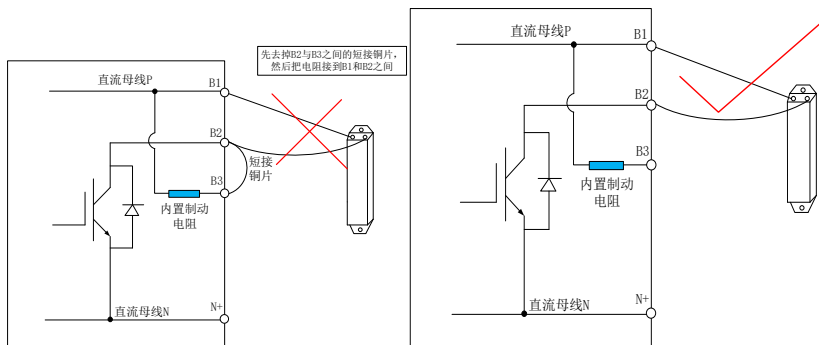
图 7.1.11 伺服制动电阻接线示意图
