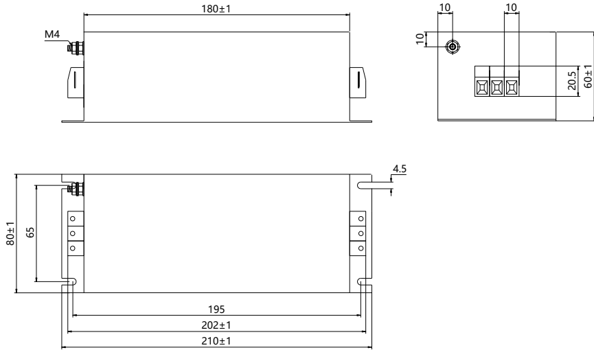
图 2.4.2 FT330 系列外形尺寸图
