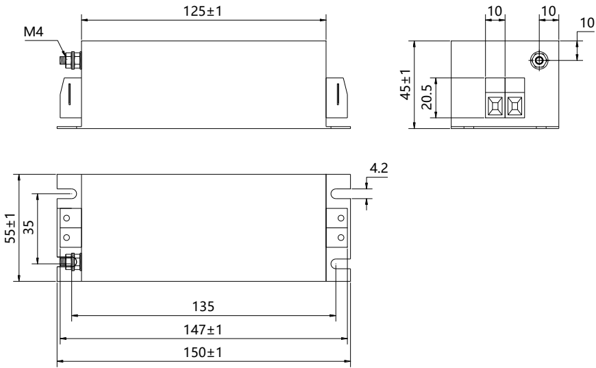
图 2.4.1 FT130 系列外形尺寸图
