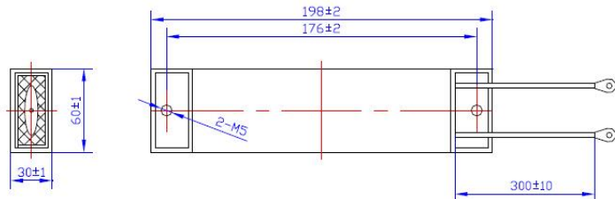
图 7.1.12 伺服制动电阻接线示意图
