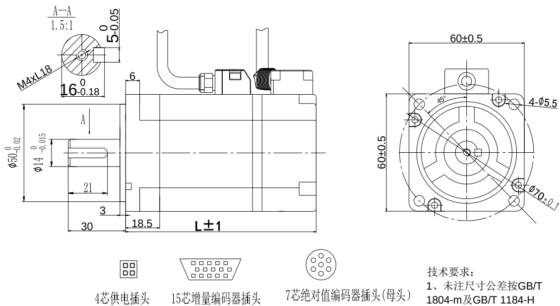
60 法兰五对极伺服电机外形尺寸图
