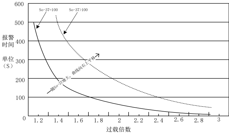
图 7.3.1 电机过载曲线与报警时间曲线图
