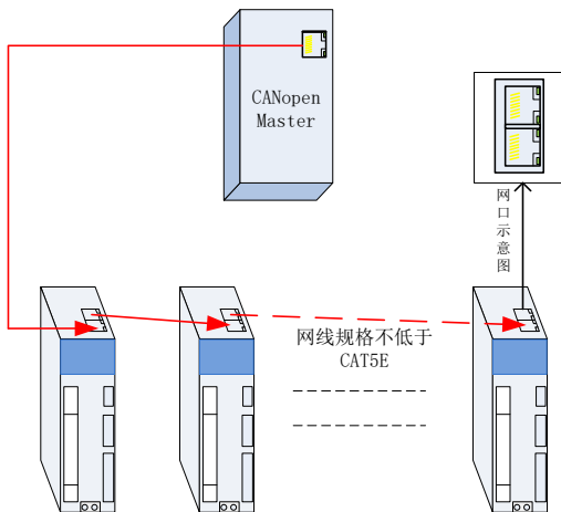
图 6. 1. 1CANopenfs 网络连接示意图
