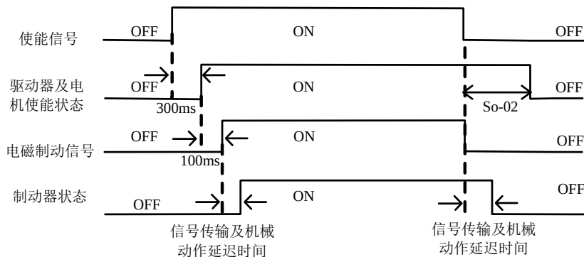
图 7.1.3 电磁抱闸制动时序图
