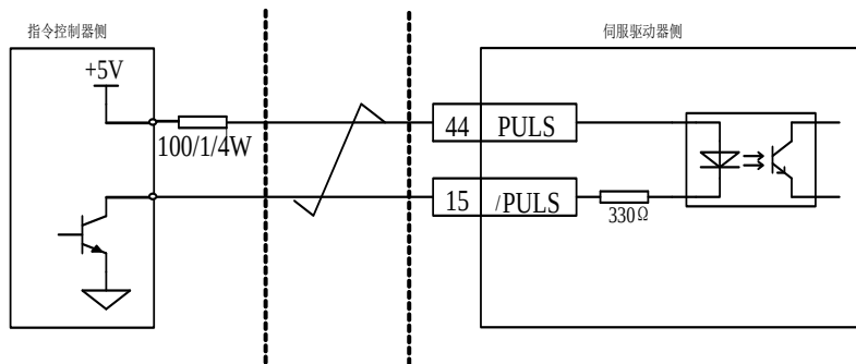
图 4.3.5 5V 集电极开路脉冲输入接口电路
