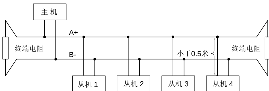
图 6.4.2 终端电阻的连接图
