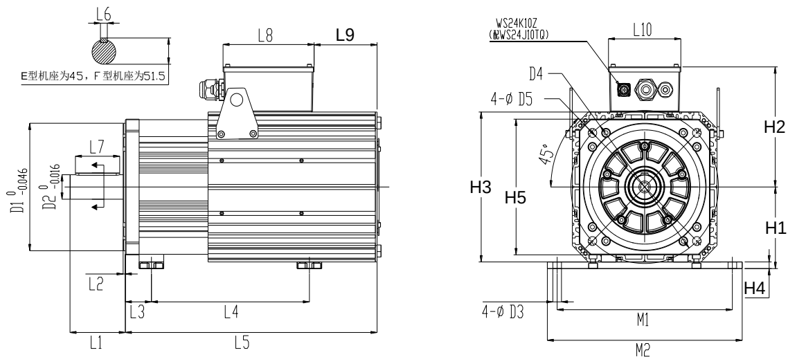
180 及 250 止口伺服电机外形尺寸图
