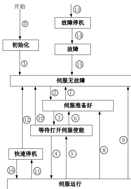
图 7.2.1 CiA402 状态机切换图
