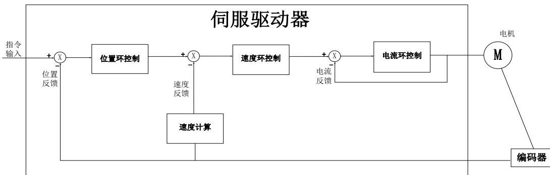
图 7 伺服系统控制框架图
