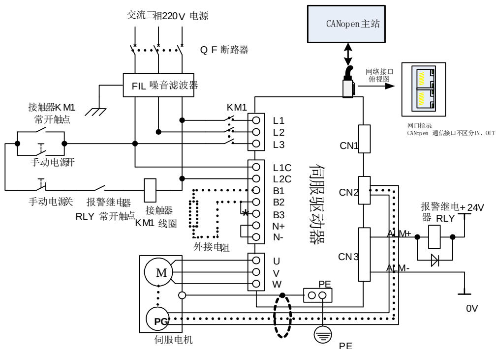
图 4.1.4 220V 驱动器典型主电路配线图
