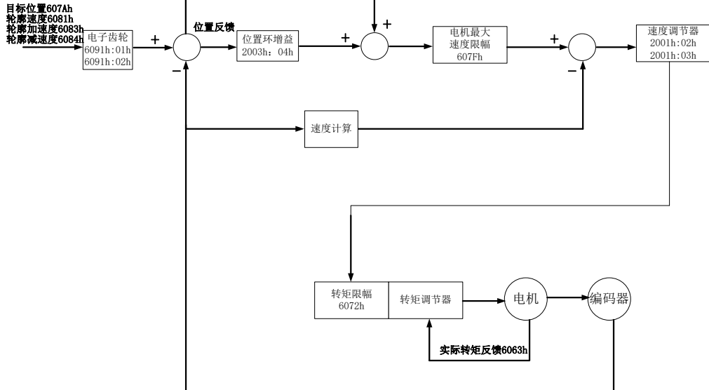
图 7.3.1 轮廓位置模式 (PP) 控制框图
