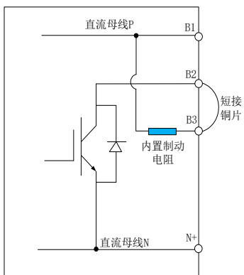
图 7.1.10 伺服内部能耗制动示意图
