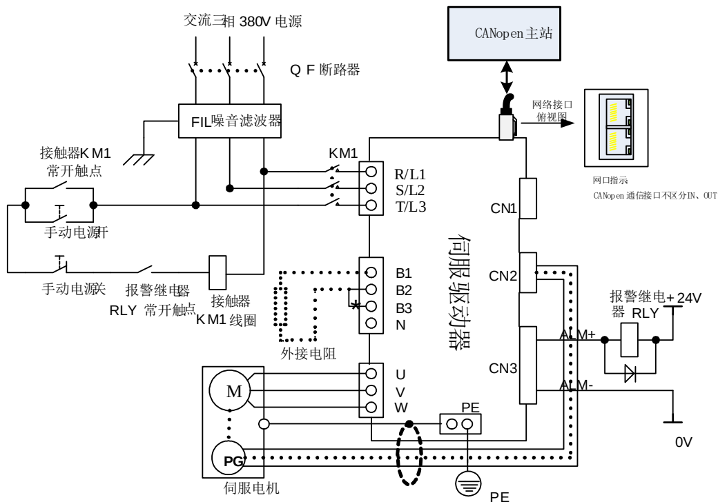
图 4.1.5 380V 驱动器典型主电路配线图
