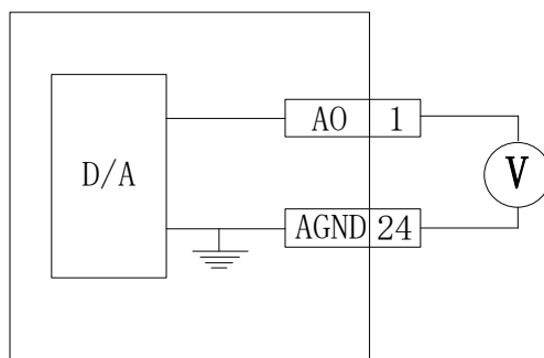
图 4.3.12 模拟量监控输出接口
