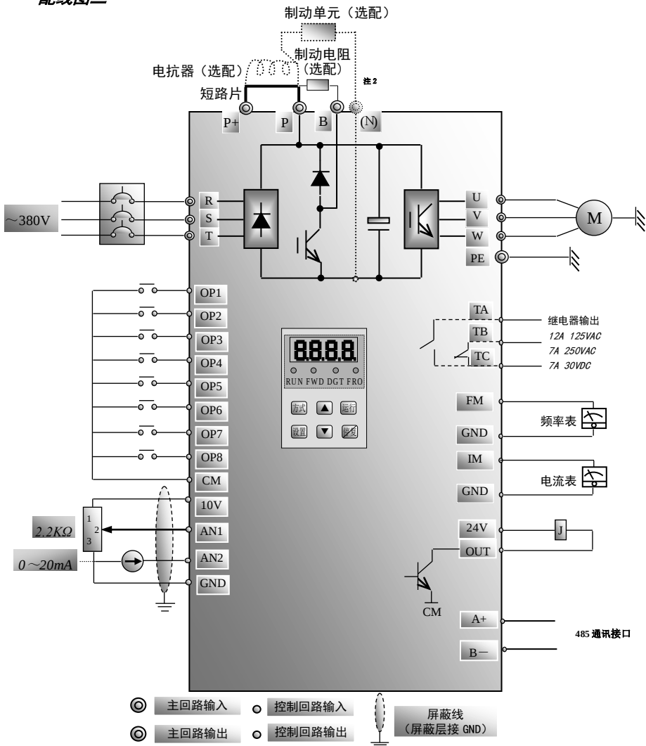
配线图二
