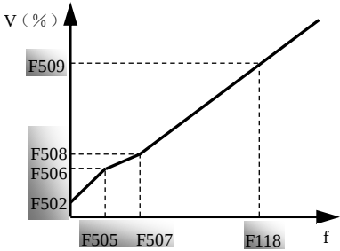
图 5-8 折线式 V/F 曲线
