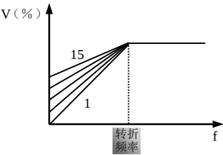
图 5-7 转矩提升示意图
