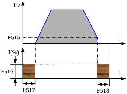
图 5-9 直流制动
