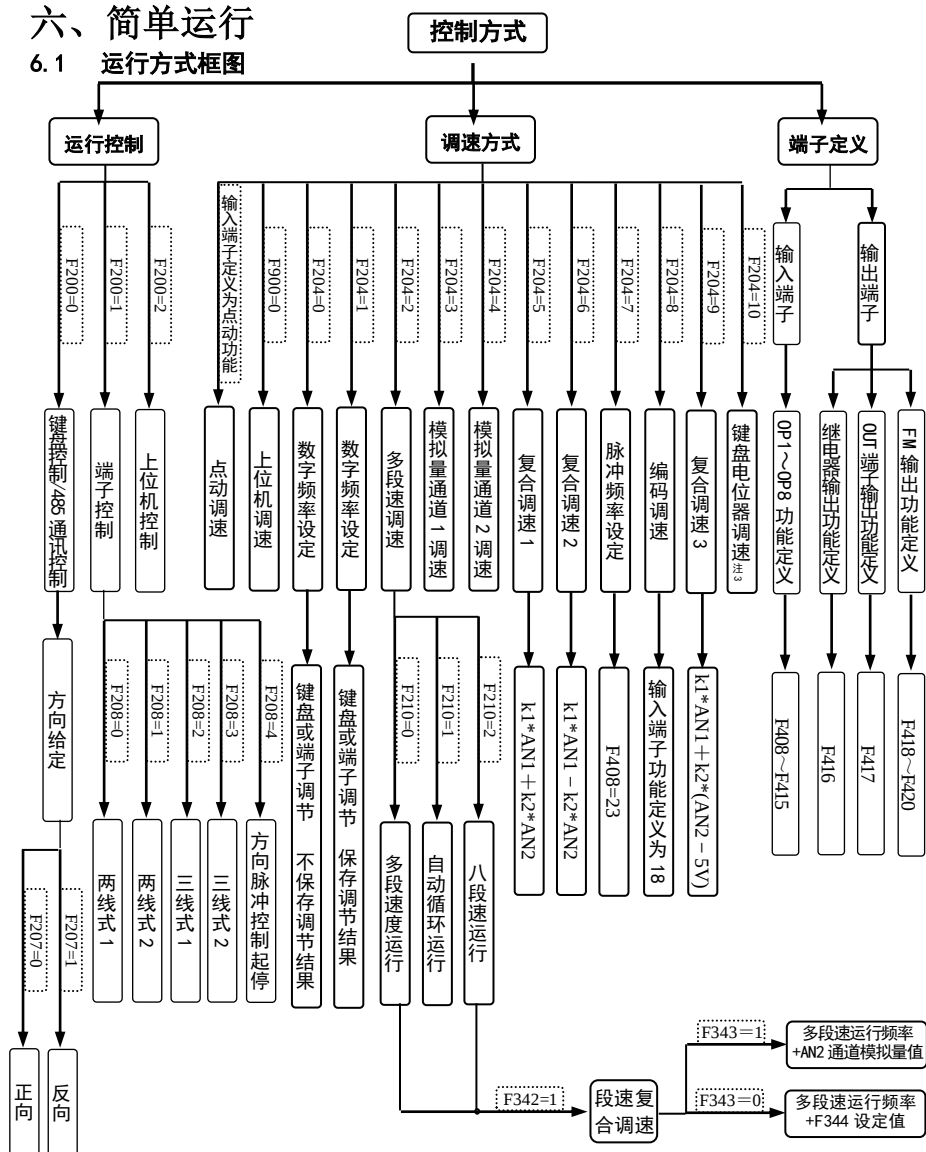
图 6-1 运行方式框图
