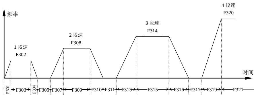
图 6-3 自动循环运行（停机等待时间大于零）
