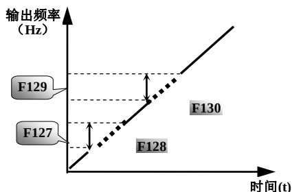
图 5-2 频率回避示意图
