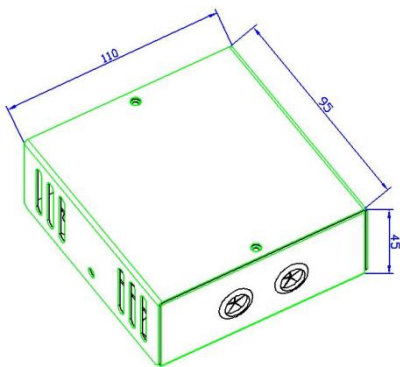
附图 5-2 多泵控制盒外观尺寸 110mm*95mm*45mm（长*宽*高）
