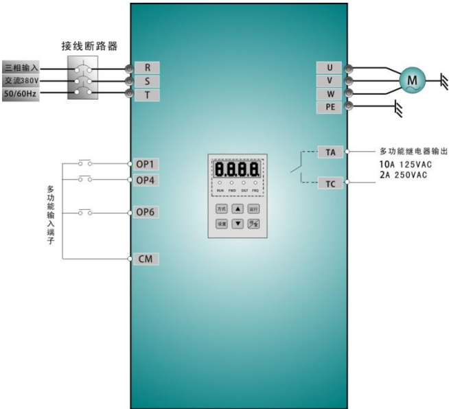
图 4—2 接线图 2
