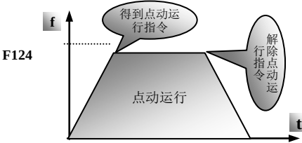
图 5-1 点动运行
