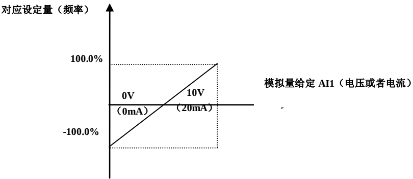
图 5-8 模拟给定与设定量的对应关系
