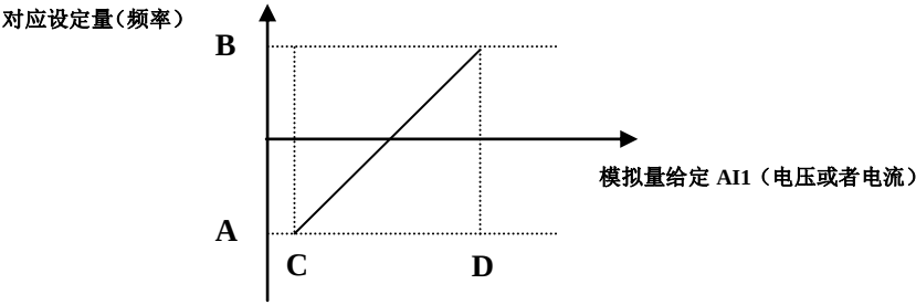
图 5-6 F400~F403 设定图示
