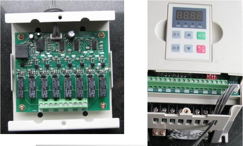
附图 5-3 扩展盒和变频器内部接线图（以 F2000-P0022T3B 为例）
