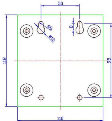
附图 5-1 多泵控制盒安装尺寸 95mm*50mm，使用 4 个 \Phi 6 螺丝安装
