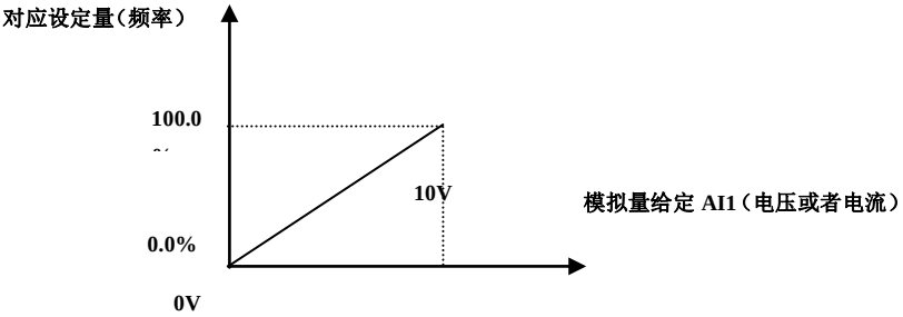
图 5-7 模拟给定与设定量的对应关系
