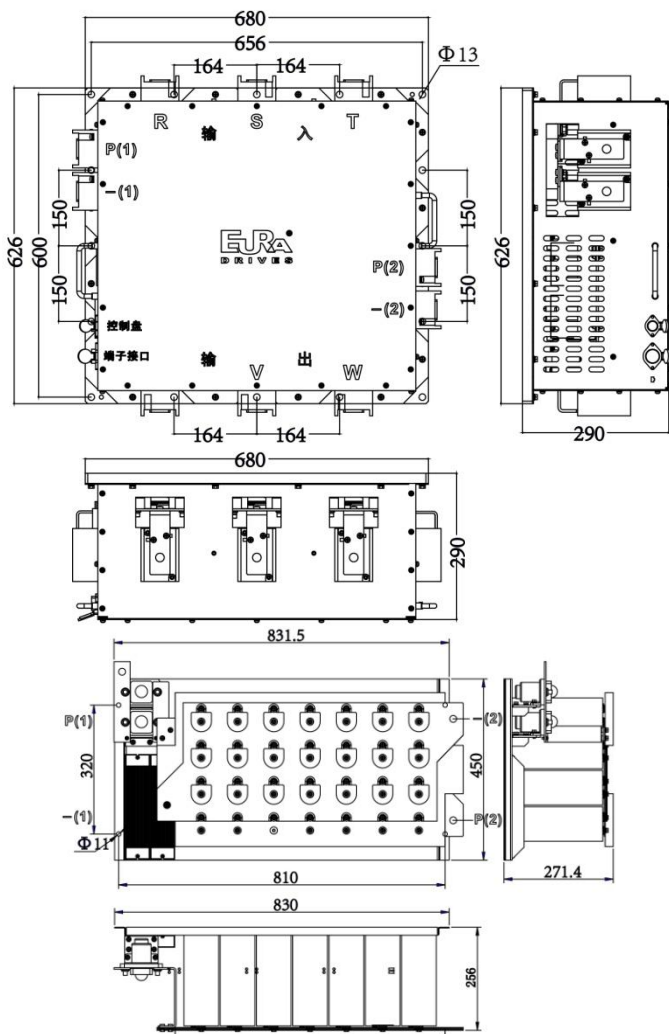
图 7-10 FB92-8Z 结构尺寸和连接
