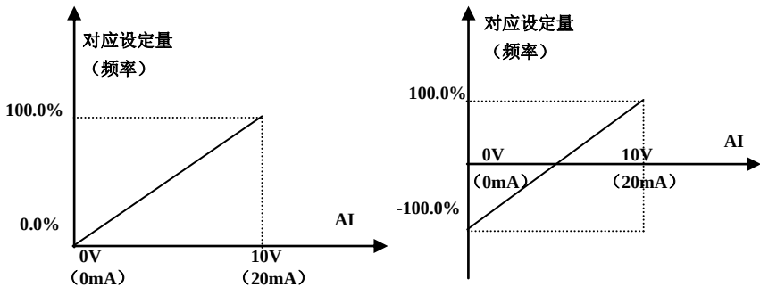
图 6-13 模拟给定与设定量的对应关系
