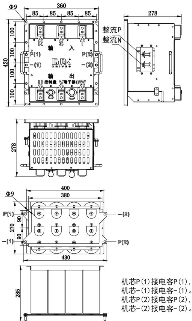
图 7-3 FB62-3Z 结构尺寸和连接
