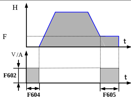
图 6-19 直流制动
