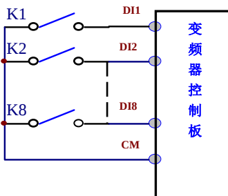
图 4-1 无源共源极接线方式示意图
