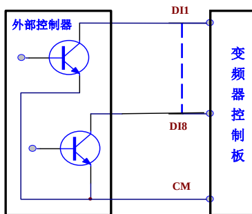
图 4-2 有源共源极接线方式示意图
