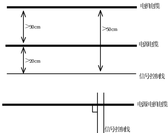
图 4-10 现场配线示意图
