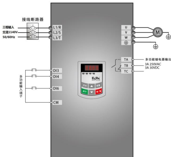
图 5-2 接线图 2
