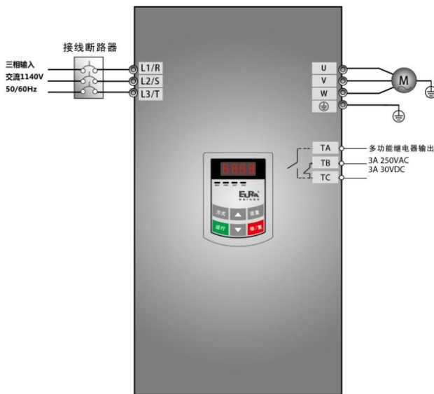
图 5-1 接线图 1
