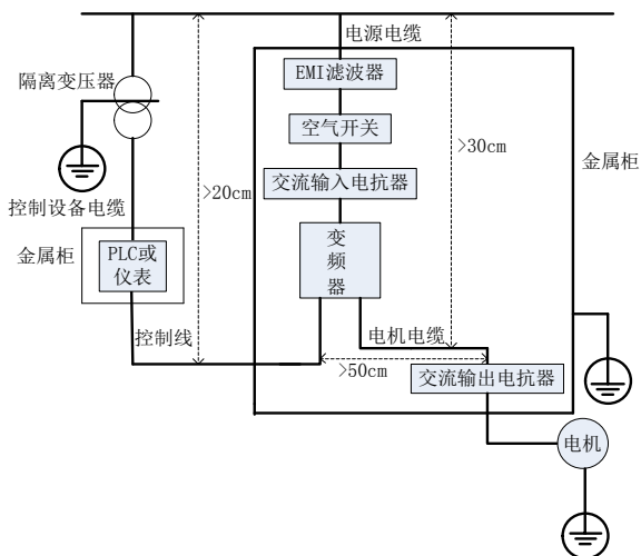
图 4-12 电气安装示意图
