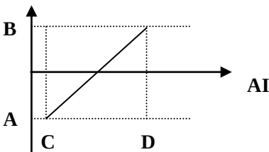
图 6-14 模拟给定与设定量的计算关系
