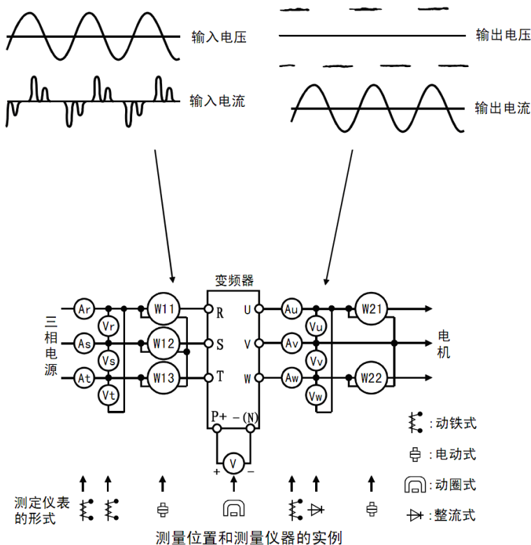
图 4-6 测量示意图
