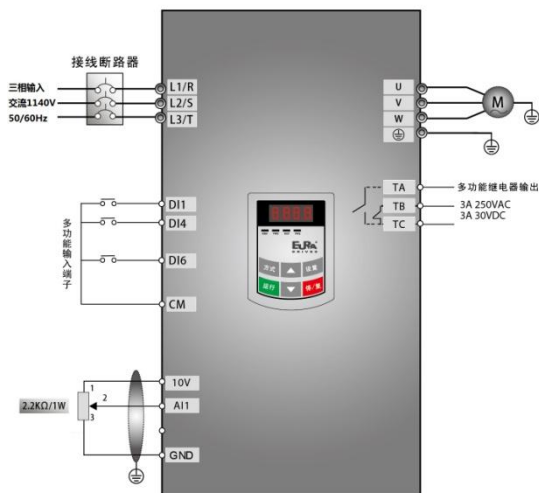
图 5-3 接线图 3
