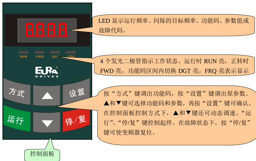
图 3-1 控制面板示意图
