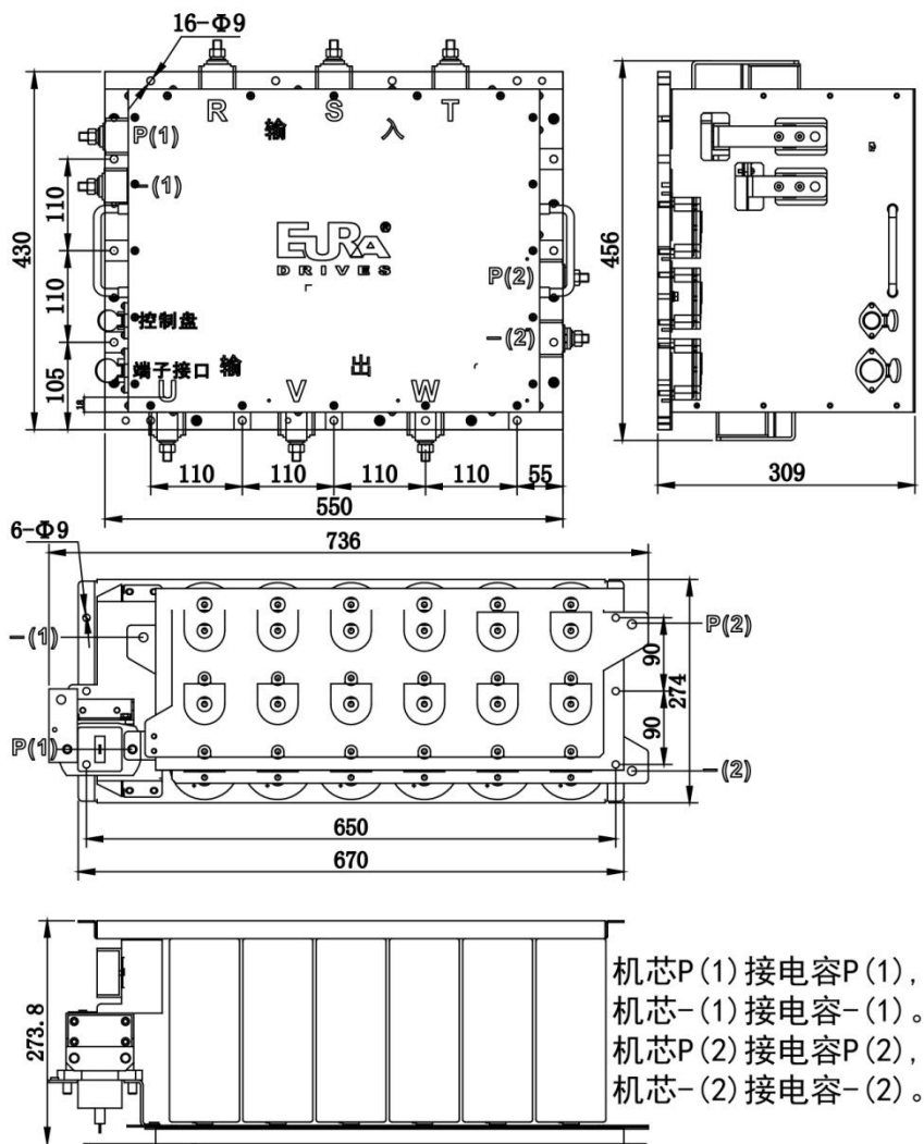
图 7-8 FB92-6Z 结构尺寸和连接
