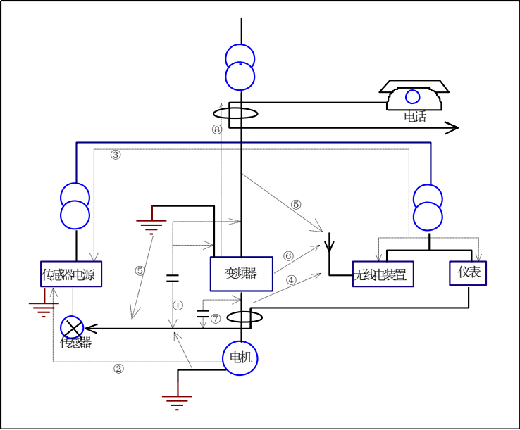
图 4-9 噪声传播途径
