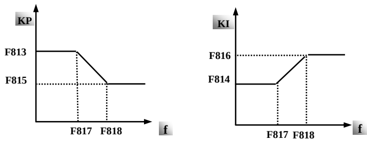
图 6-23 PI 参数示意图
