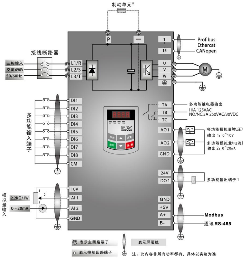
图 4-7 三相变频器标准配线图（NPN 方式）
