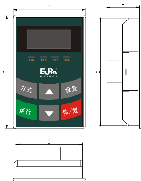
图 3-3 控制面板结构示意图
