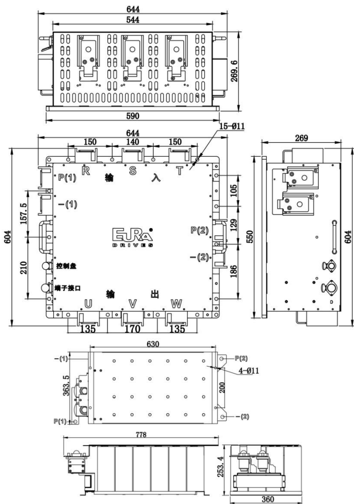
图 7-9 FB92-7Z 结构尺寸和连接
