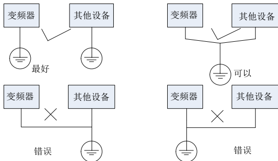
图 4-11 接地示意图
