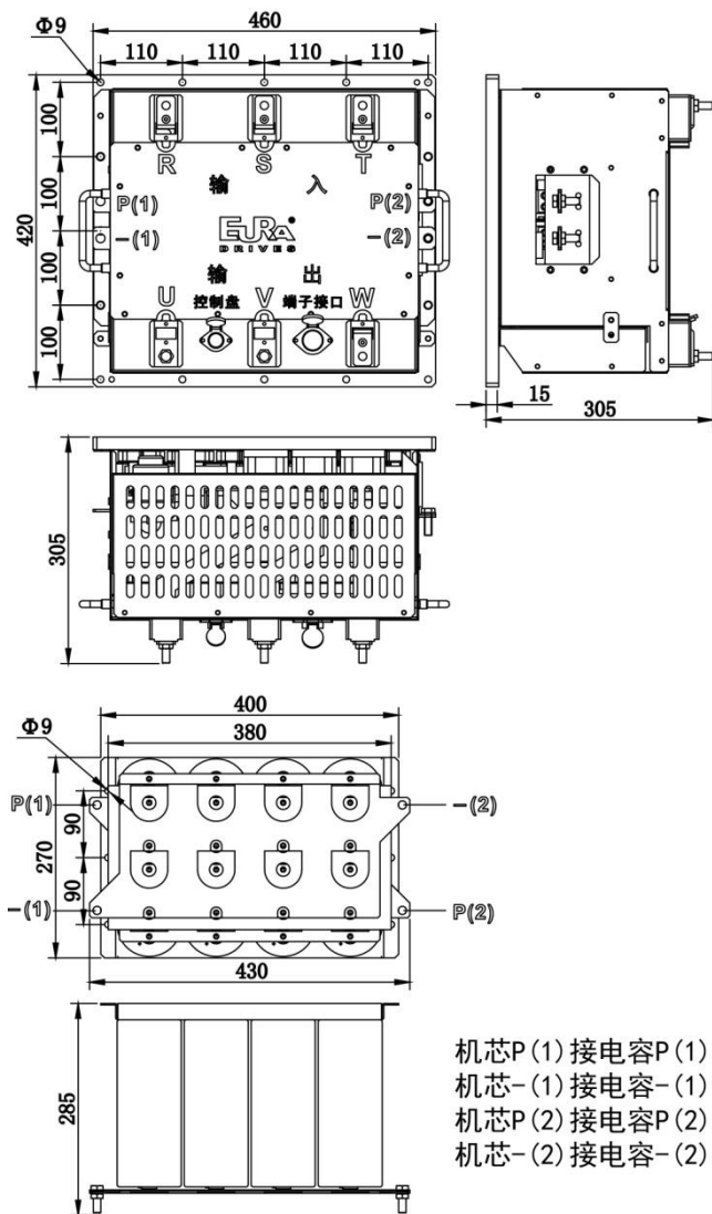
图 7-4 FB62-4Z 结构尺寸和连接
