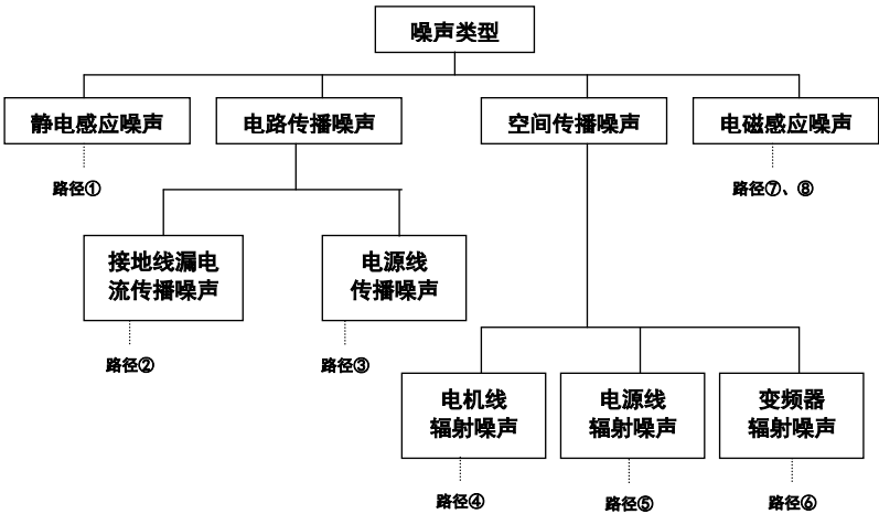
图 4-8 噪声类型图示
