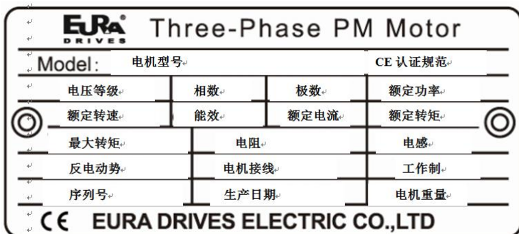
图 8-1 EVPM 电机铭牌
