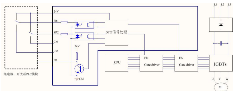
图 5-6 STO 功能原理示意图
