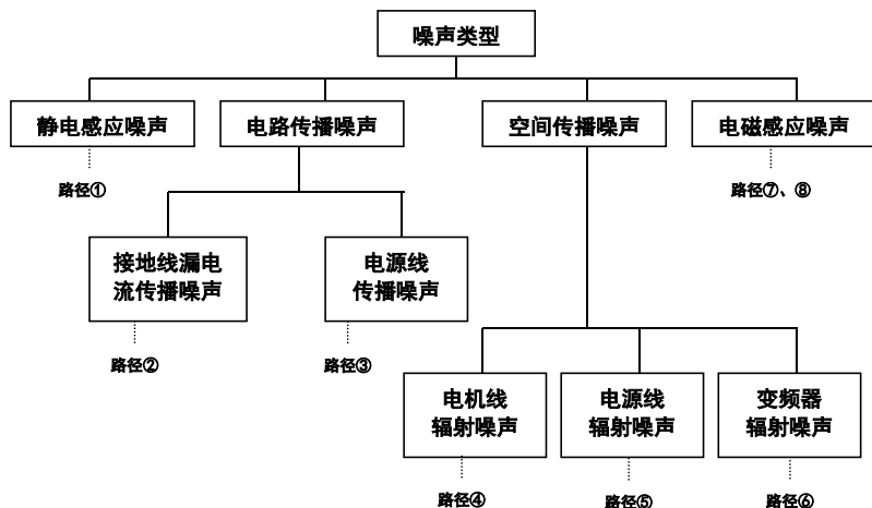
图 4-13 噪声类型
