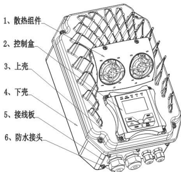
图 2-5 产品外形及结构部件图
