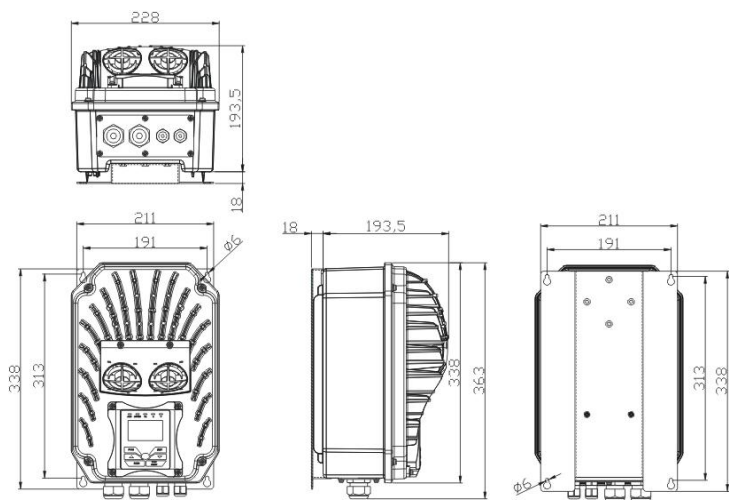
附图 3-3 驱动器 J2 壁挂尺寸图
