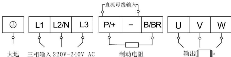
图 4-3 端子示意图
