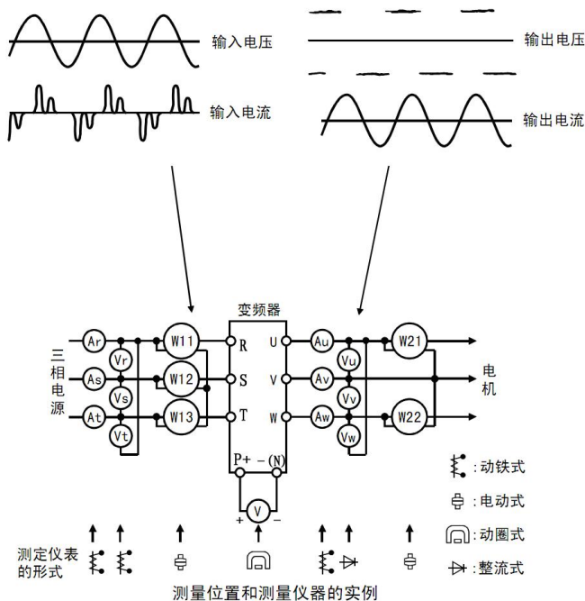
图 4-11 测量示意图
