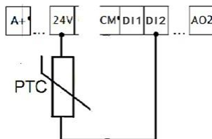
图 6-8 PTC 保护示意图
