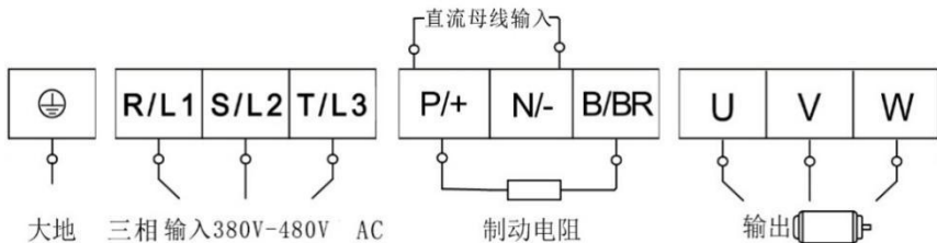
图 4-4 端子示意图
