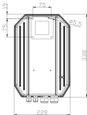
附图 3-4 驱动器 J2 与电机安装尺寸图
