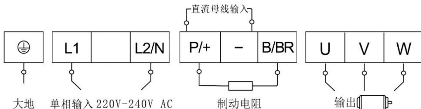
图 4-2 端子示意图
