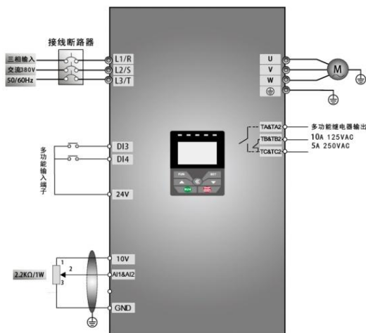
图 5-3 接线图 3
