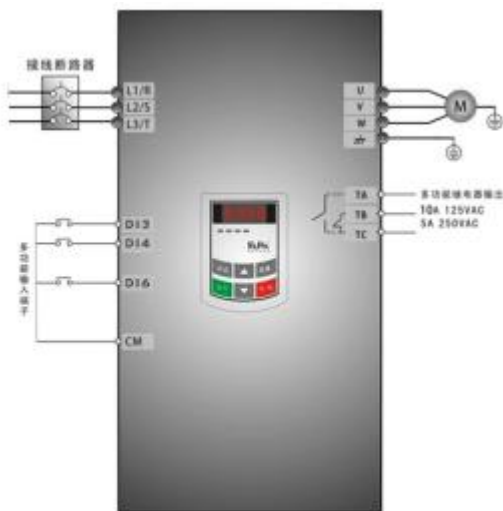
图 5-8 接线图 2
