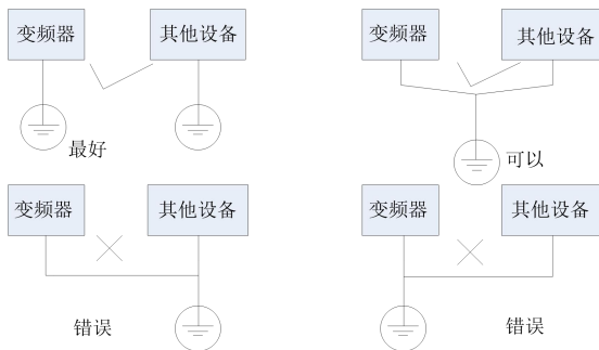
图 4-15 接地示意图
