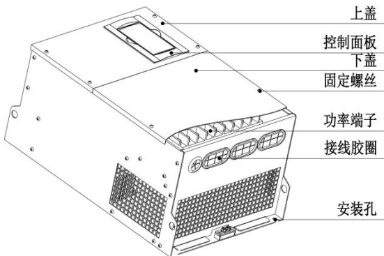
图 2-4 产品外观图
