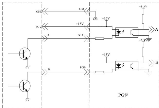
开路集电极输出编码器
