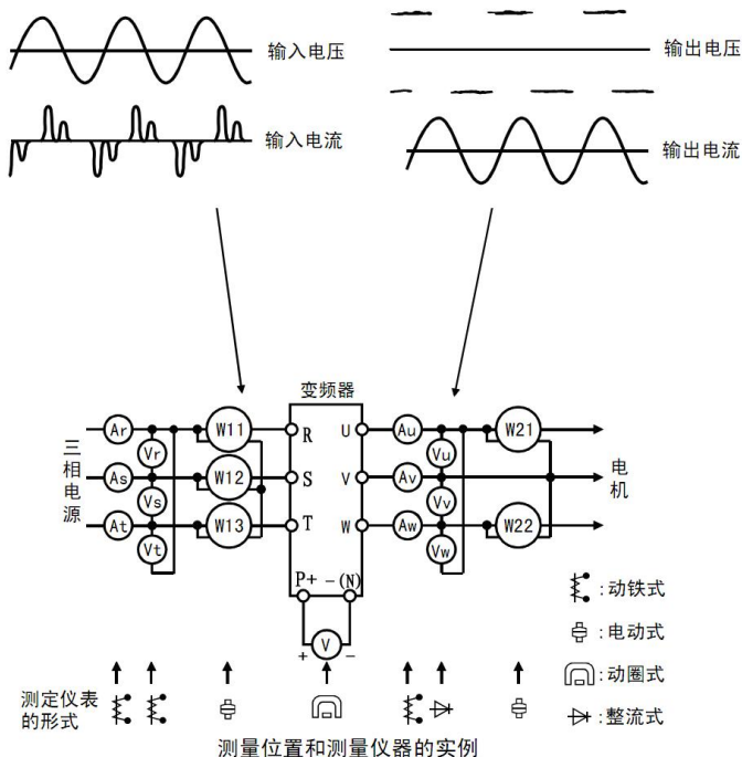
图 4-10 测量示意图
