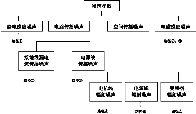
图 4-12 噪声类型图示
