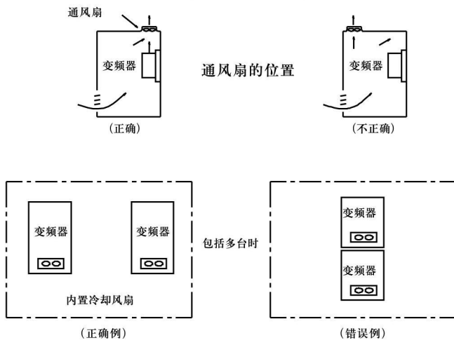
图 1-3 变频器安装在控制柜内示意图
