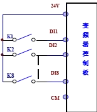
图 4-7 无源共漏极接线方式示意图
