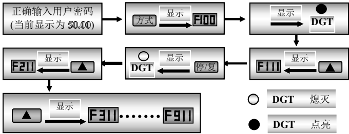
图 3-7 功能码区内和区间切换
