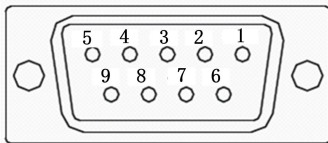
图 4-4 旋转变压器编码器端子排列示意图
