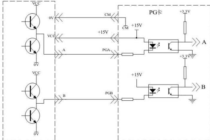
推挽输出编码器
