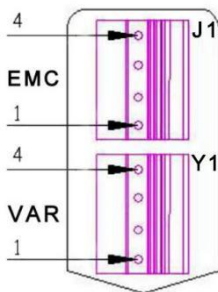
图 4-17 安规/压敏短接跳线接插件 J1/Y1
