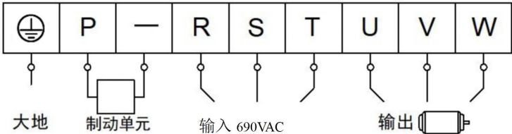
图 4-2 接线示意图
