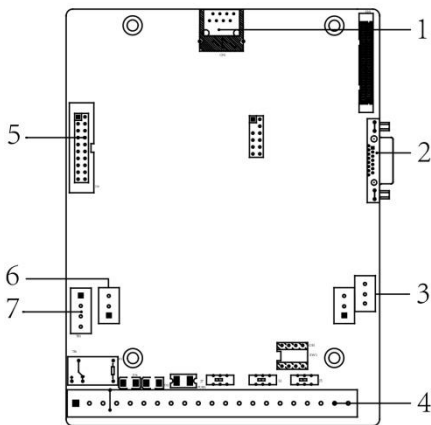
图 2-5 接口介绍
