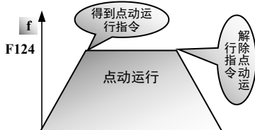
图 6-1 点动运行
