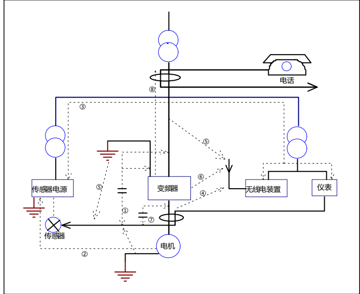
图 4-12 噪声类型图示
