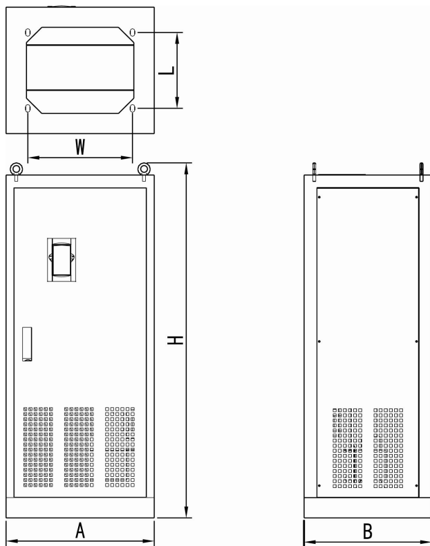
690V 柜式金属机壳外形
