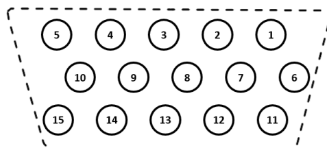
图 2-7 DB15 端子排列示意图
