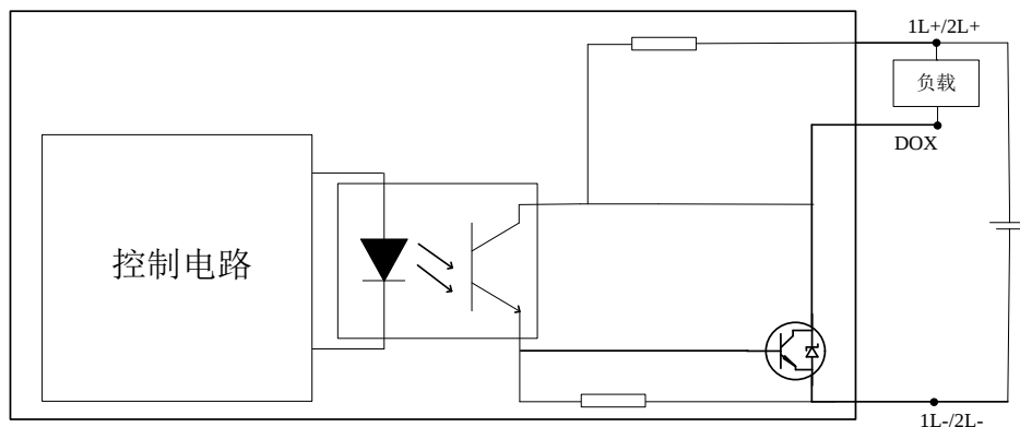
图 2-5 D0 输出通道电气原理图
