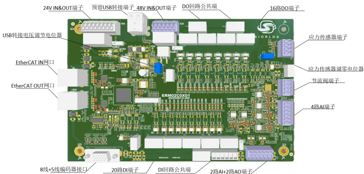
图 2-1 ERMS243S-36DTD-A80 整体视图
