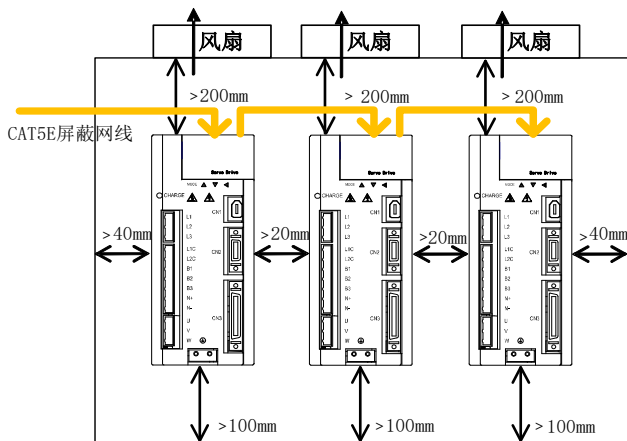
图 3.1.2 多台并列安装最小安装尺寸示意图
