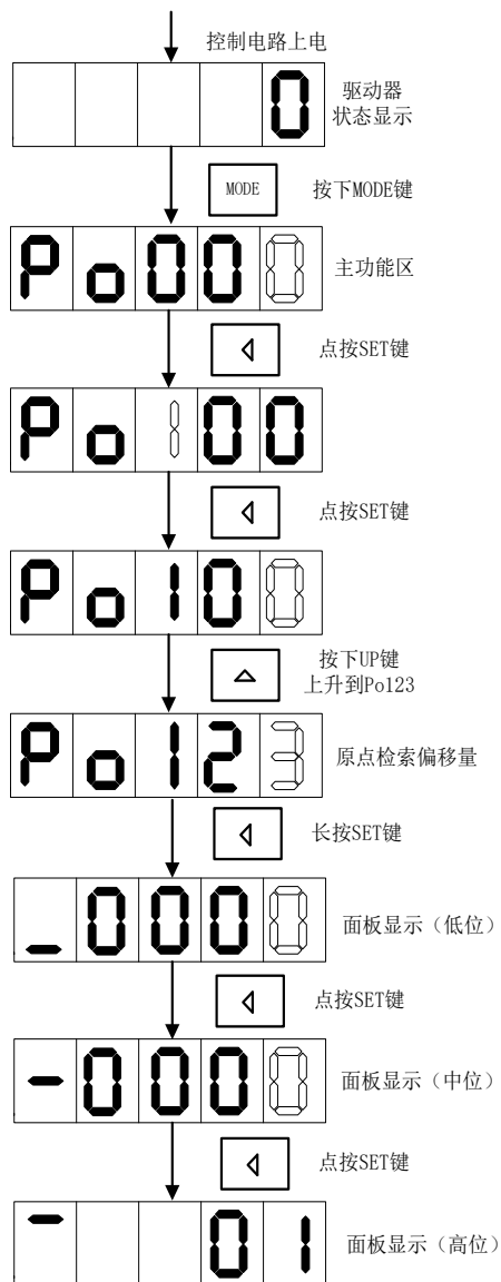
图 5.3.4 用户参数的设置示意
