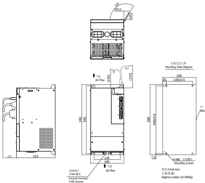
图 3.1.7 伺服驱动器结构尺寸 7
