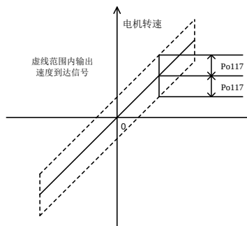
图 7.2.5 速度到达信号输出示意图
