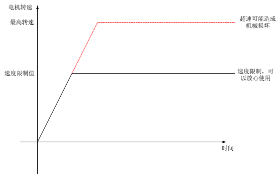
图 7.2.8 转矩模式下速度限制示意图
