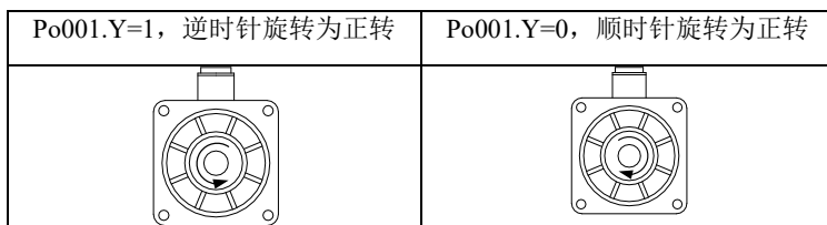
图 6.1.6 电机旋转方向示意图
