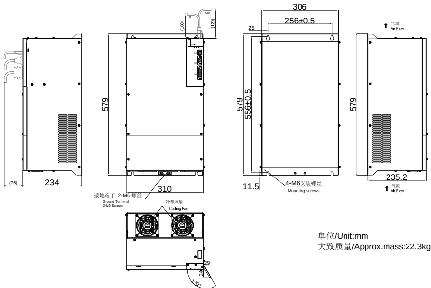
图 3.1.11 伺服驱动器结构尺寸 11
