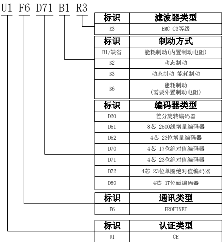
图 2.1.2 伺服驱动器功能部分命名规则
