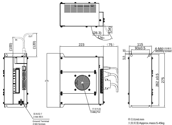
图 3.1.6 伺服驱动器结构尺寸 6
