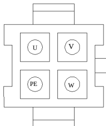
图 4.4.1 4 芯航电源安普插头示意图
