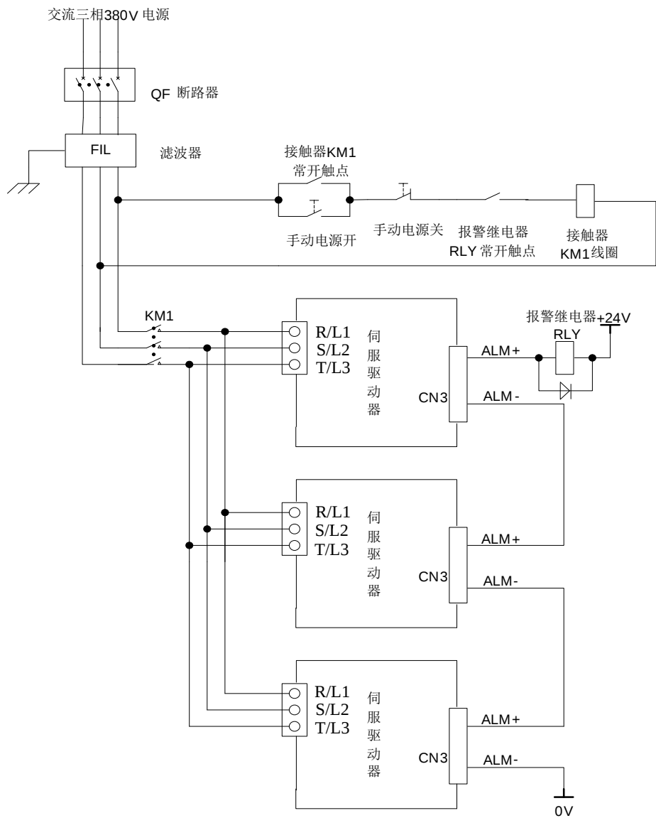
图 4.3.25 380V 多台联机时的接线
