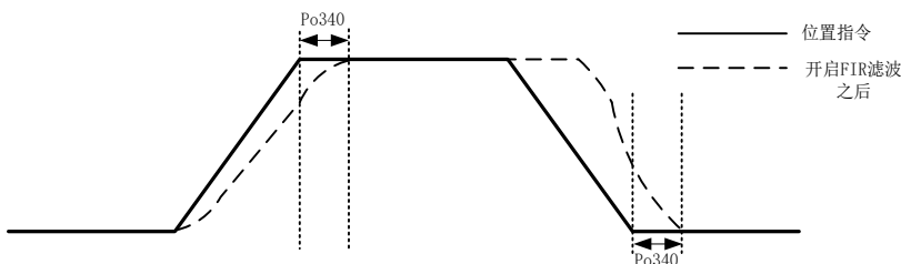
图 8.3.5 梯形位置指令与 FIR 滤波器之后的位置指令示意图
