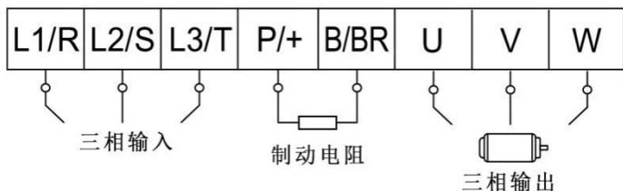
图 4-3 端子示意图
