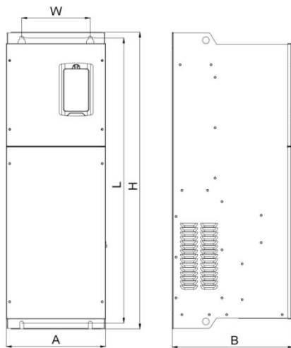
L5-LB 金属壁挂外形
