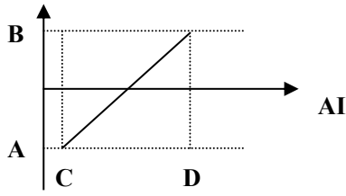
图 6-15 模拟给定与设定量的计算关系
