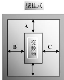
图 4-1 变频器安装示意图
