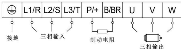
图 4-5 端子示意图
