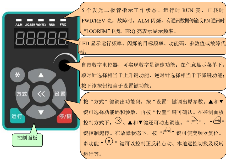
图 3-1 控制面板示意图
