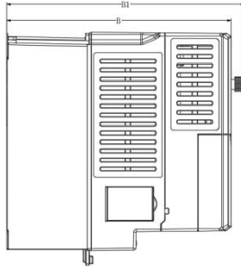
塑壳外形
