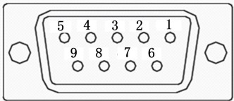
图 4-9 绝对值编码器端子排列示意图
