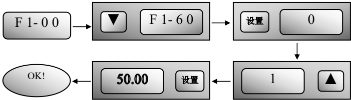
图 6-5 恢复出厂值
