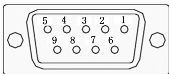
图 4-8 旋转变压器编码器端子排列示意图
