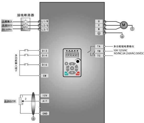
图 5-9 接线图 3
