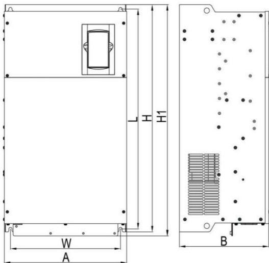
C4A-C61 金属壁挂外形
