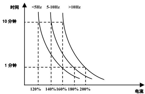
图 6-22 不同频率下的电机过载保护值
