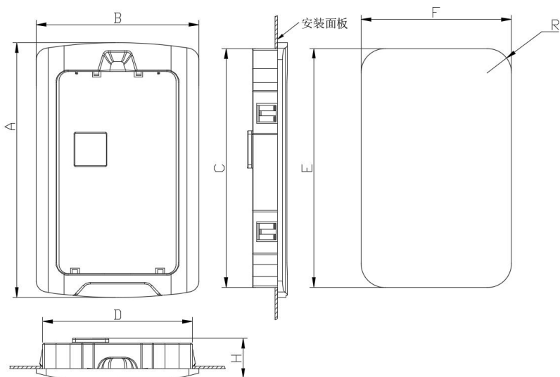
图 3-4 控制面板安装支架结构尺寸示意图
