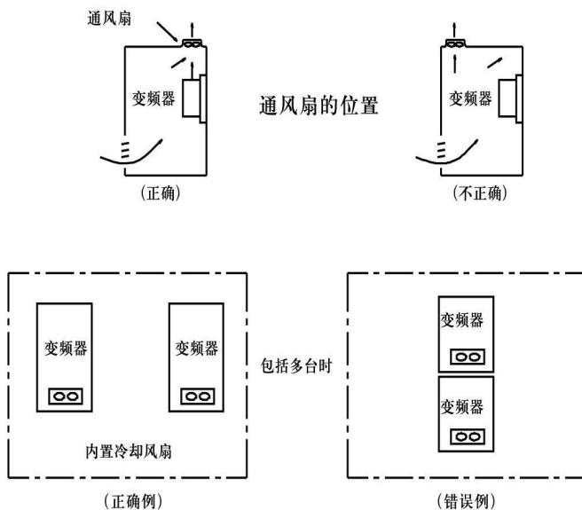
图 1-3 变频器安装在控制柜内示意图
