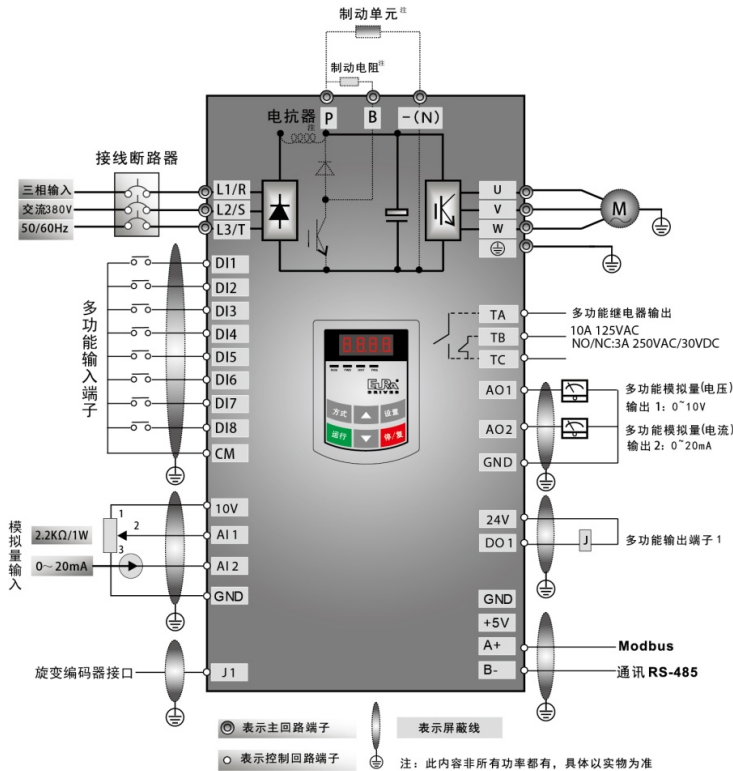
图 4-15 三相变频器标准配线图（NPN 方式）
