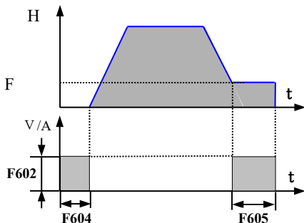
图 6-20 直流制动
