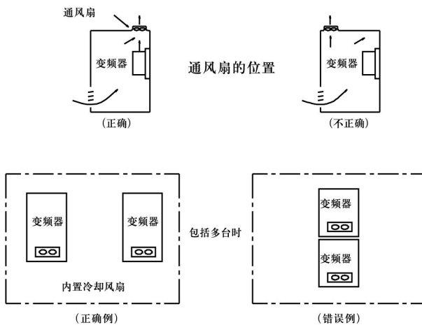
图 1-3 变频器安装在控制柜内示意图
