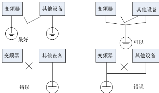
图 4-19 接地示意图
