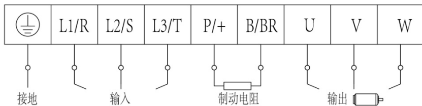
图 4-4 端子示意图
