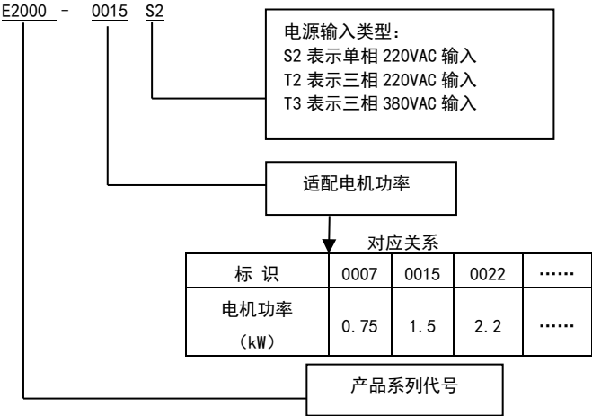
图 2-1 产品型号命名规则
