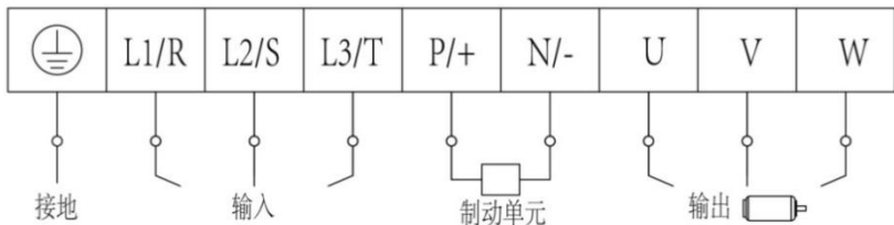
图 4-7 端子示意图
