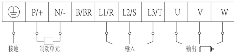
图 4-6 端子示意图
