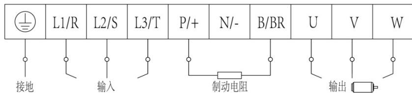
图 4-5 端子示意图
