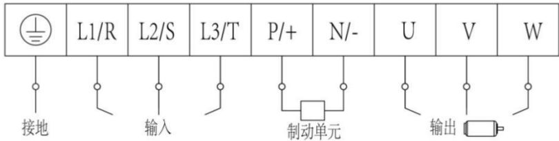
图 4-7 端子示意图
