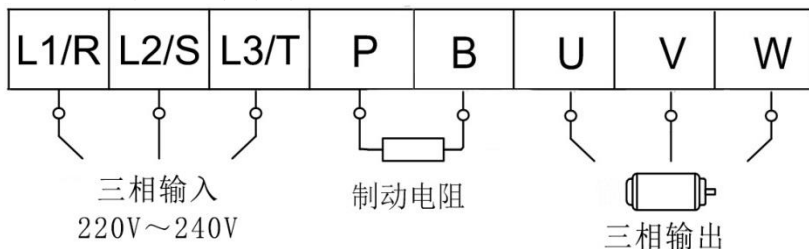
图 4-3 端子示意图
