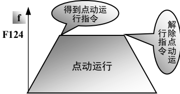
图 6-1 点动运行
