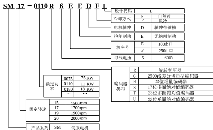
图 2.2.2 伺服电机命名规则（180 及 250 止口电机）
