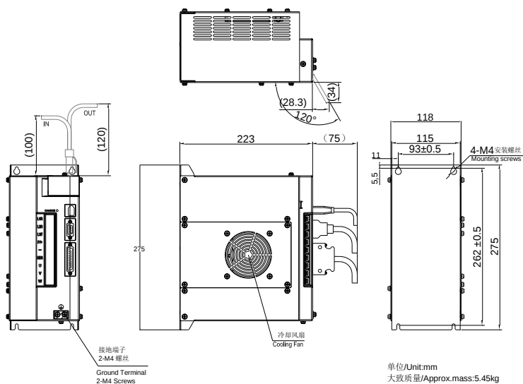
图 3.1.6 伺服驱动器结构尺寸 5
