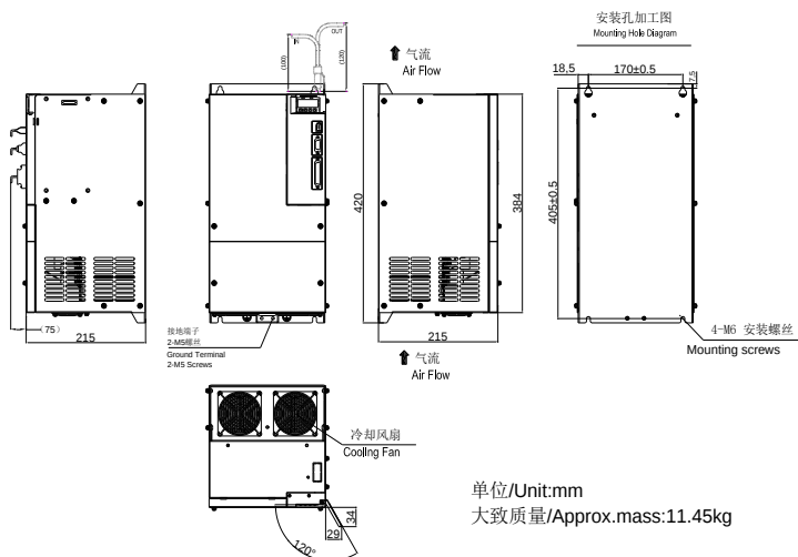
图 3.1.9 伺服驱动器结构尺寸 8
