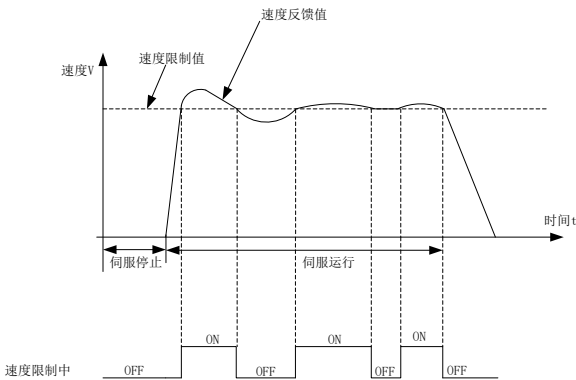
图 6.6.2 转矩模式下速度限制中输出示意图
