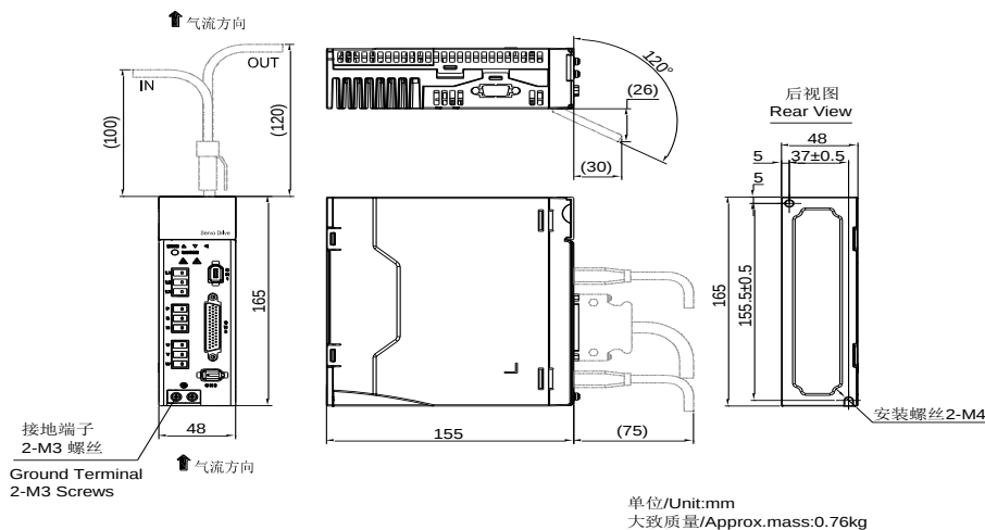
图 3.1.3 伺服驱动器结构尺寸 1
