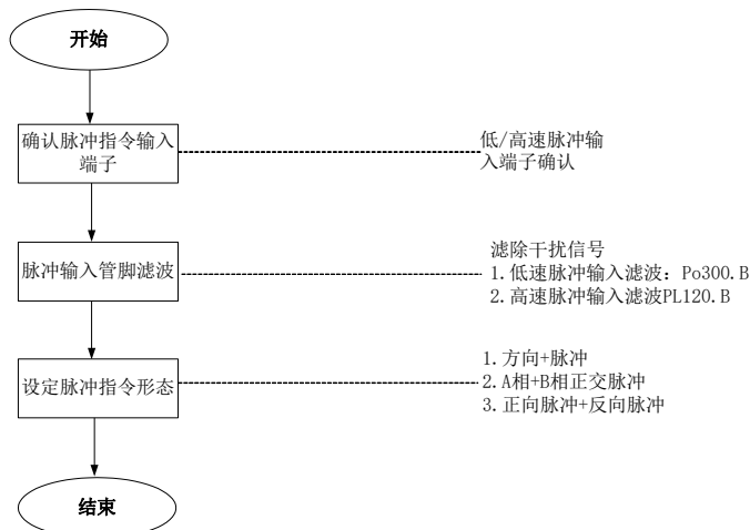
图 6.4.3 外部位置脉冲指令来源设置示意图
