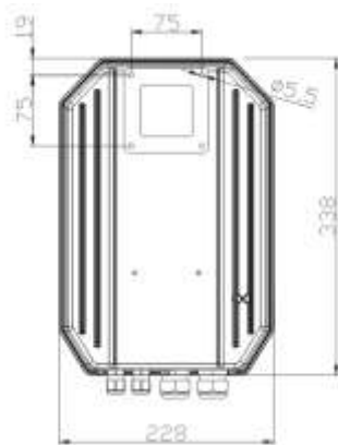
附图 3-5 驱动器 J2 与电机安装尺寸图
