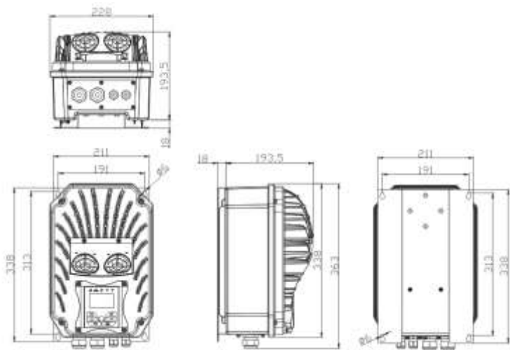
附图 3-4 驱动器 J2 壁挂尺寸图
