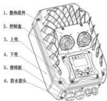
图 2-6 J2 壳产品外形及结构部件图
