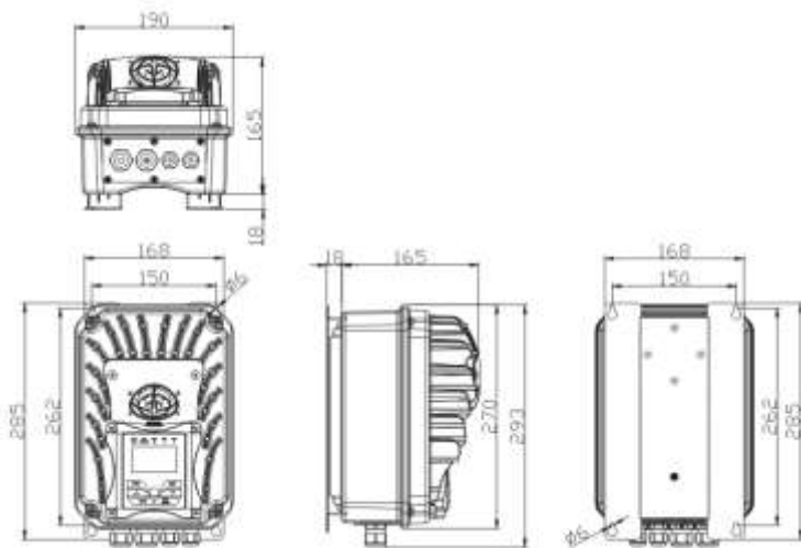
附图 3-2 驱动器 J1 壁挂尺寸图
