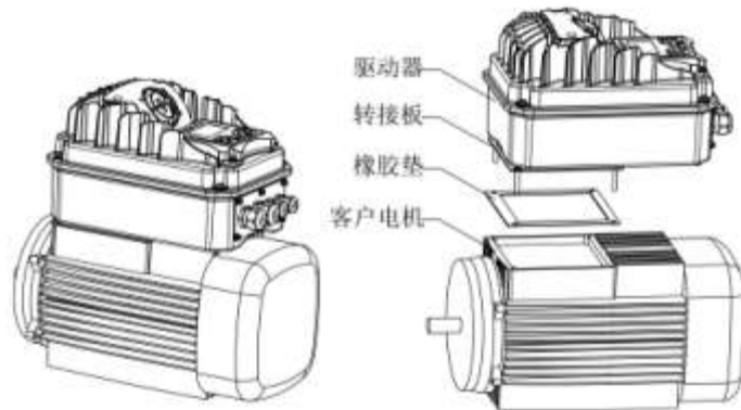
图 2-8 方案 2 电机转接板安装示意图
