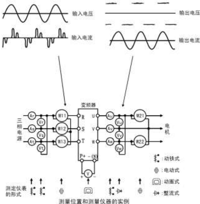
图 4-11 测量示意图
