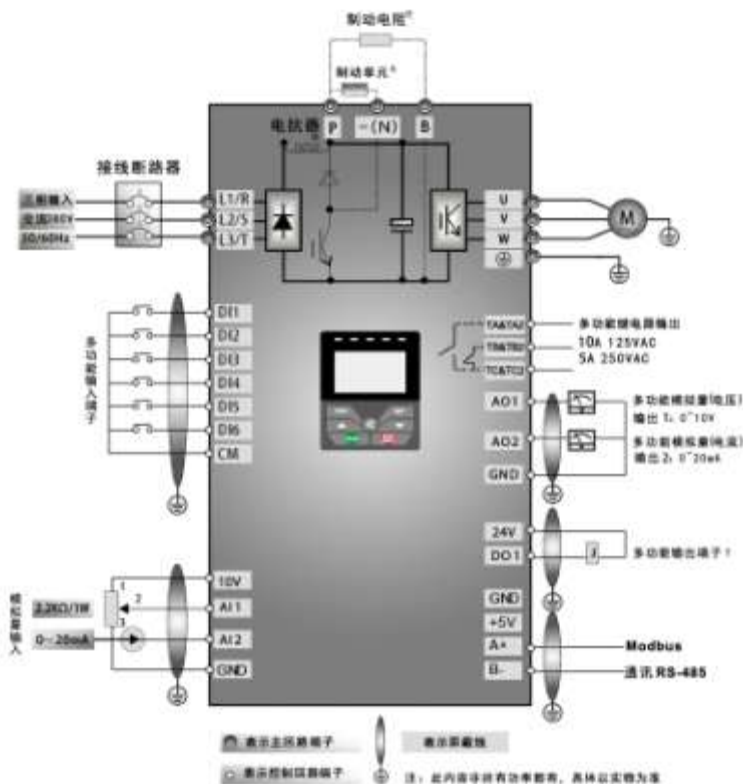
图 4-12 三相变频器标准配线图 (NPN 方式)
