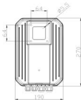
附图 3-3 驱动器 J1 与电机安装尺寸图
