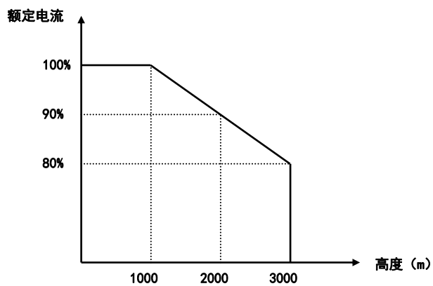
图 2-15 变频器额定电流与海拔高度降额曲线图
