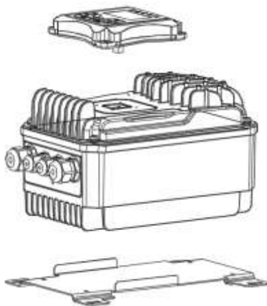
图 4-1-2 J0 变频器与壁挂板安装示意图
