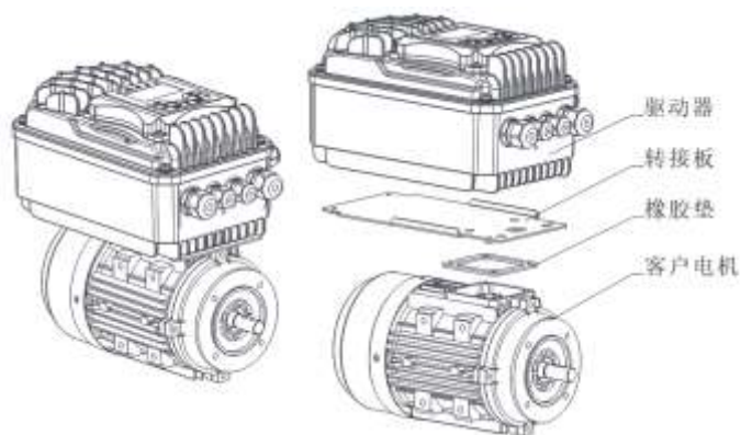
图 2-7 方案 2 电机转接板安装示意图
