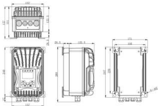
附图 3-1 驱动器 J0 壁挂尺寸图
