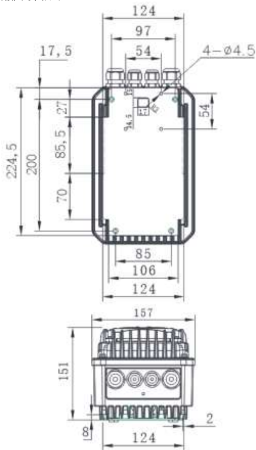
图 2-9 钣金转接板尺寸图
