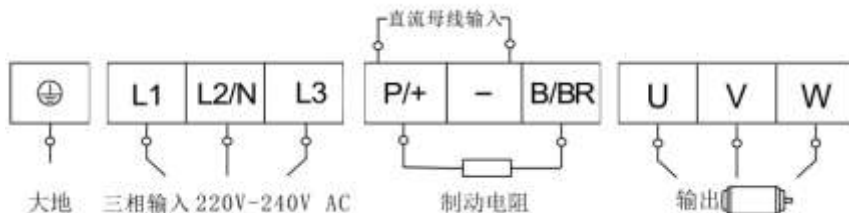
图 4-3 端子示意图
