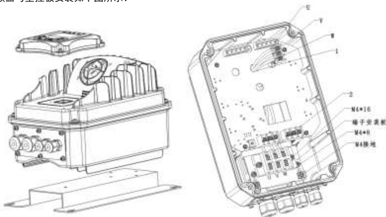
图 4-1-5 J1 变频器与壁挂板安装示意图
