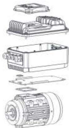
图 4-1-3 J0 变频器与电机安装示意图
