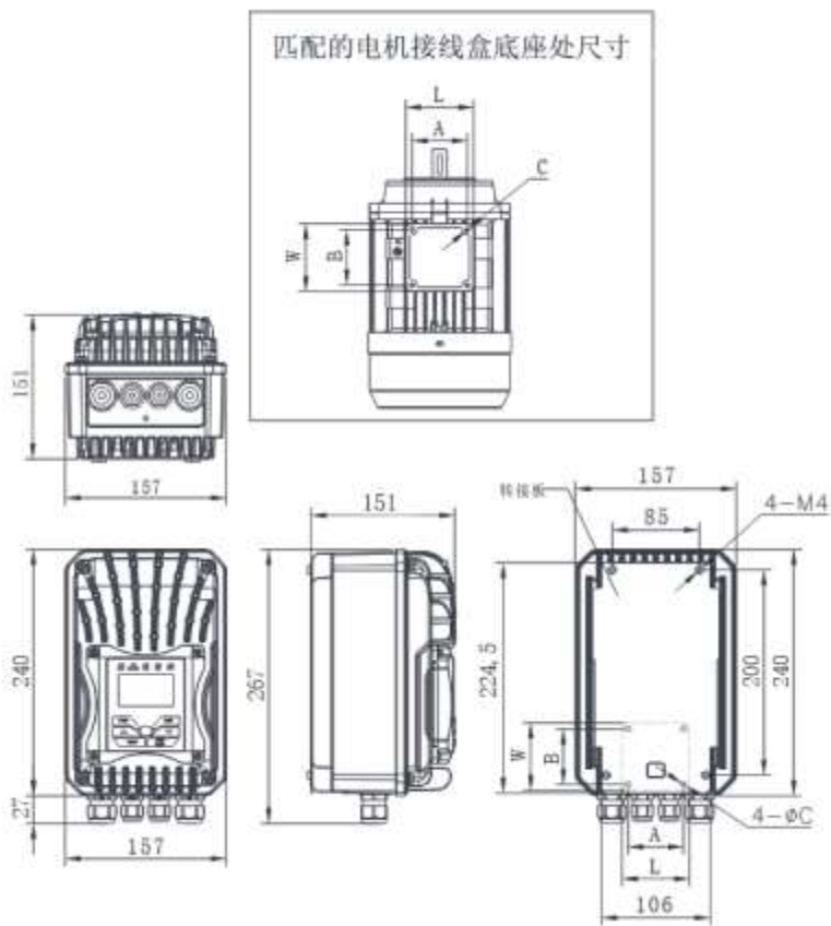
图 2-11 J0 驱动器与电机转接板尺寸图
