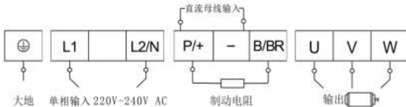
图 4-2 端子示意图
