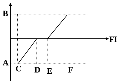
图 6-13 脉冲输入与设定量的计算关系
