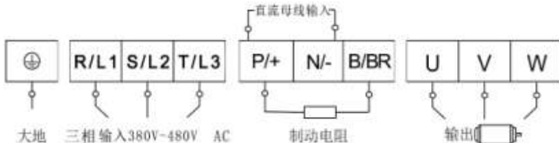
图 4-4 端子示意图
