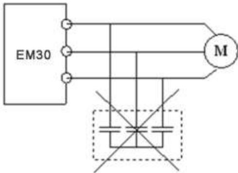
图 2-14 变频器输出端禁止使用电容器
