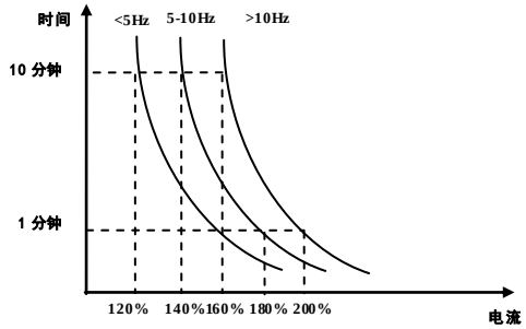
图 6-18 不同频率下的电机过载保护值
