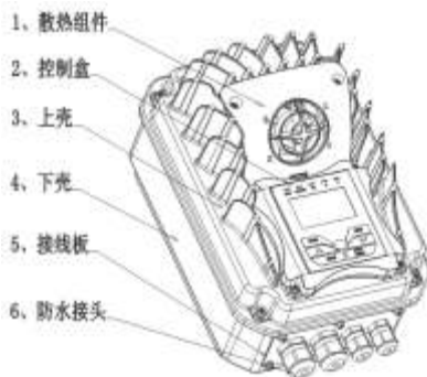
图 2-5 J1 壳产品外形及结构部件图
