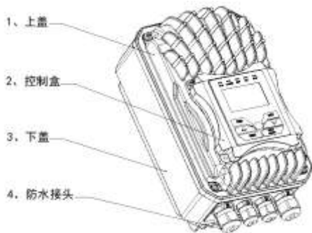
图 2-4 J0 壳产品外形及结构部件图
