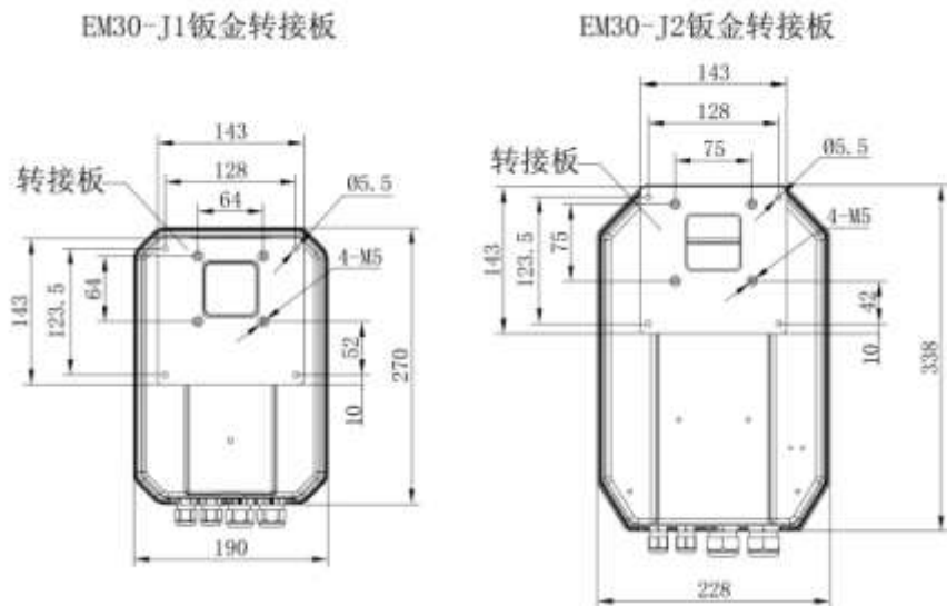
图 2-10 钣金转接板尺寸图
