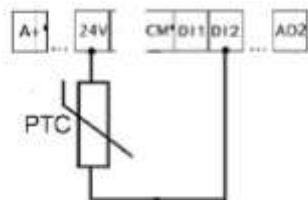
图 6-8 PTC 保护示意图
