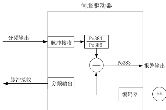
图 6.4.43 龙门同步实际使用中内部原理图
