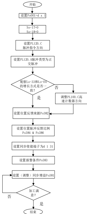
图 6. 4. 42 龙门同步功能设置流程图
