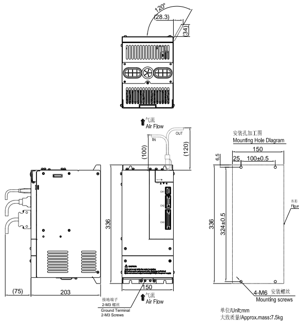
图 3.1.7 伺服驱动器结构尺寸 6
