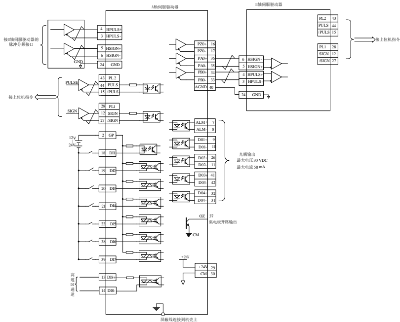
图 6.4.44 龙门同步典型接线图
