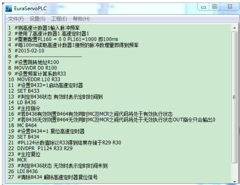
图 6.8.6 编译界面
