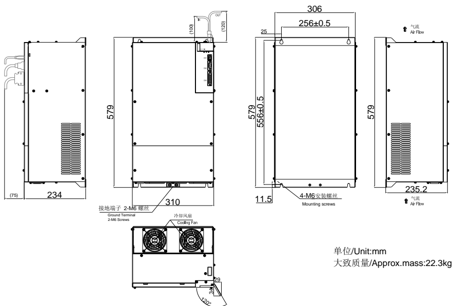
图 3.1.11 伺服驱动器结构尺寸 10
