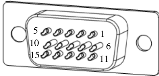
图 4.2.4 增量型编码器端子排列示意图
