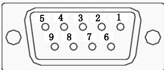
图 4.2.5 旋转变压器编码器端子排列示意图
