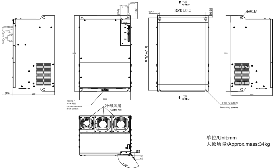
图 3.1.12 伺服驱动器结构尺寸 11
