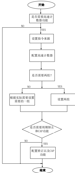
图 6.7.2 高速计数器设置流程
