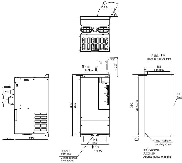
图 3.1.8 伺服驱动器结构尺寸 7
