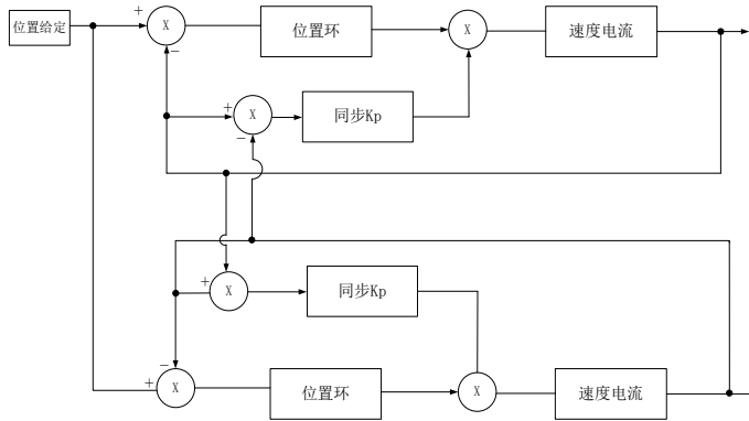
图 6. 4. 41 龙门同步典型应用接线图
