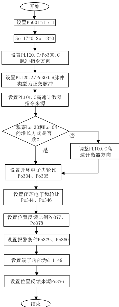
图 6. 4. 38 全闭环功能设置流程图
