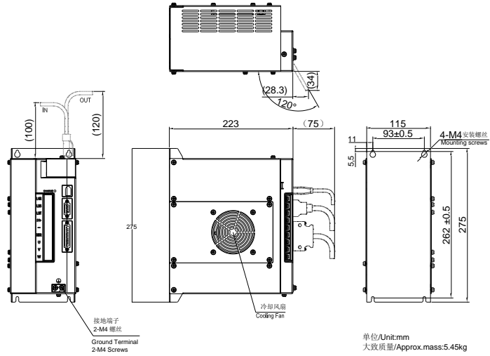
图 3.1.6 伺服驱动器结构尺寸 5
