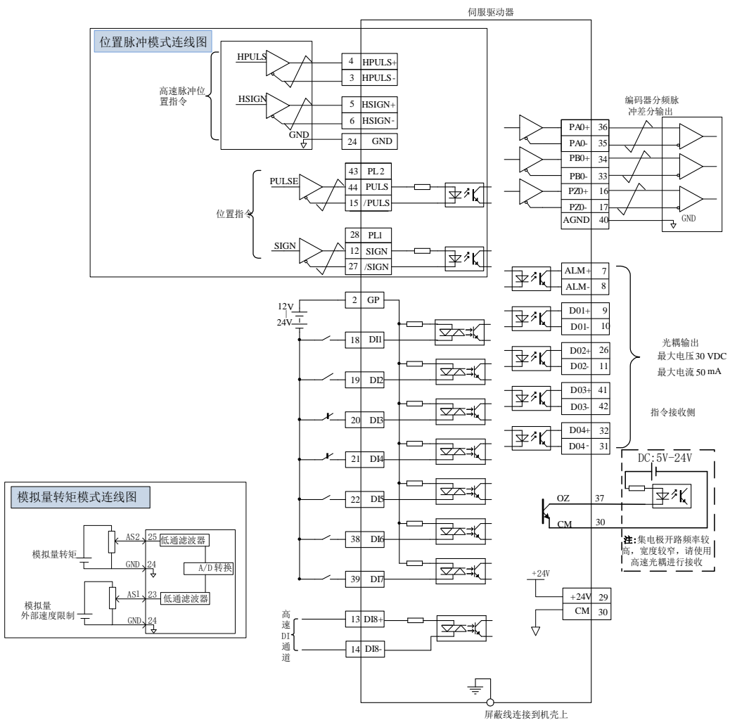
图 4.3.1 三种模式下接线示意图
