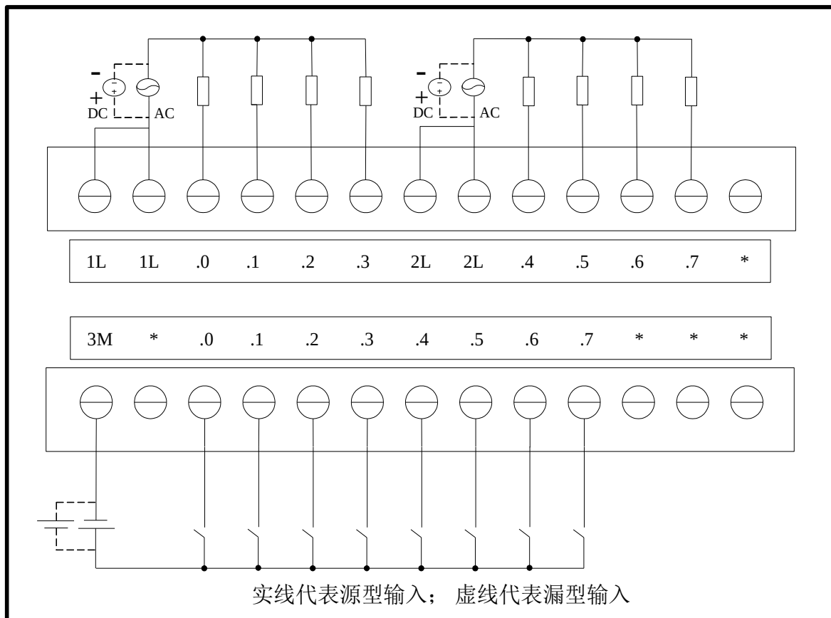
图 4-41 EC223-16DR 接线图
