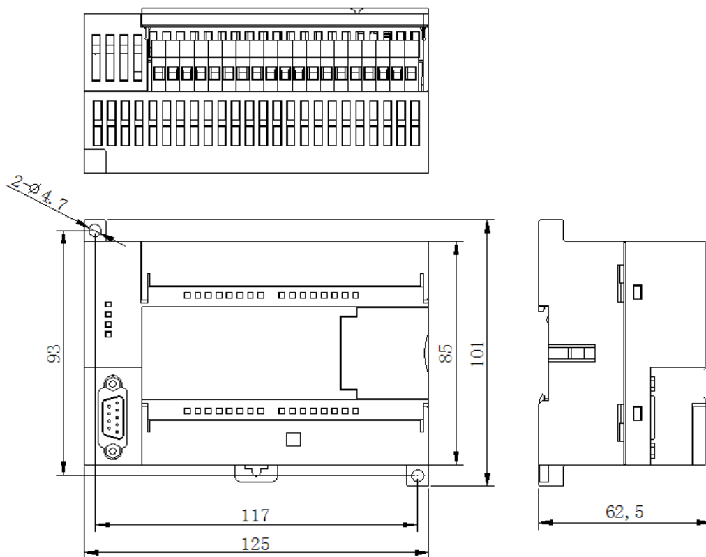
图 2-7 P4 外形尺寸及安装图
