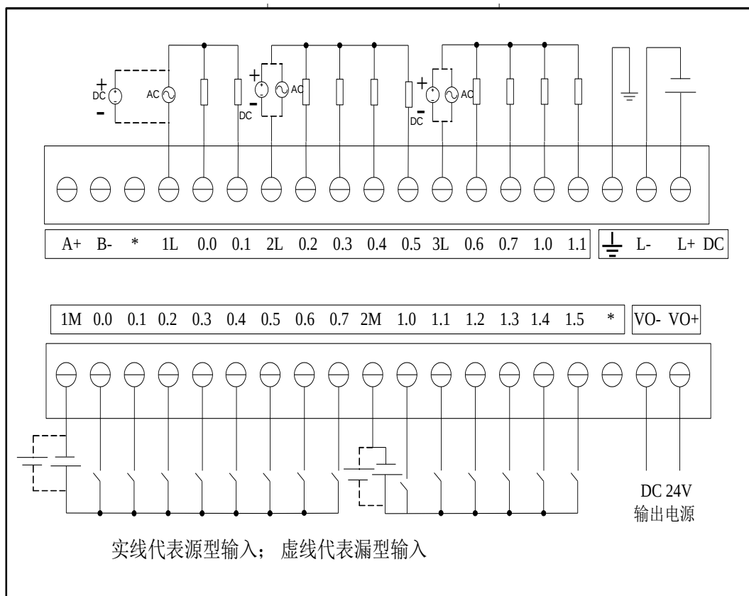
图 3-13 EC204-24DR 接线图
