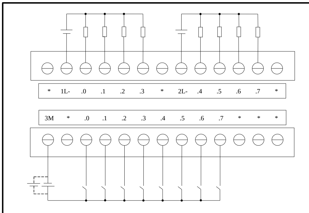
图 4-36 EC223-16DTD 接线图
