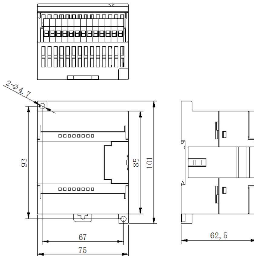
图 2-5 P2 外形尺寸及安装图
