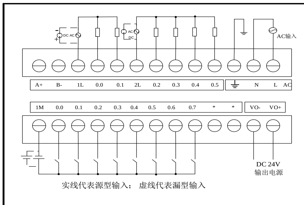
图 3-8 EC202-14AR 接线图
