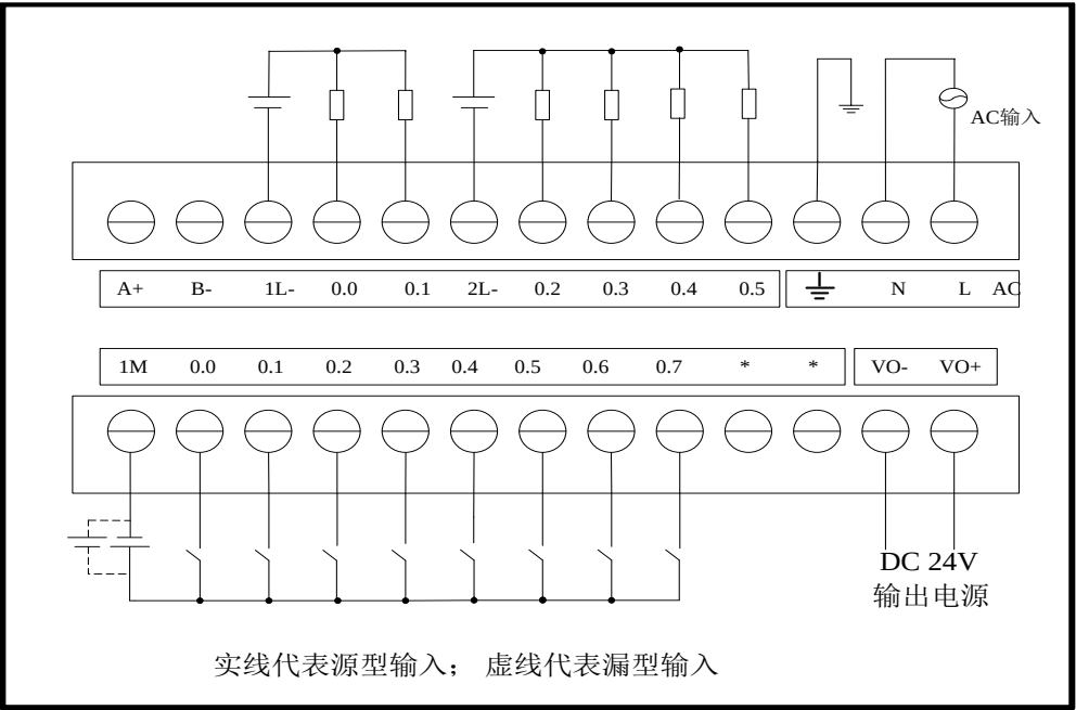
图 3-6 EC202-14ATD 接线图
