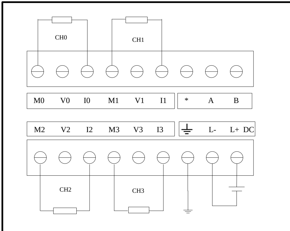
图 5-15 EC232-04IVM 电流接线图
