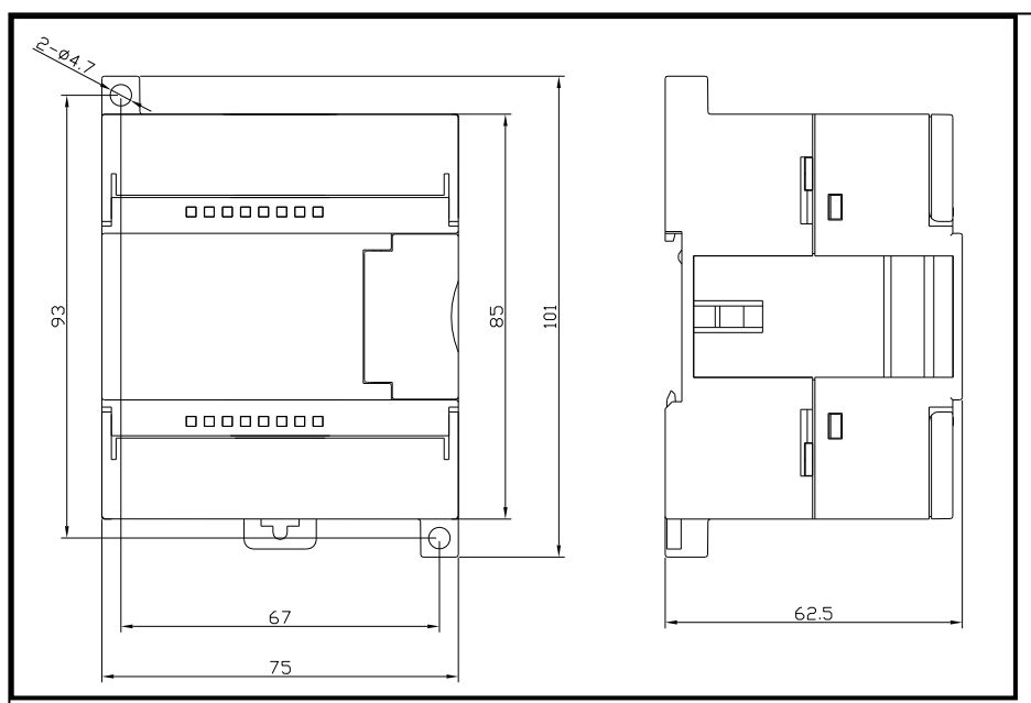
图 4-20 EC222-16DTD 安装尺寸图
