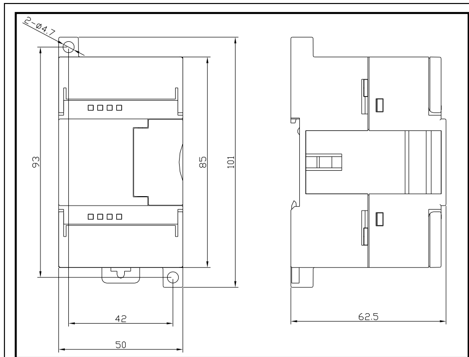
图 5-21 EC233-04IVM 安装原理图
