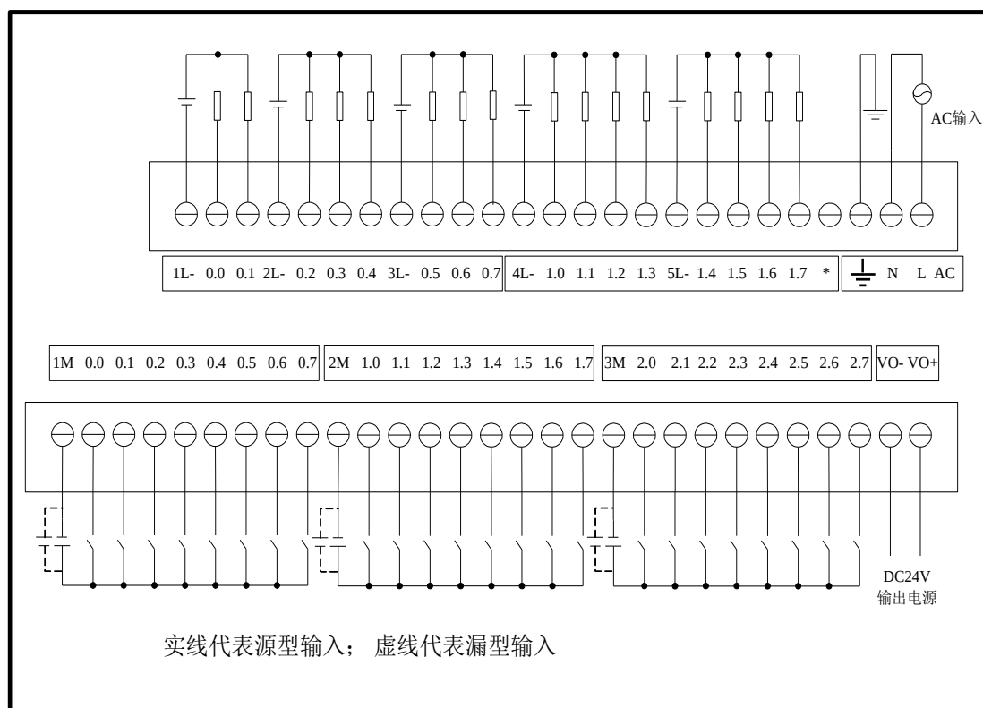
图 3-14 EC206-40ATD 接线图
