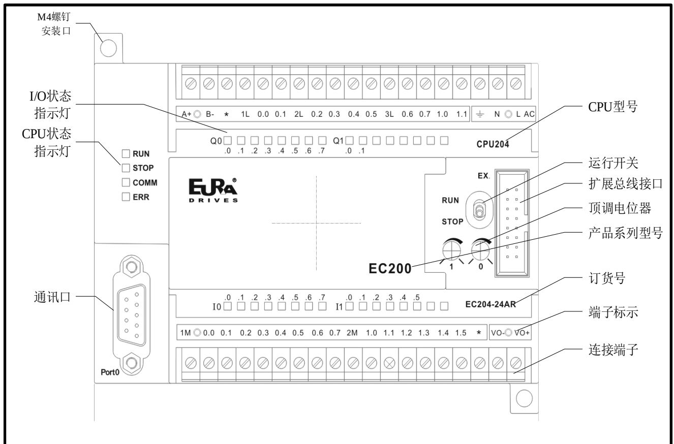
图 3-1 EC204-24AR 前面板视图
