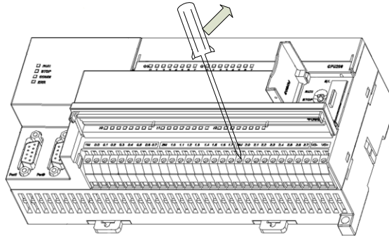
图 2-9 可插拔端子的拆卸示意图
