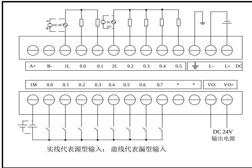
图 3-9 EC202-14DR 接线图
