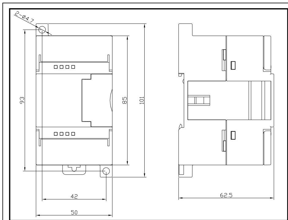
图 4-29 EC223-08DTD 安装尺寸图
