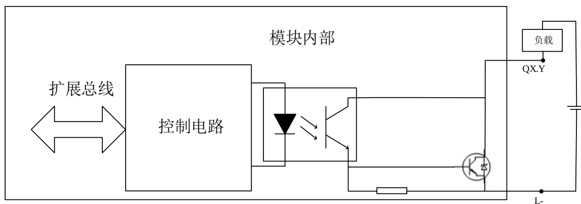
图 4-28 DO 漏型电气原理图
