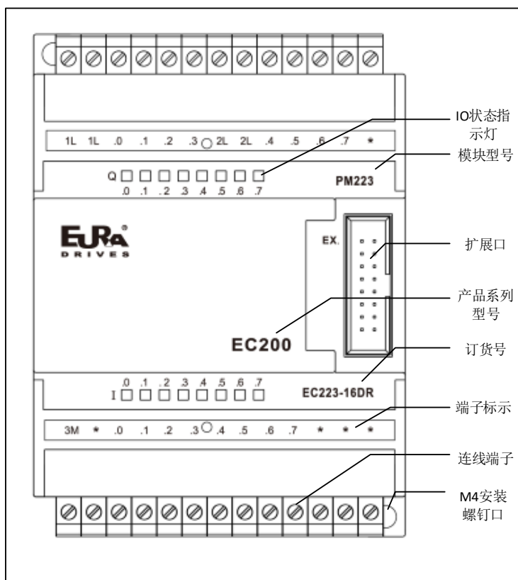
图 4-40 EC223-16DR 前面板图
