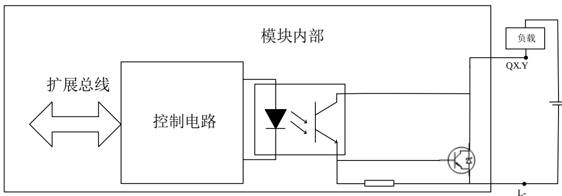
图 4-11 DO 漏型电气原理图
