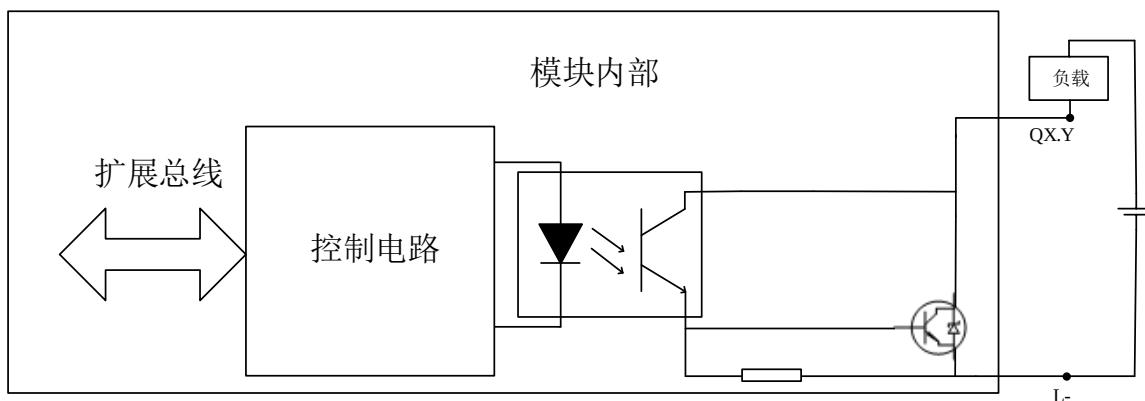
图 4-19 DO 漏型电气原理图
