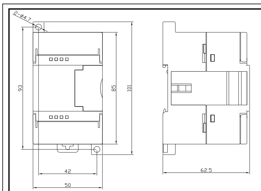
图 4-4 EC221-08DX 安装尺寸图
