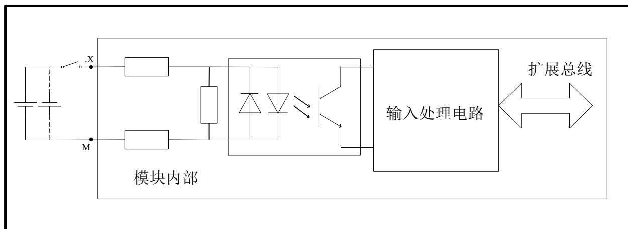
图 4-37 DI 电气原理图
