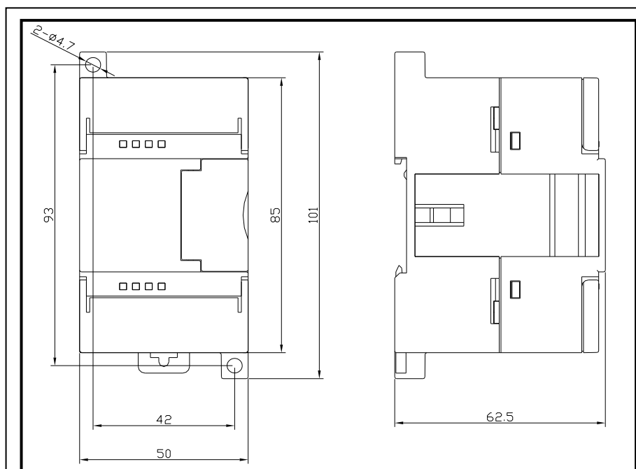
图 5-5 EC231-04IVM 安装尺寸图
