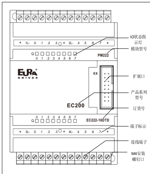
图 4-17 EC222-16DTD 前面板图
