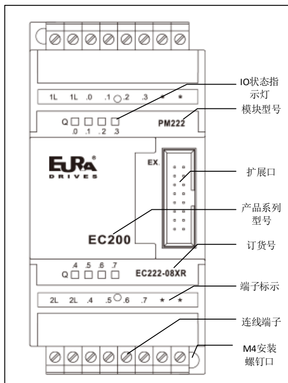
图 4-13 EC222-08XR 前面板示意图
