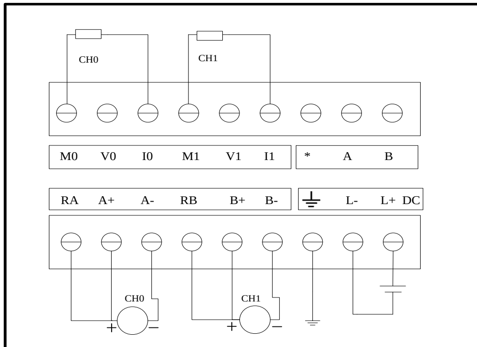
图 5-19 EC233-04IVM 电流模式接线图
