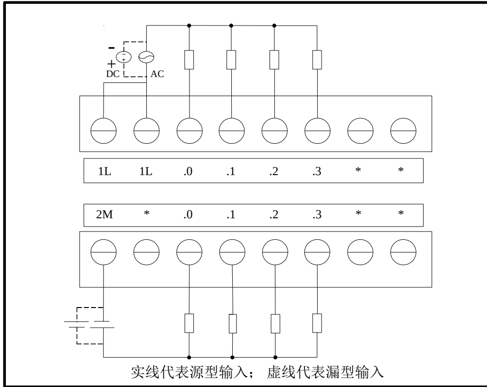
图 4-31 EC223-08DR 接线图
