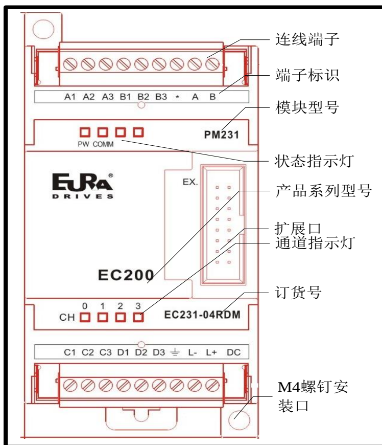
图 5-6 EC231-04RDM 前面板图
