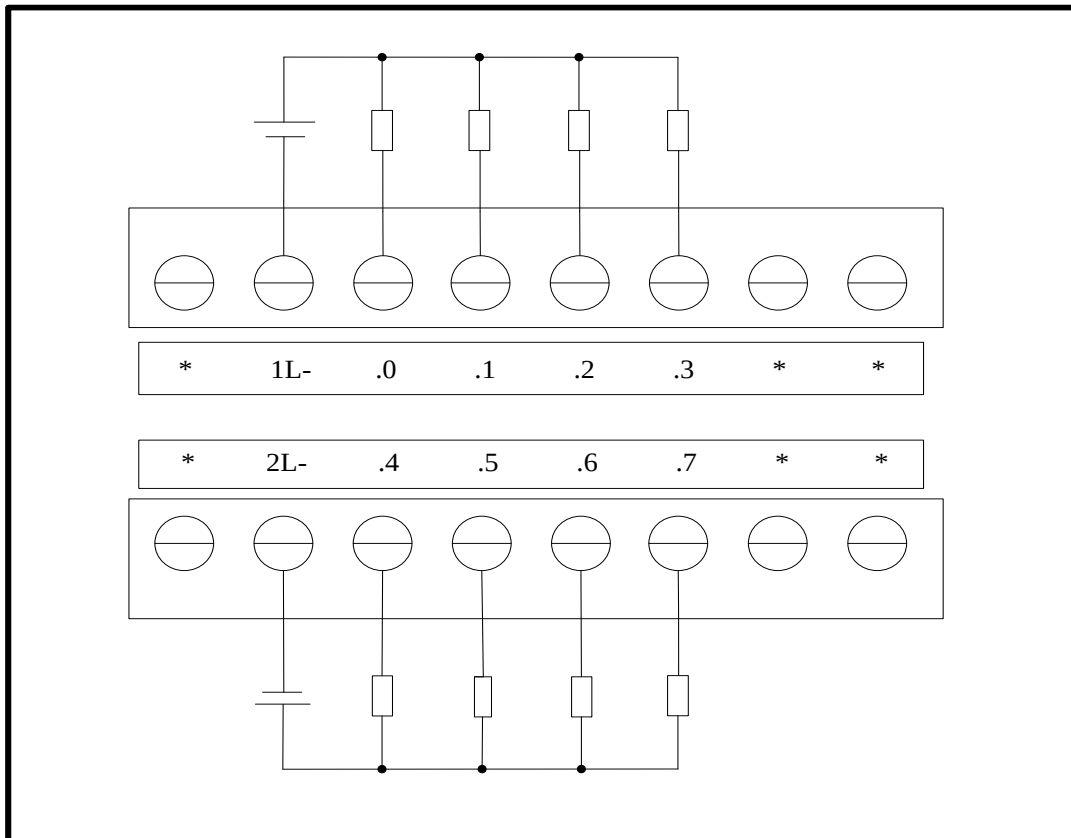
图 4-10 EC222-08DTD 接线图
