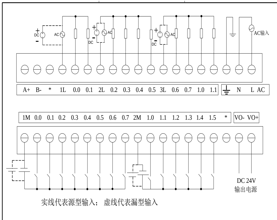
图 3-12 EC204-24AR 接线图
