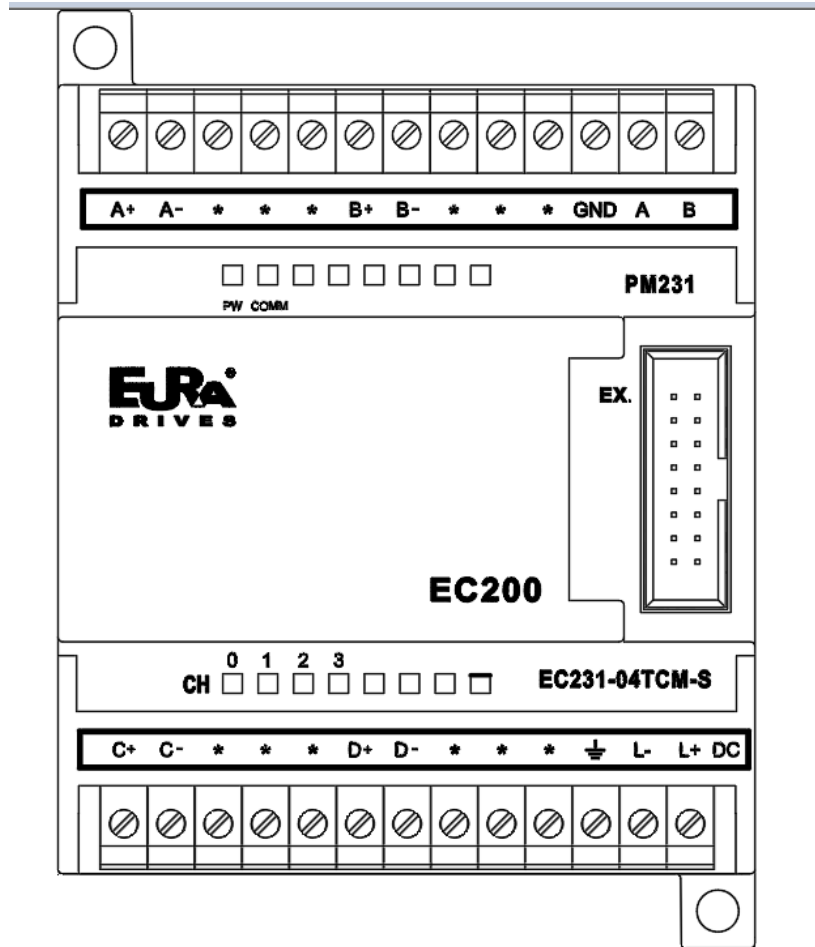
图 5-10 EC231-04TCM-S 前面板图
