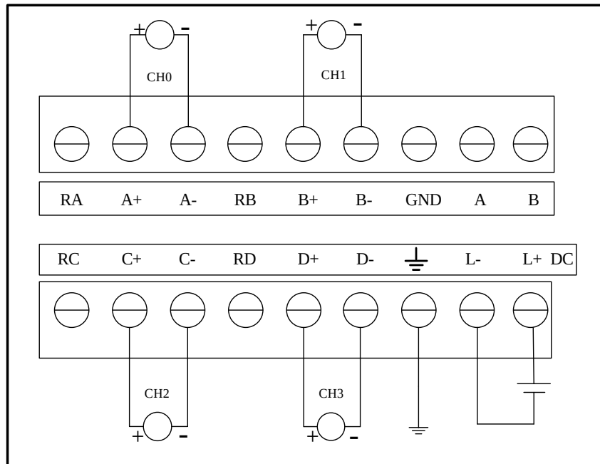
图 5-2 EC231-04IVM 接线图：电压信号
