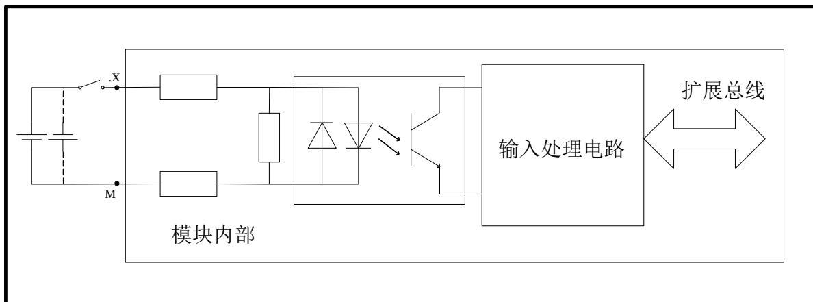
图 4-27 DI 电气原理图
