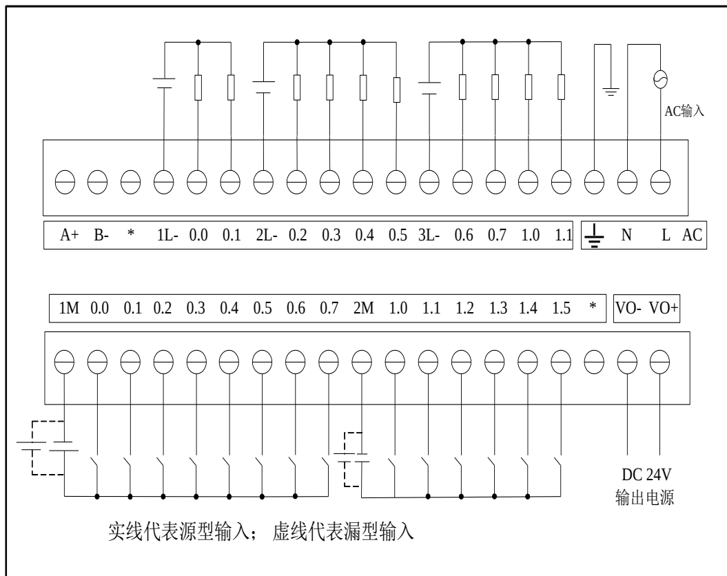
图 3-10 EC204-24ATD 接线图
