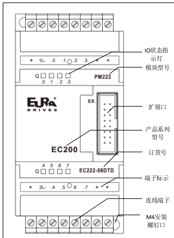
图 4-9 EC222-08DTD 前面板图
