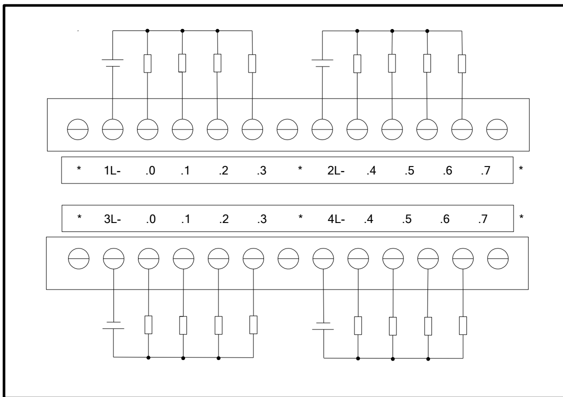
图 4-18 EC222-16DTD 接线图
