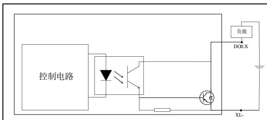
图 3-4 DO 输出通道电气原理图
