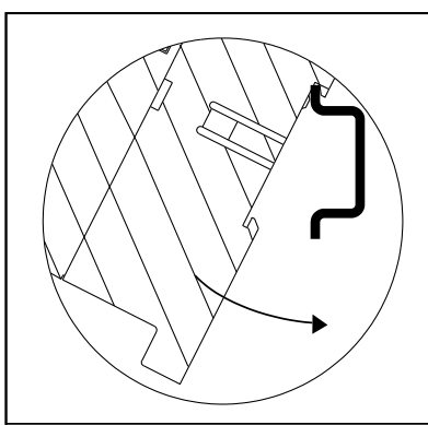
图 2-3 安装示意图
