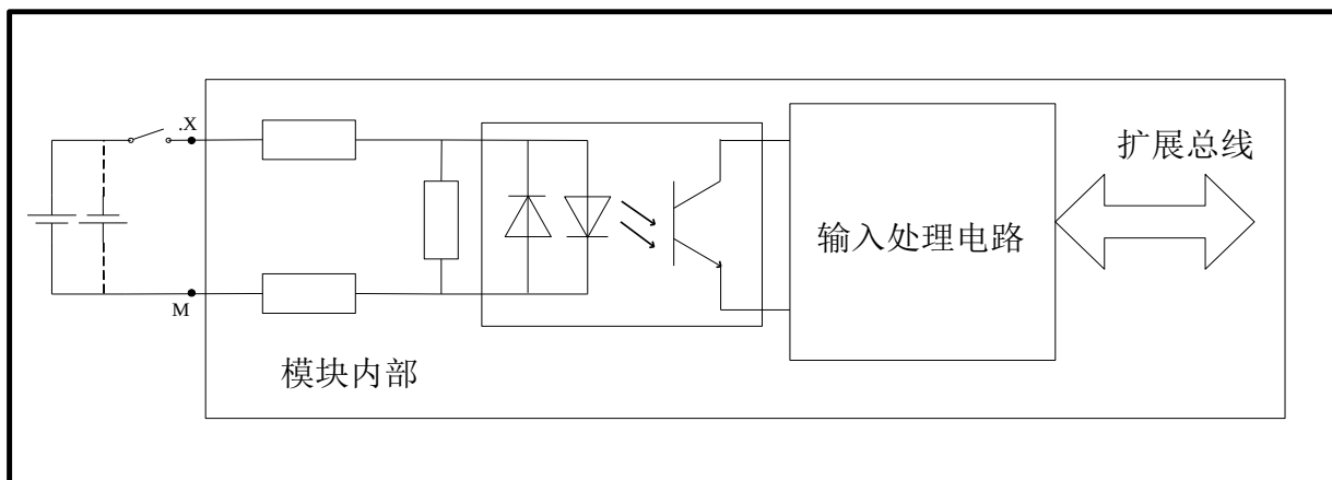
图 4-47 DI 电气原理图
