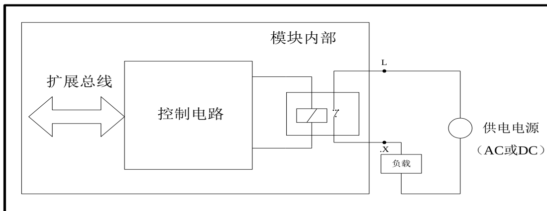
图 4-43 DO 电气原理图
