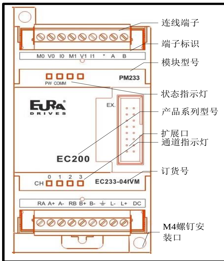
图 5-17 EC233-04IVM 前面板图
