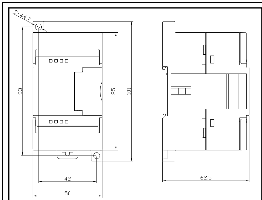
图 5-16 EC232-04IVM 安装尺寸图
