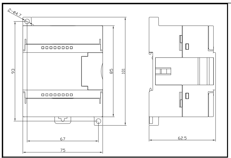
图 4-8 EC221-16DX 安装尺寸图
