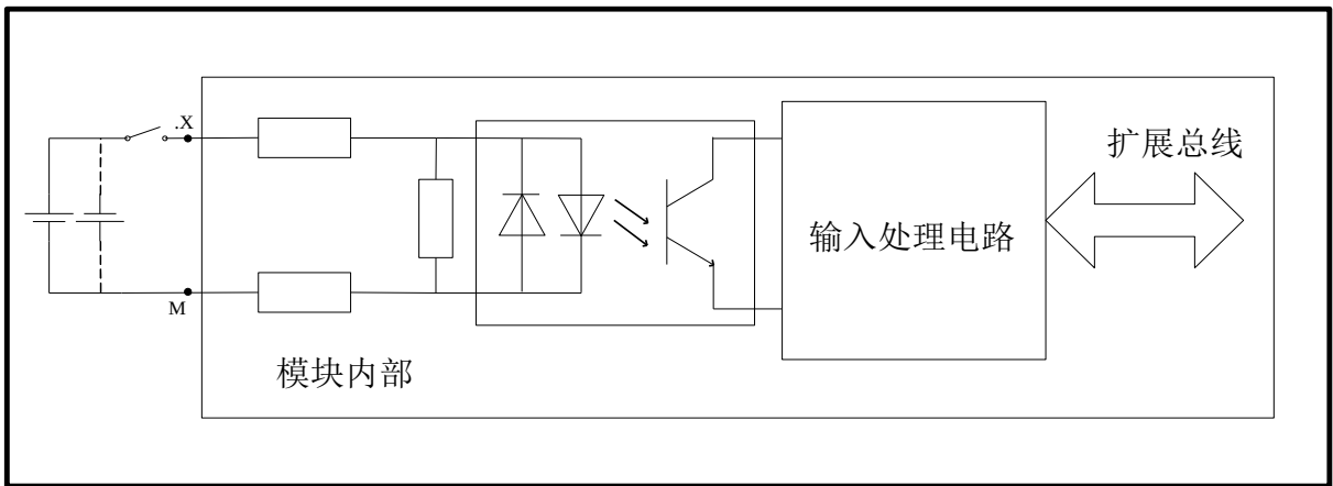
图 4-32 DI 电气原理图
