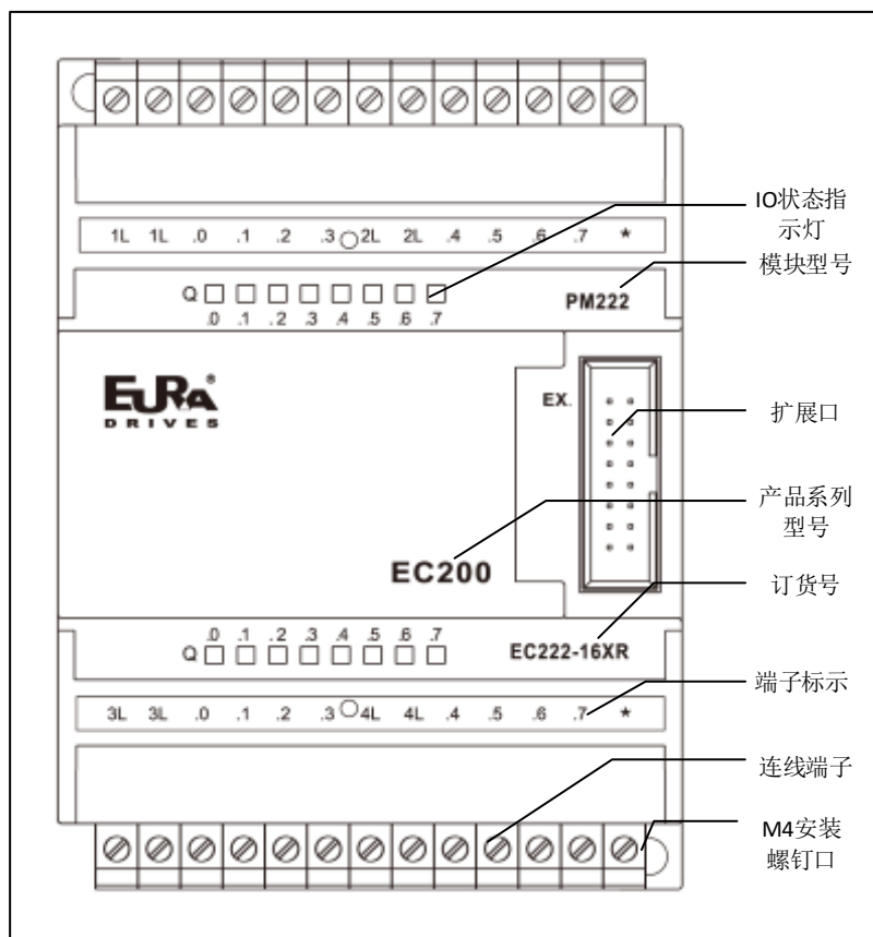
图 4-21 EC222-16XR 前面板图
