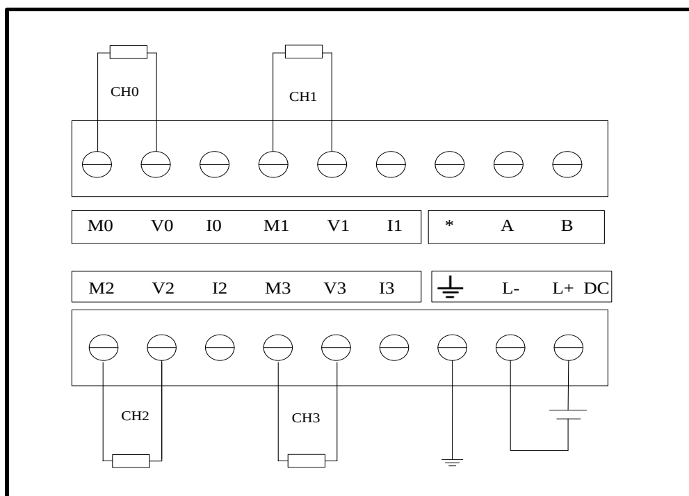
图 5-14 EC232-04IVM 电压接线图
