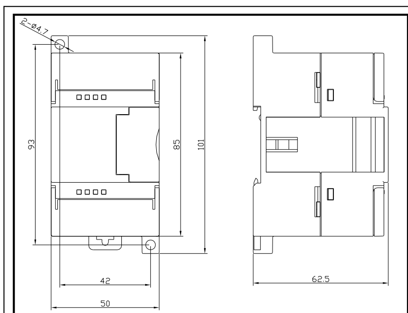
图 4-16 EC222-08XR 安装尺寸图
