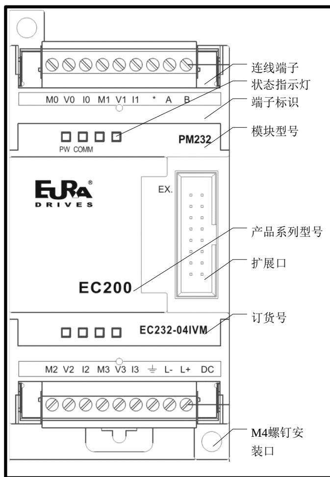
图 5-13 EC232-04IVM 前面板图
