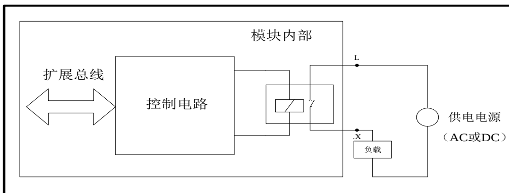
图 4-15 EC222-08XR 电气原理图
