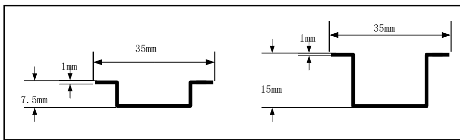
图 2-2 DIN 导轨示意图
