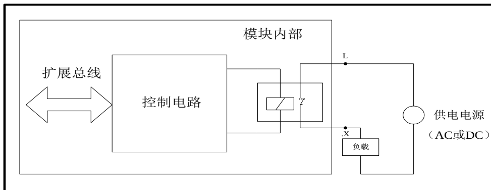
图 4-33 DO 电气原理图
