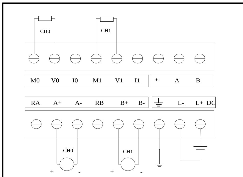
图 5-18 EC233-04IVM 电压模式接线图
