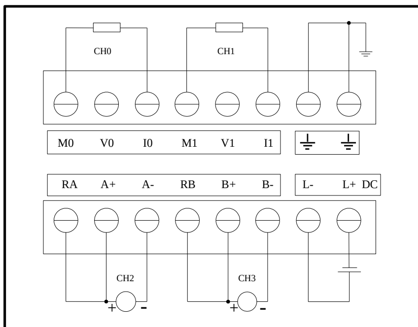
图 5-20 EC233-04IVM 电流四线制接线图
