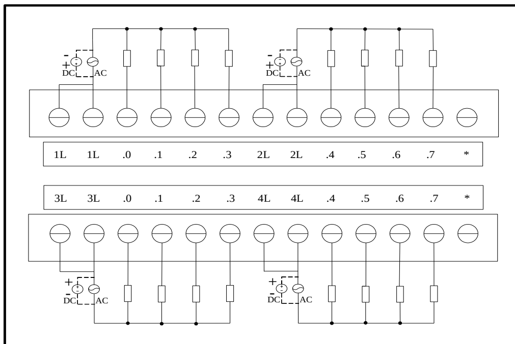
图 4-22 EC222-16XR 接线图
