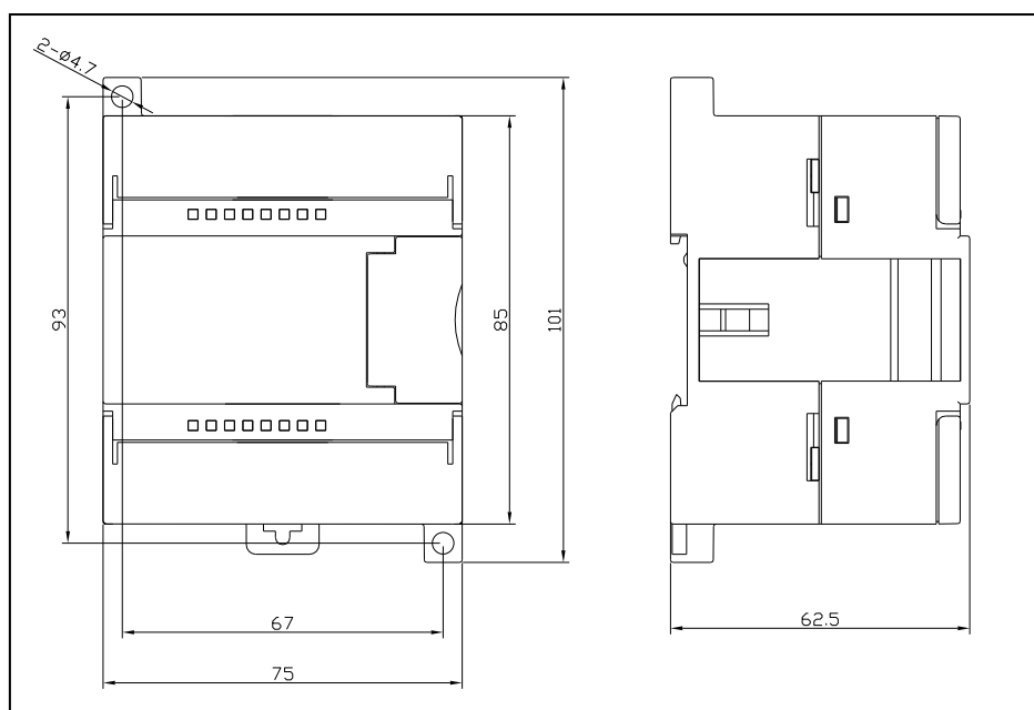
图 5-12 EC231-04TCM-S 安装尺寸图
