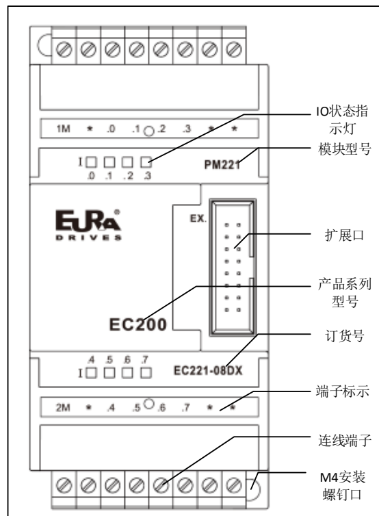
图 4-1 EC221-08DX 前面板图
