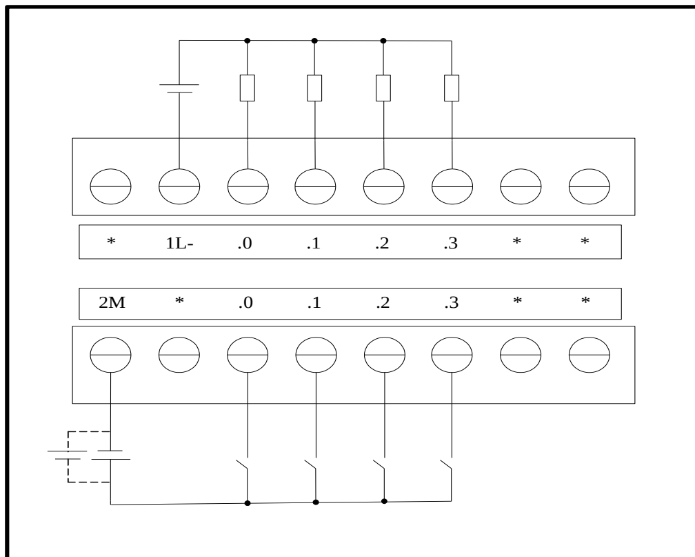
图 4-26 EC223-08DTD 接线图
