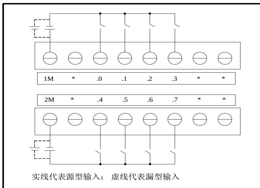
图 4-2 EC221-08DX 接线图
