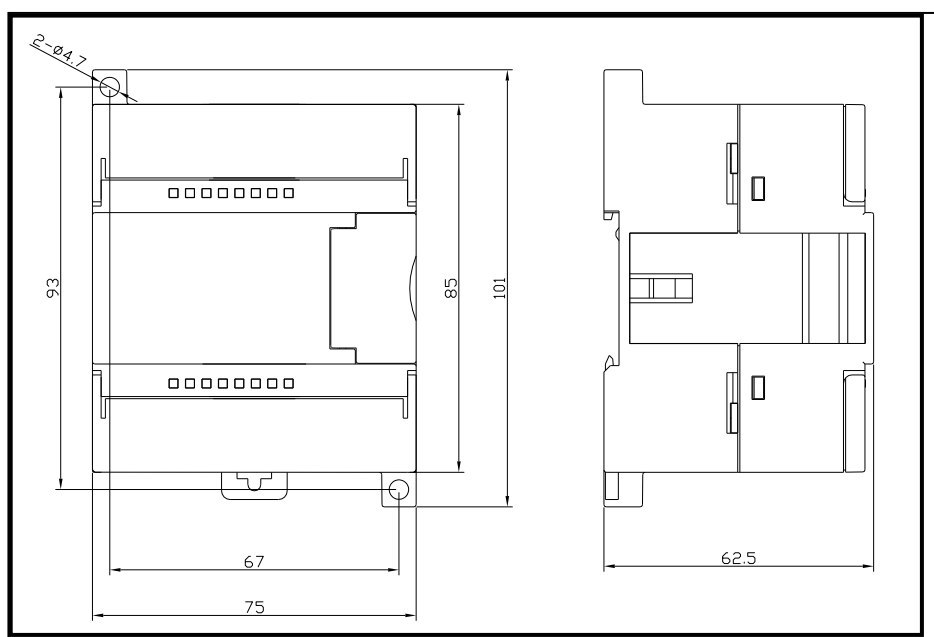
图 4-44 EC223-16DR 安装尺寸图
