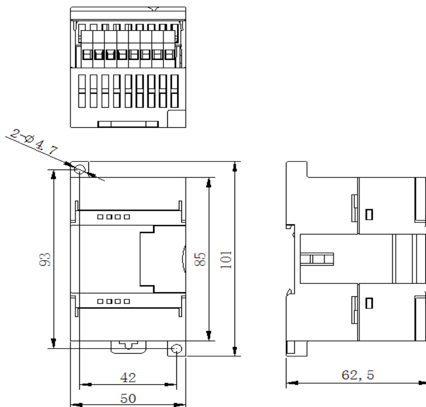
图 2-4 P1 外形尺寸及安装图
