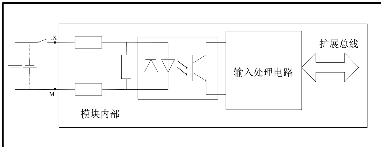
图 4-7 EC221-16DX 电气原理图
