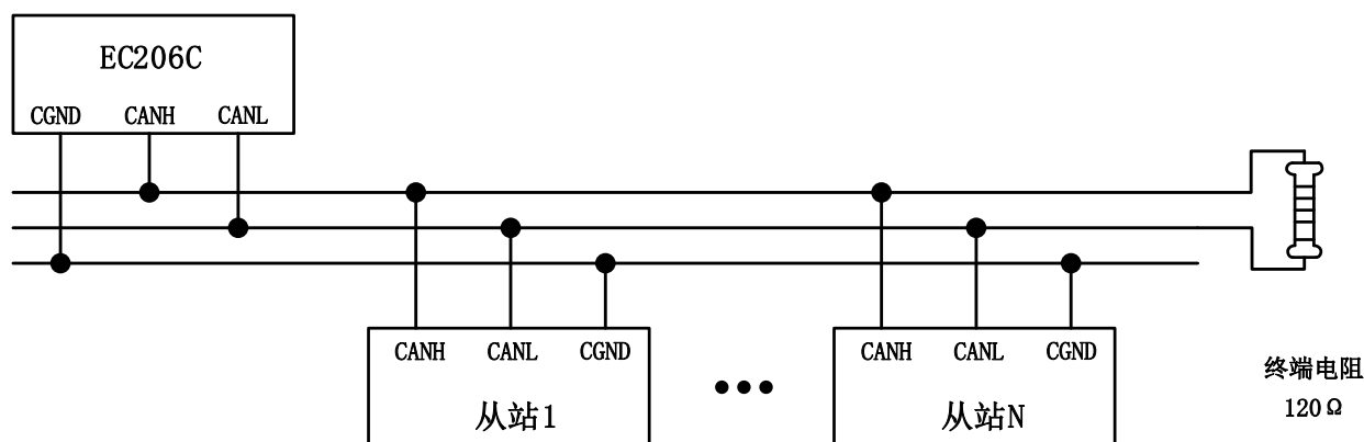
图 3-3 CANopen 总线连接示意图
