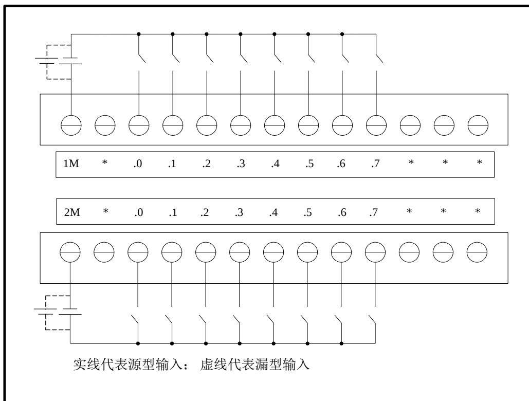
图 4-6 EC221-16DX 接线图
