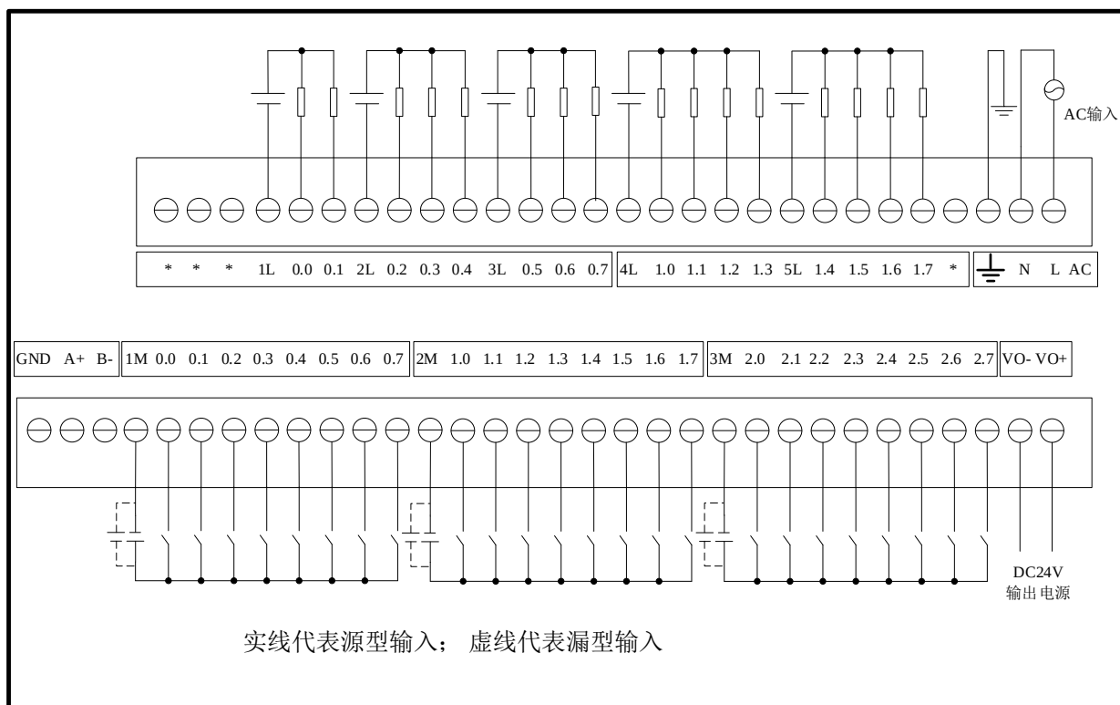
图 3-19 EC206E-40ATD 接线图
