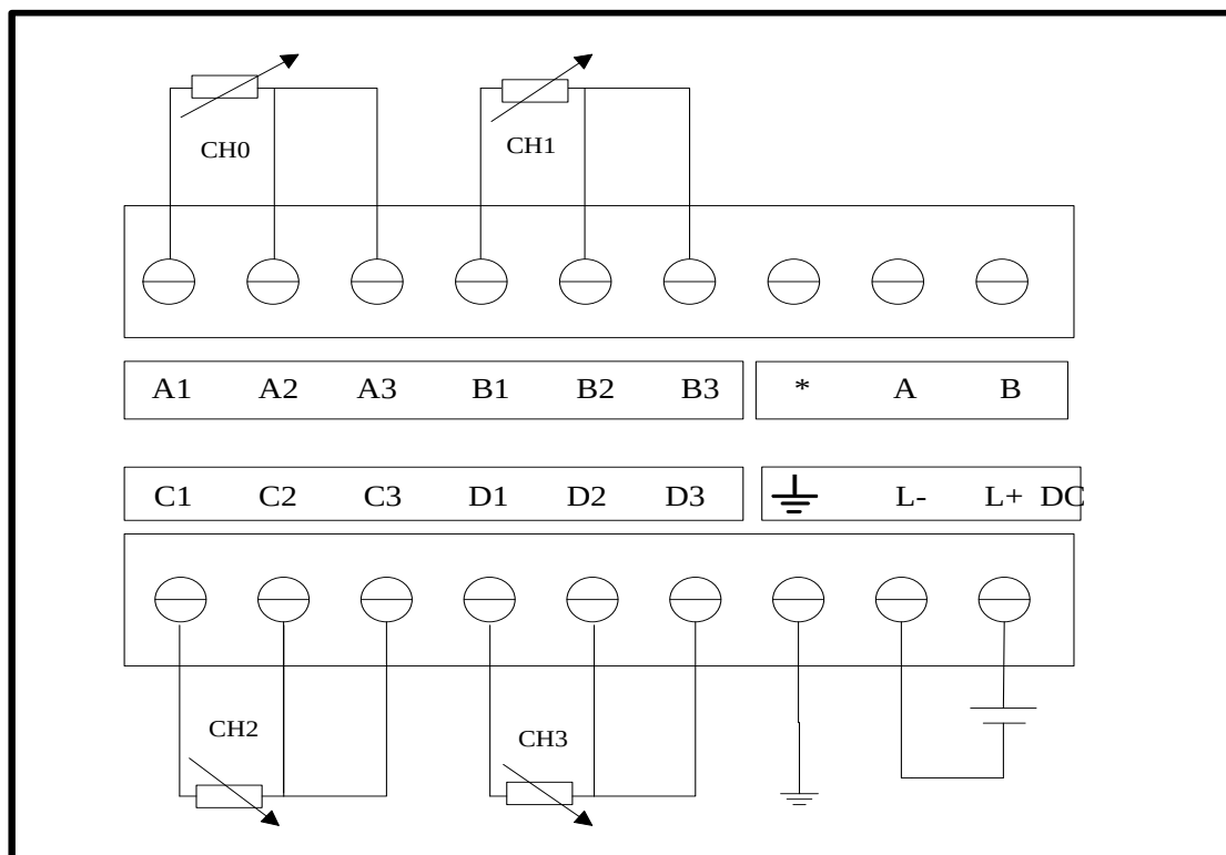
图 5-8 EC231-04RDM 三线制接线图
