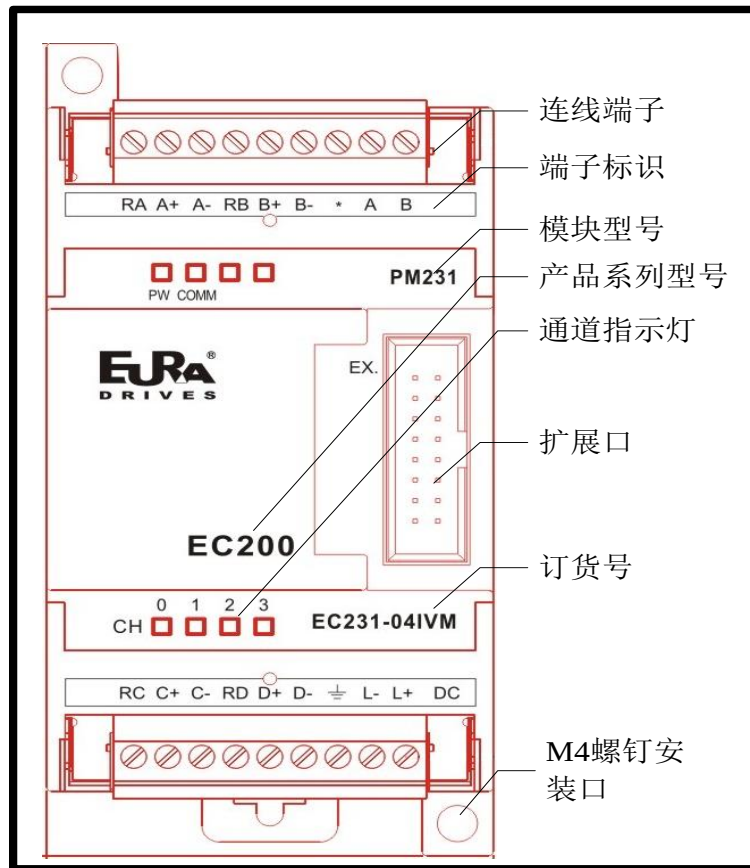
图 5-1 EC231-04IVM 前面板图
