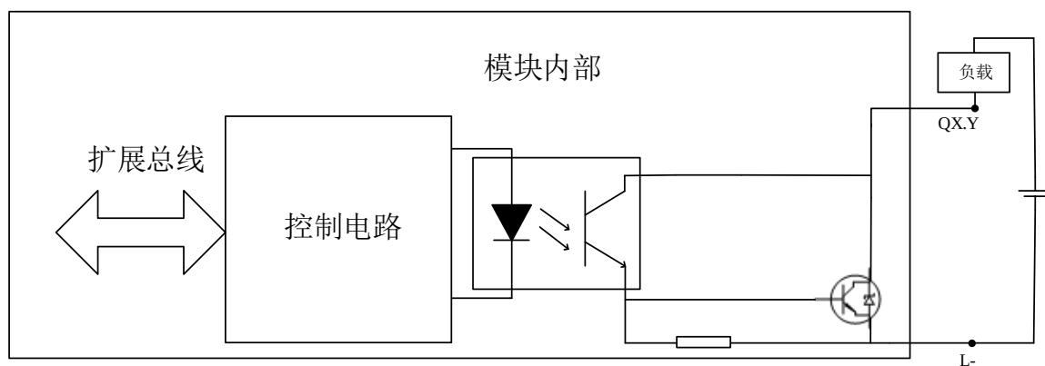
图 4-48 DO 漏型电气原理图
