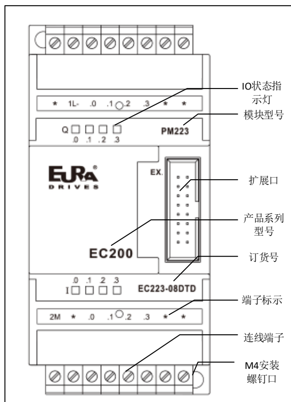
图 4-25 EC223-08DTD 前面板图
