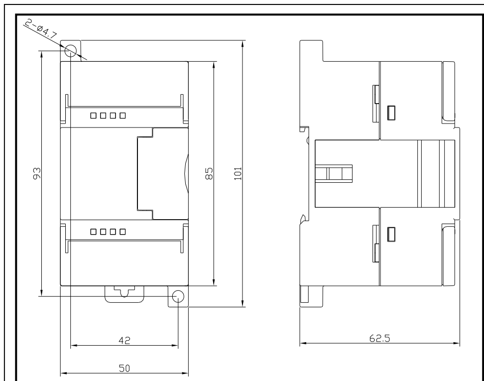
图 5-9 EC231-04RDM 安装尺寸图
