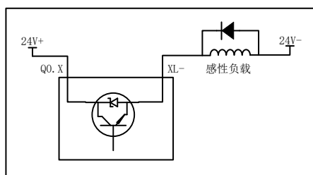
图 3-5 感性负载接线图
