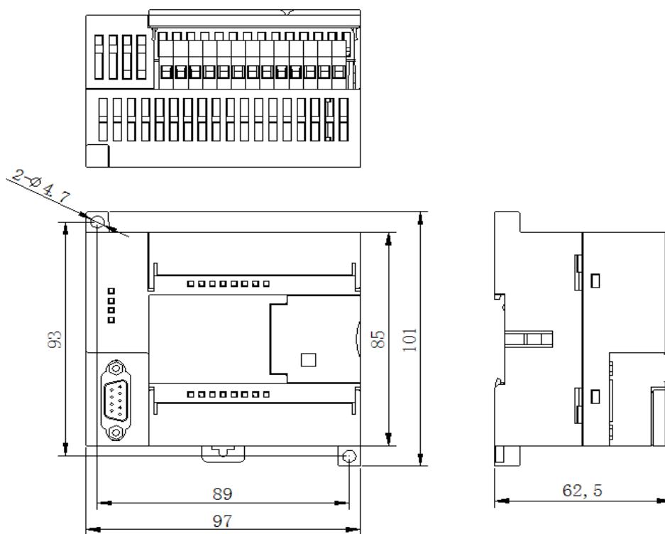
图 2-6 P3 外形尺寸及安装图
