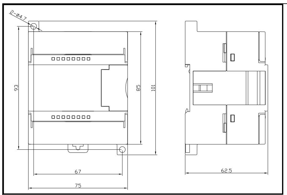
图 4-24 EC222-16XR 安装尺寸图
