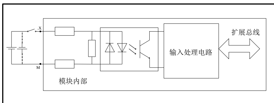
图 4-3 EC221-08DX 电气原理图
