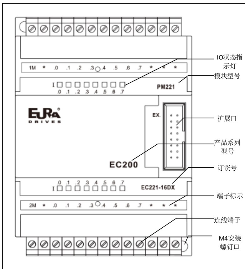
图 4-5 EC221-16DX 前面板图
