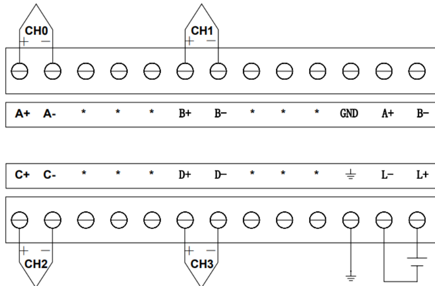
图 5-11 EC231-04TCM-S 端子接线图
