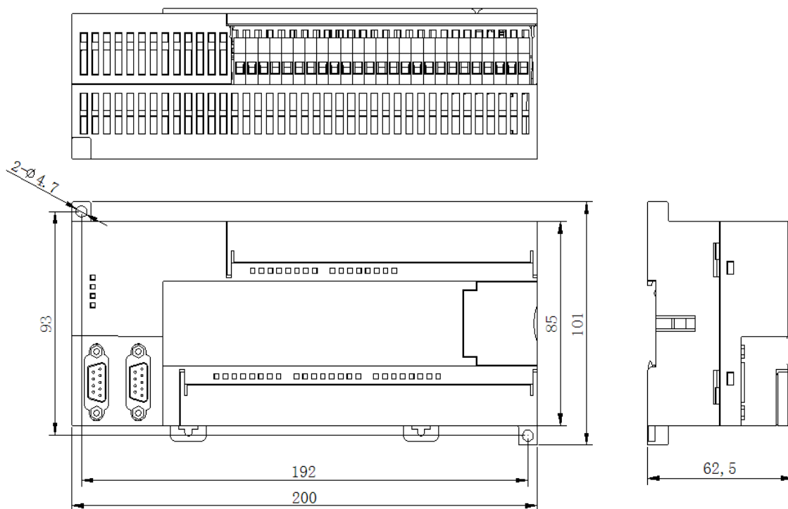
图 2-8 P5 外形尺寸及安装图
