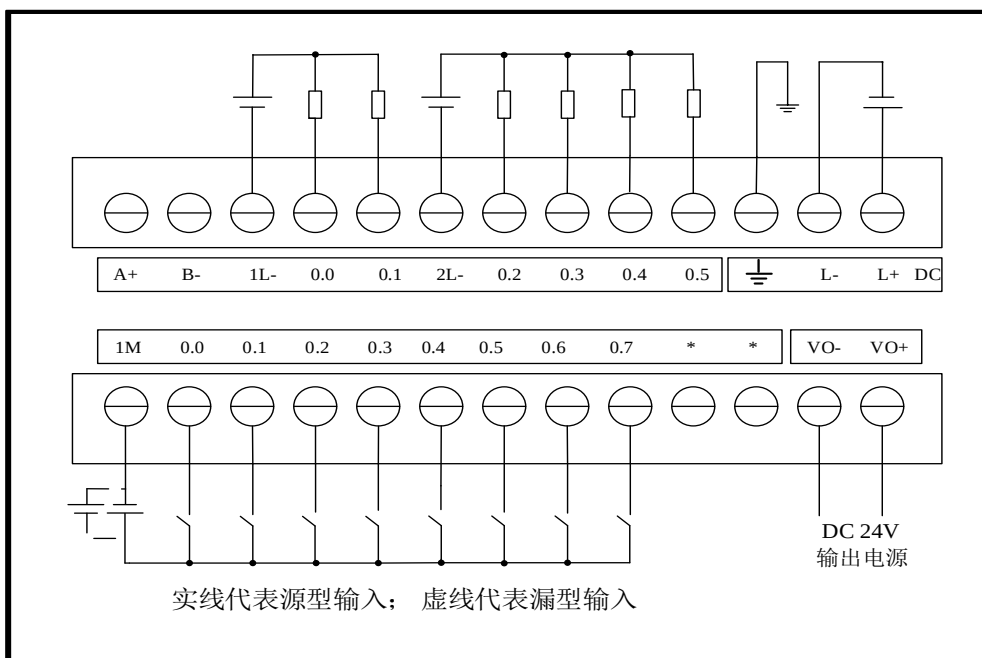
图 3-7 EC202-14DTD 接线图
