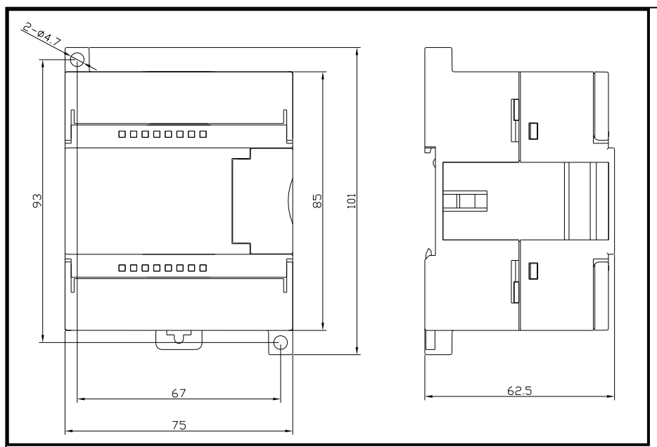
图 4-49 EC253-10DTD 安装尺寸图
