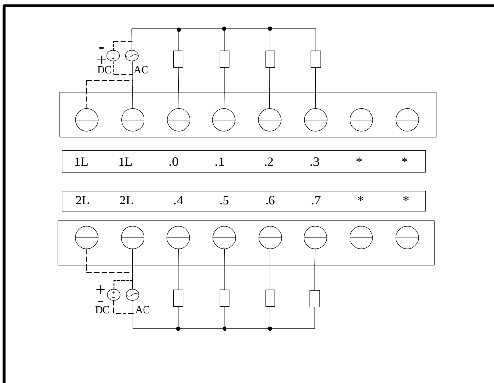
图 4-14 EC222-08XR 接线图
