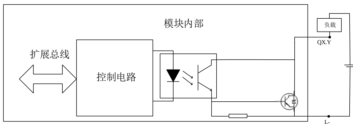
图 4-38 DO 漏型电气原理图
