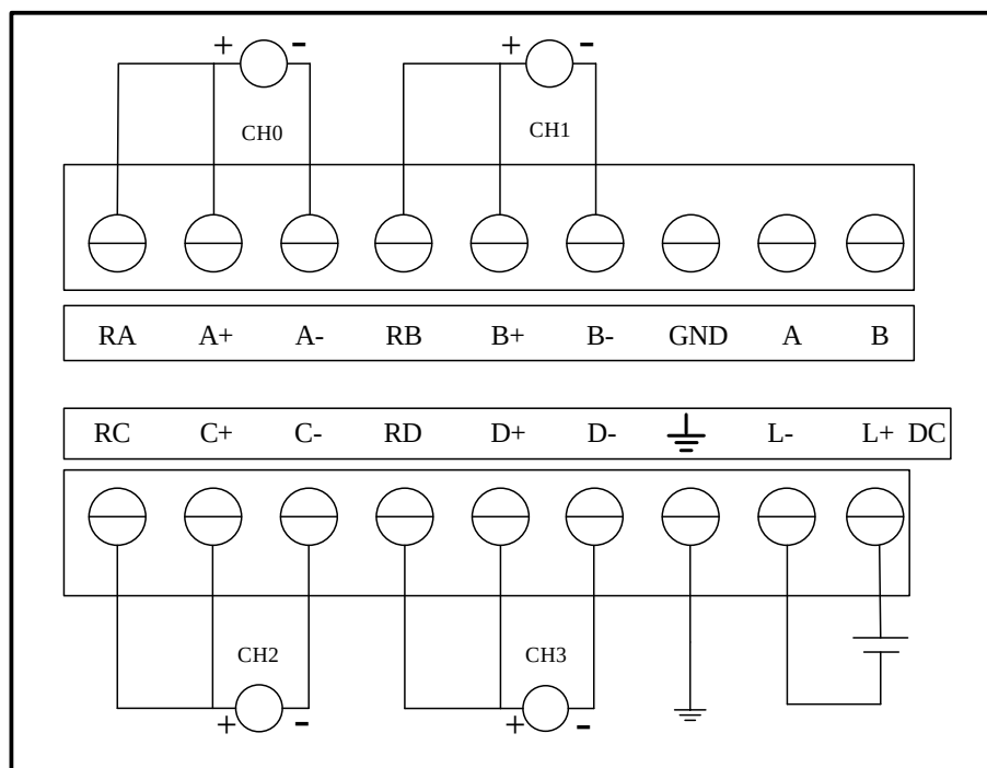
图 5-4 EC231-04IVM 接线图：电流信号（四线制）
