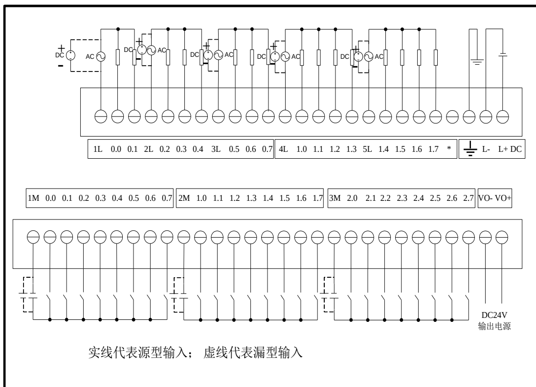
图 3-17 EC206-40DR 接线图
