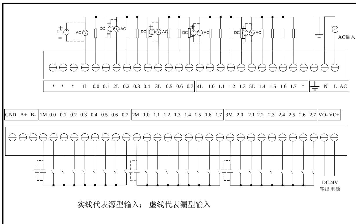
图 3-18 EC206E-40AR 接线图
