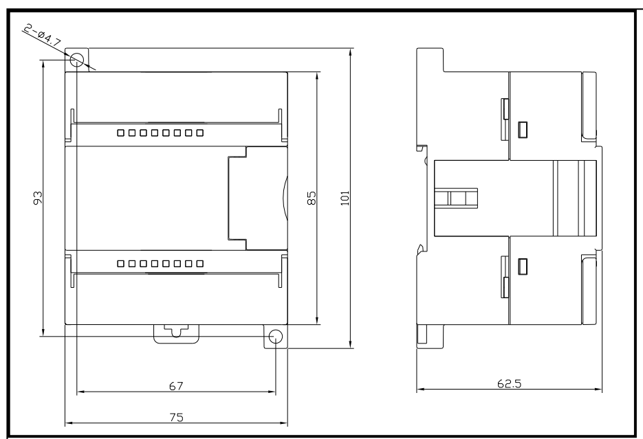
图 4-39 EC223-16DTD 安装尺寸图
