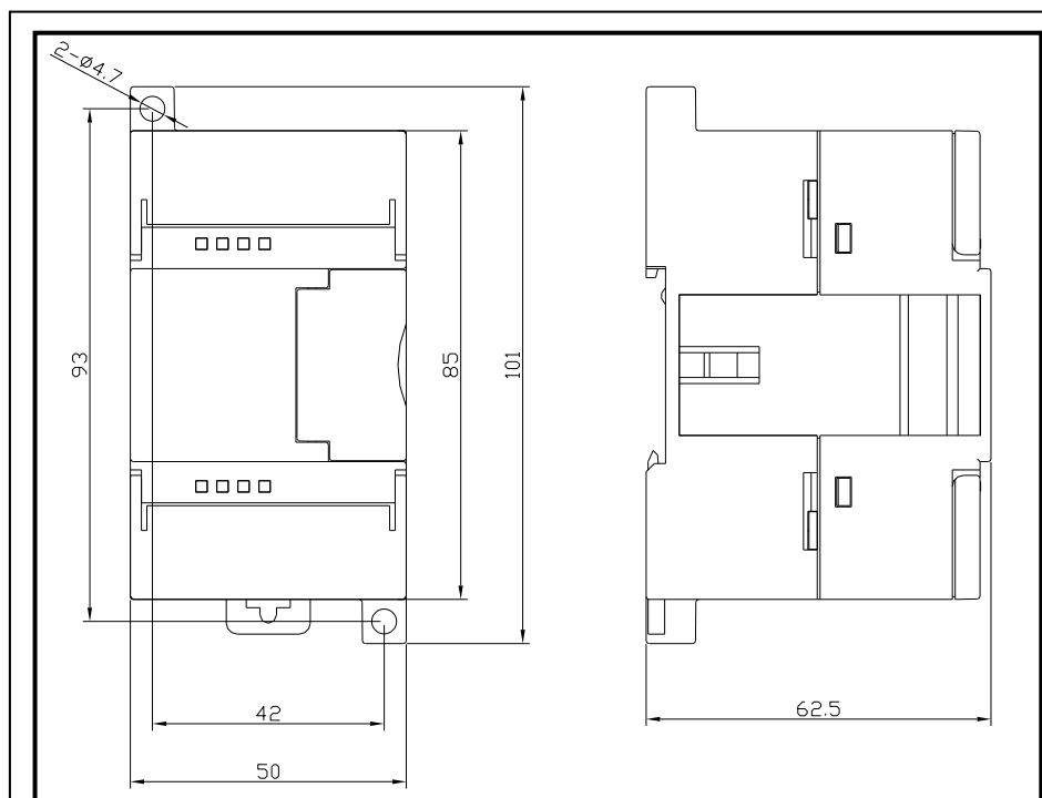
图 4-34 EC223-08DR 安装尺寸图
