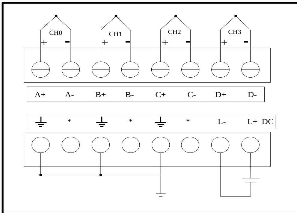
图 5-7 EC231-04RDM 两线制接线图
