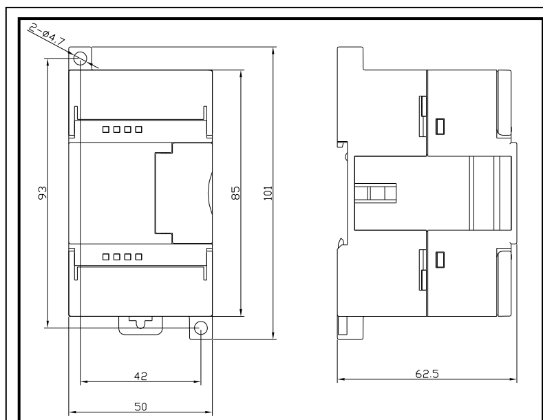
图 4-12 EC222-08DTD 安装尺寸图
