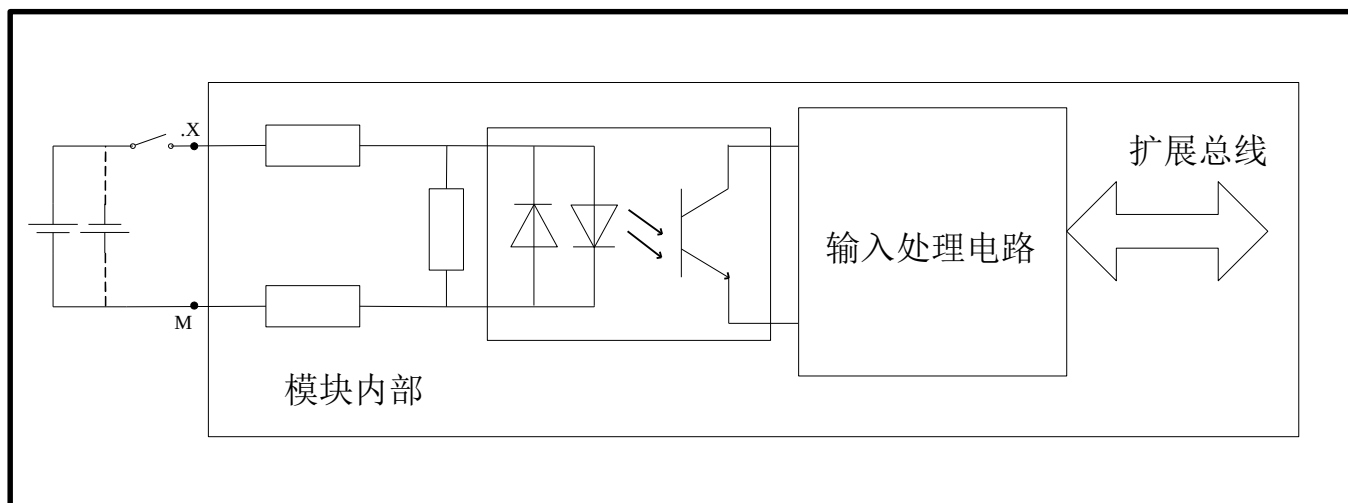
图 4-42 DI 电气原理图
