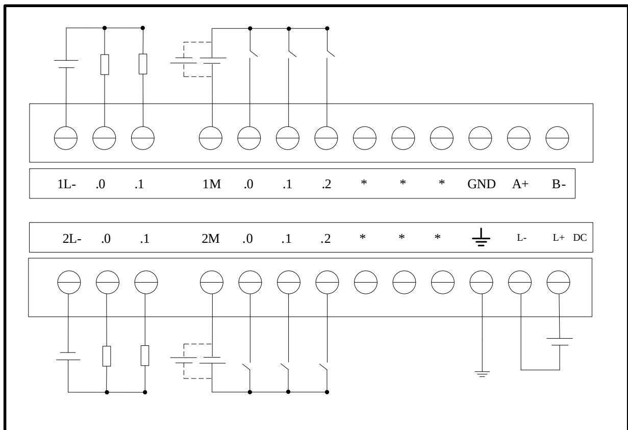
图 4-46 EC253-10DTD 接线图
