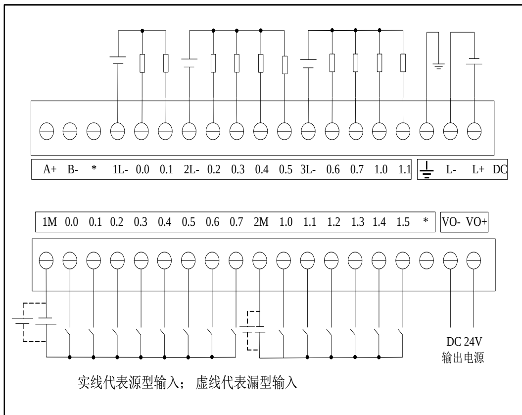
图 3-11 EC204-24DTD 接线图
