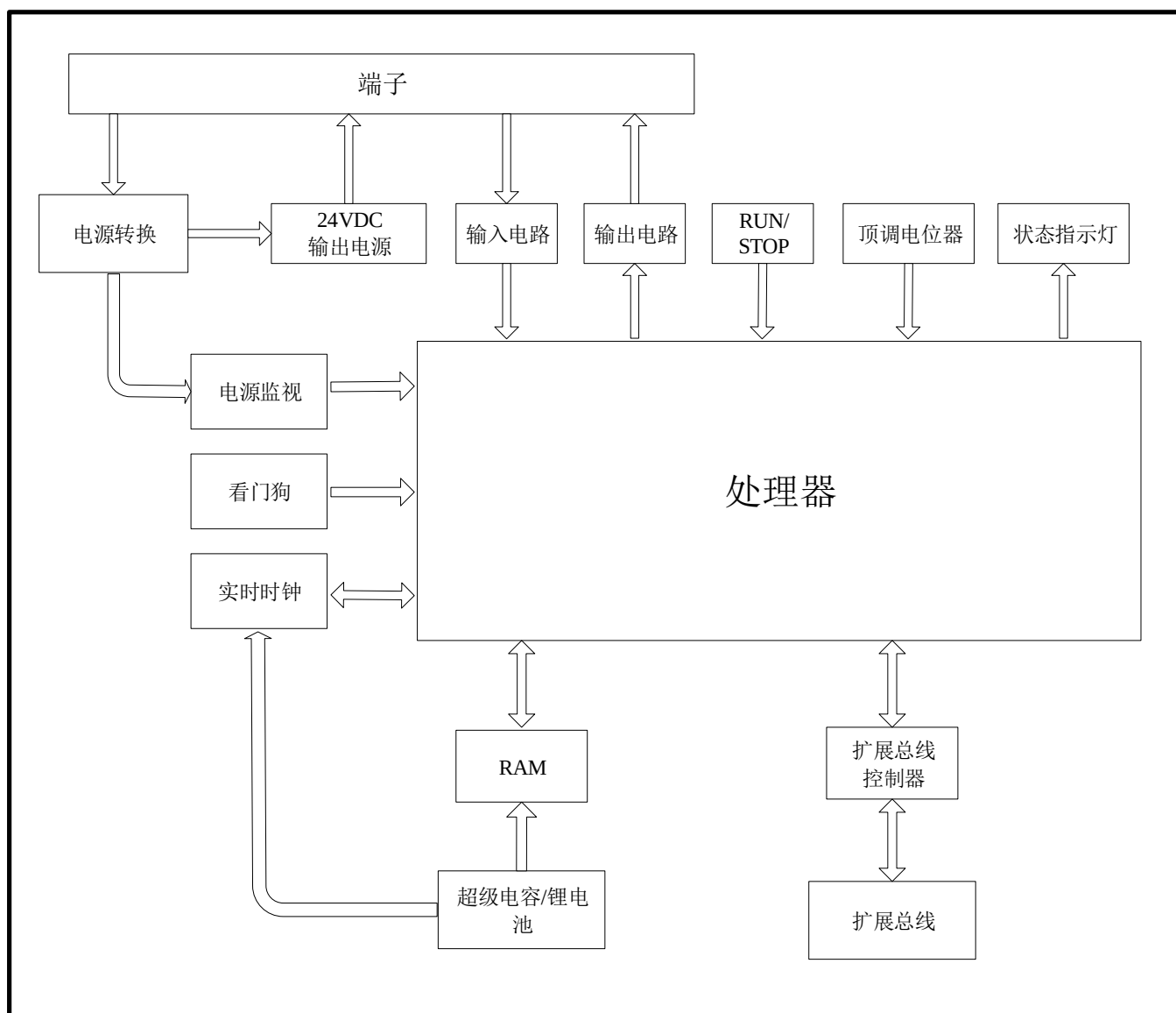
图 3-2 CPU 硬件原理框图
