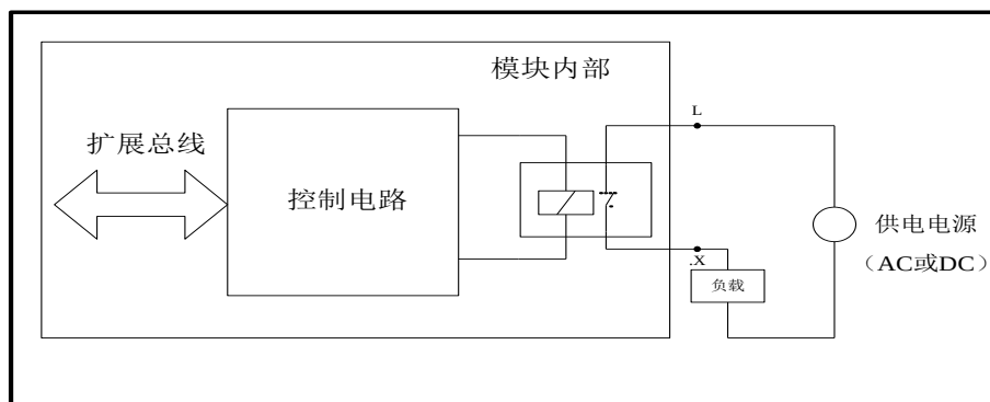
图 4-23 EC222-16XR 电气原理图
