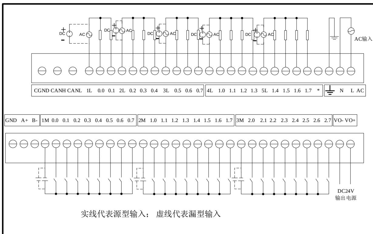
图 3-20 EC206C-40AR 接线图
