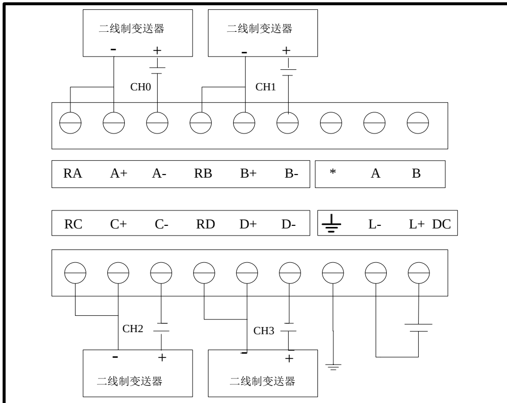
图 5-3 EC231-04IVM 接线图：电流信号（二线制）
