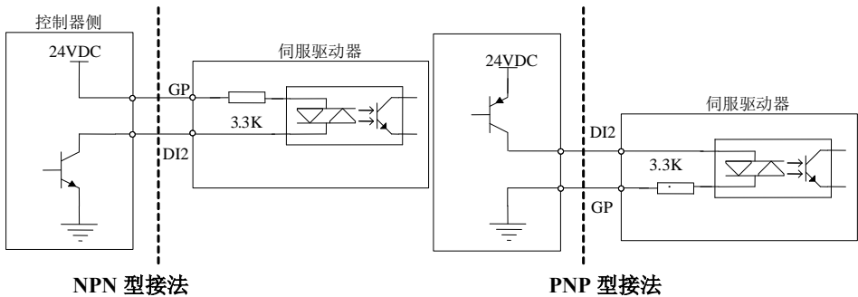
图 4.3.5 有源接点接口电路
