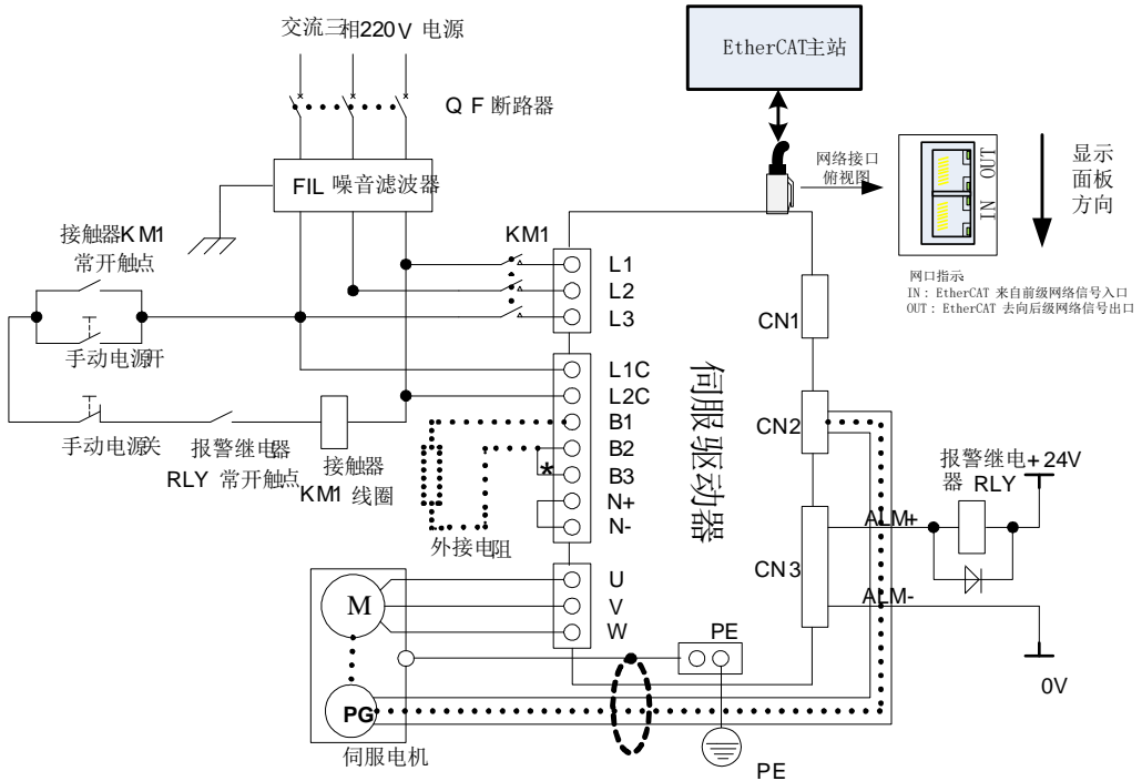
图 4.1.5 220V 驱动器典型主电路配线图
