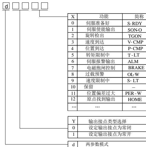
图 8.3.2 可编程输出端子功能设定示意图
