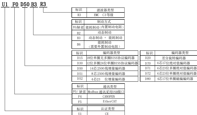
图 2.1.2 伺服驱动器功能部分命名规则
