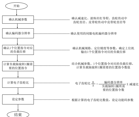
图 7.1.13 电子齿轮比设置步骤流程图
