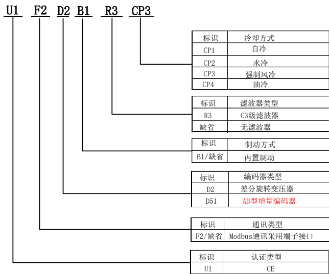
图 1.4.2 伺服驱动器功能部分命名规则
