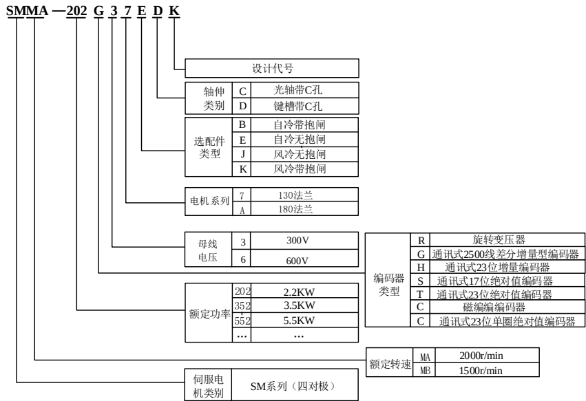
图 1.5.1 伺服电机的命名规则（180 及以下法兰电机）
