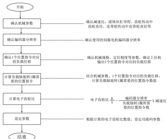
图 7.1.13 电子齿轮比设置步骤流程图
