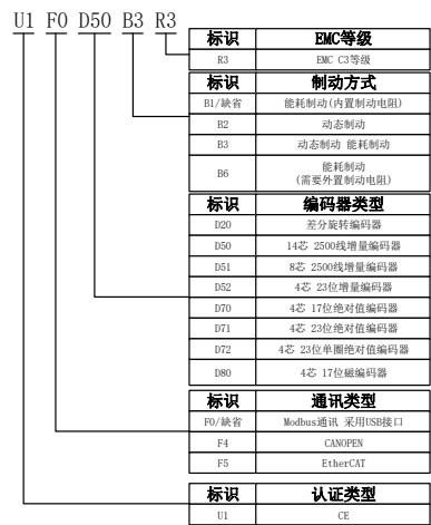
图 2.1.2 伺服驱动器功能部分命名规则
