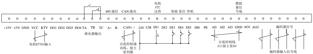
辅泵伺服接线示意图
