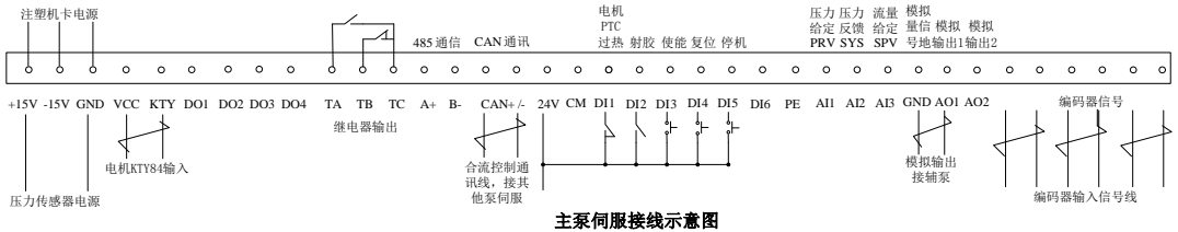
主泵伺服接线示意图
