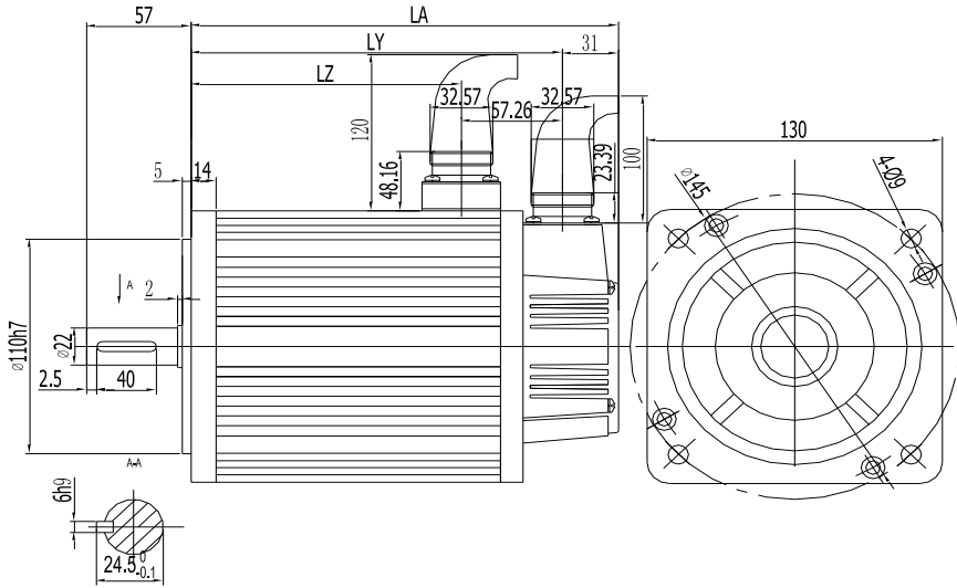
附图1 7(110 止口)机座伺服电机结构尺寸图
